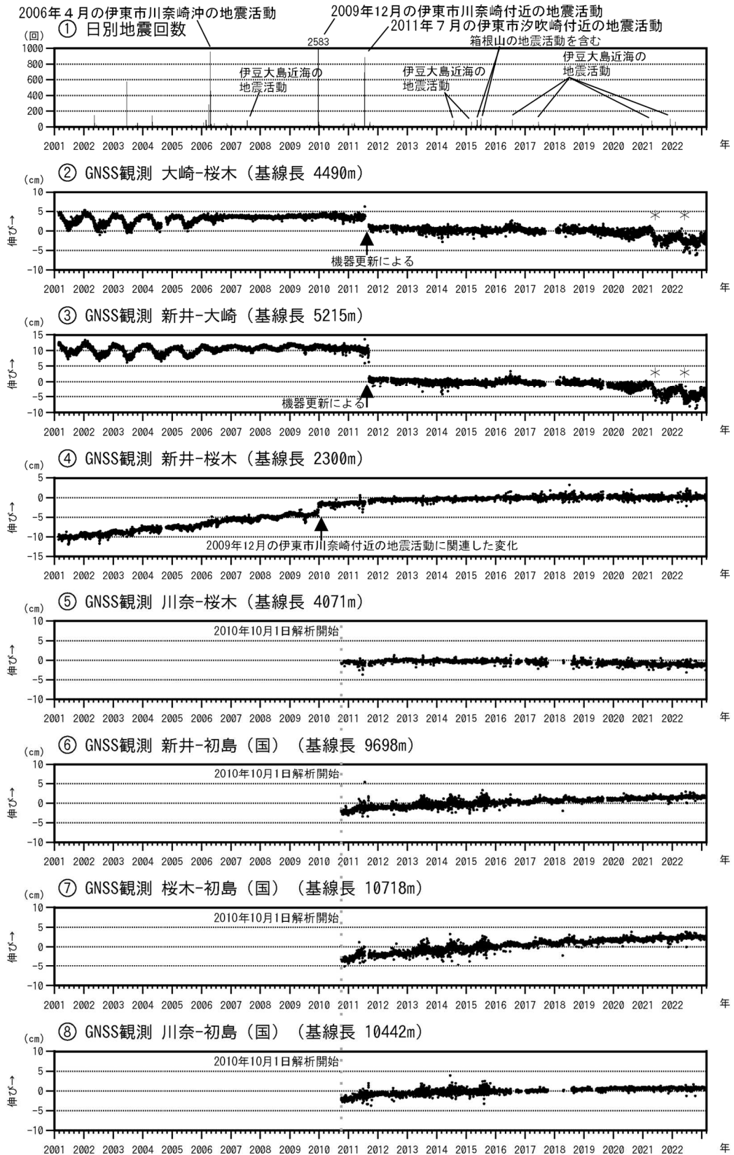
図3 伊豆東部火山群 火山活動経過図（2001年2月1日～2023年2月28日）
