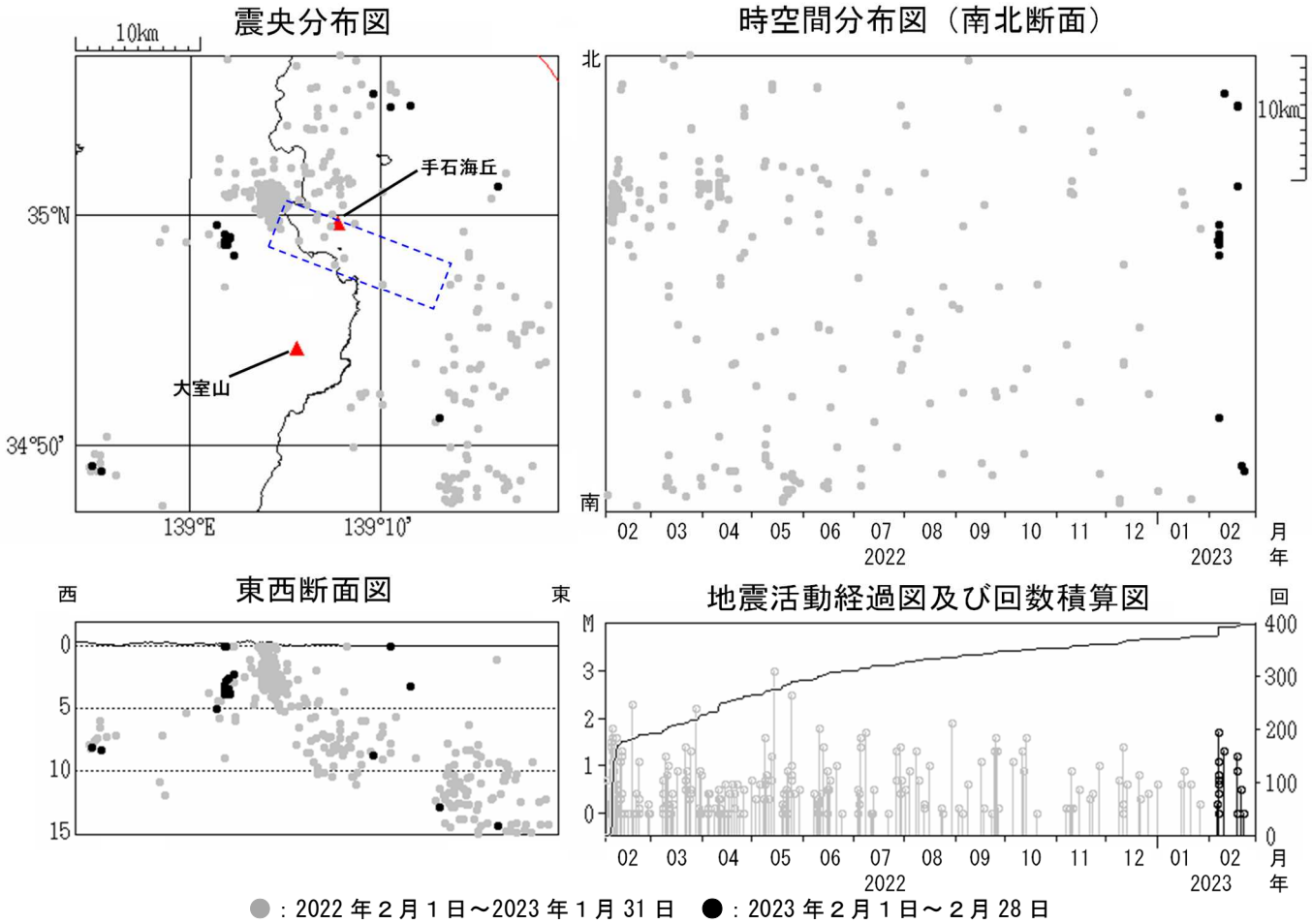
図2 伊豆東部火山群 広域地震観測網による震源分布図（2022年2月1日～2023年2月28日） □の領域は群発地震活動の発生する可能性がある範囲（火口が出現する可能性のある範囲）を示しています。 ( https://www.data.jma.go.jp/vois/data/tokyo/STOCK/level/PDF/level_316.pdf ) 広域地震観測網により震源決定したもので、深さは全て海面以下として決定しています。 M（マグニチュード）は地震の規模を表し、M0.0以上を表示しています。 図中の震源要素は一部暫定値が含まれており、後日変更することがあります。 この図では、関係機関の地震波形を一元的に処理し、地震観測点の標高を考慮する等した手法で得られた震源を用いています。
