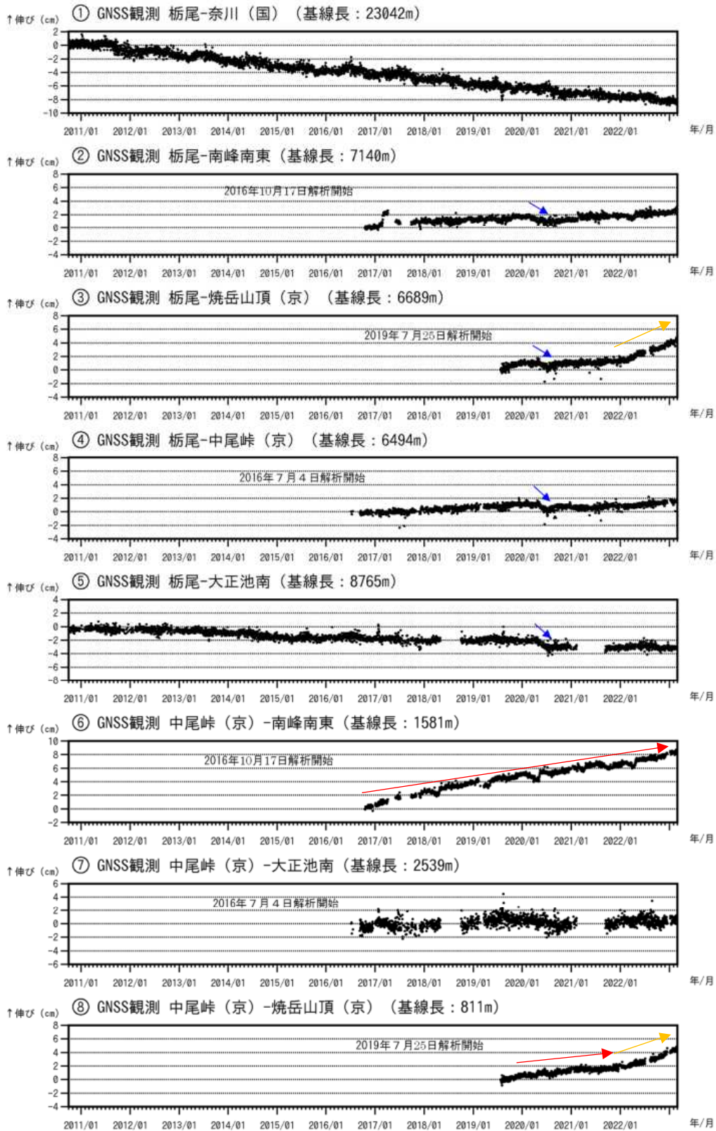
図6 焼岳 GNSS 連続観測による基線長変化（2010年10月1日～2023年2月28日） 図7のGNSS基線①～⑧に対応しています。グラフの空白部分は欠測を示します。（国）は国土地理院、（京）は京都大学の観測点です。
