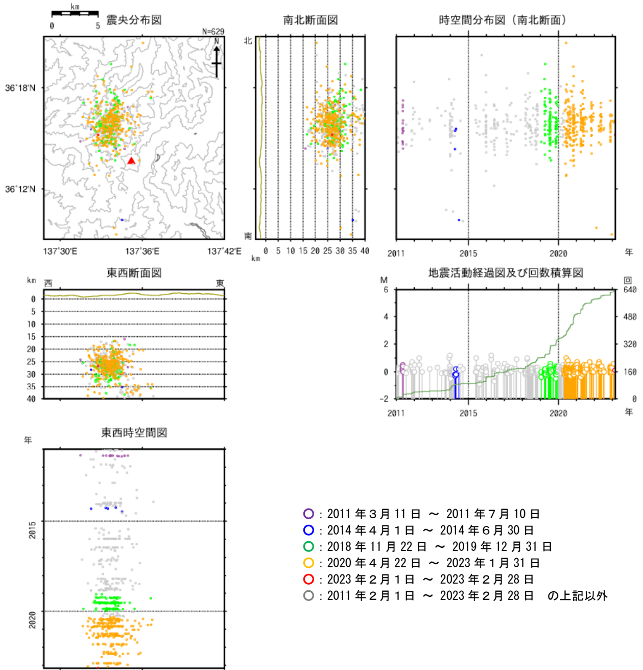
図10 焼岳 広域地震観測網による深部低周波地震の震源分布図（2011年1月1日～2023年2月28日） 広域地震観測網により震源決定したもので、深さは全て海面以下として決定しています。そのため、山頂付近の浅い地震の震源も海面下に決定されています。 M（マグニチュード）は地震の規模を表します。 図中の震源要素は一部暫定値が含まれており、後日変更することがあります。
