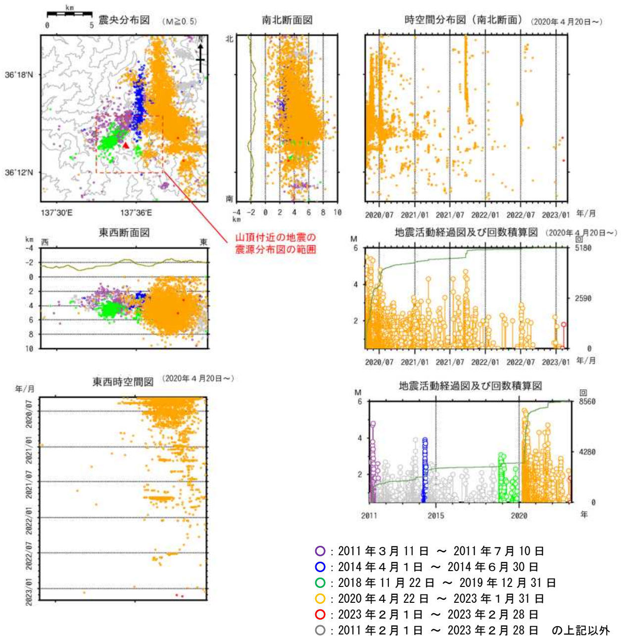
図9 焼岳 広域地震観測網による山体及び周辺の地震活動(2011年1月1日～2023年2月28日) 広域地震観測網により震源決定したもので、深さは全て海面以下として決定しています。そのため、山頂付近の浅い地震の震源も海面下に決定されています。 M(マグニチュード)は地震の規模を表します。 図中の震源要素は一部暫定値が含まれており、後日変更することがあります。 地震活動経過図及び回数積算図の緑色線は積算回数を示し、右軸で表されます。 震央分布図中の赤破線領域が、図2で示す領域に対応しています。
