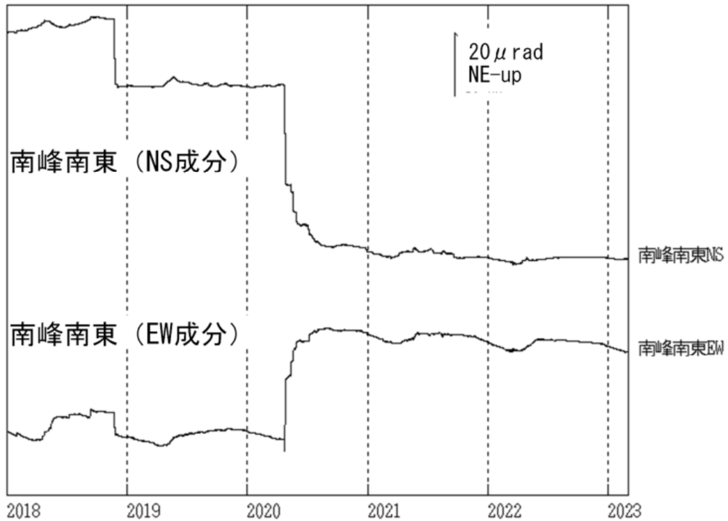
図8 焼岳 南峰南東観測点における傾斜データ（2018年1月1日～2023年2月28日）
