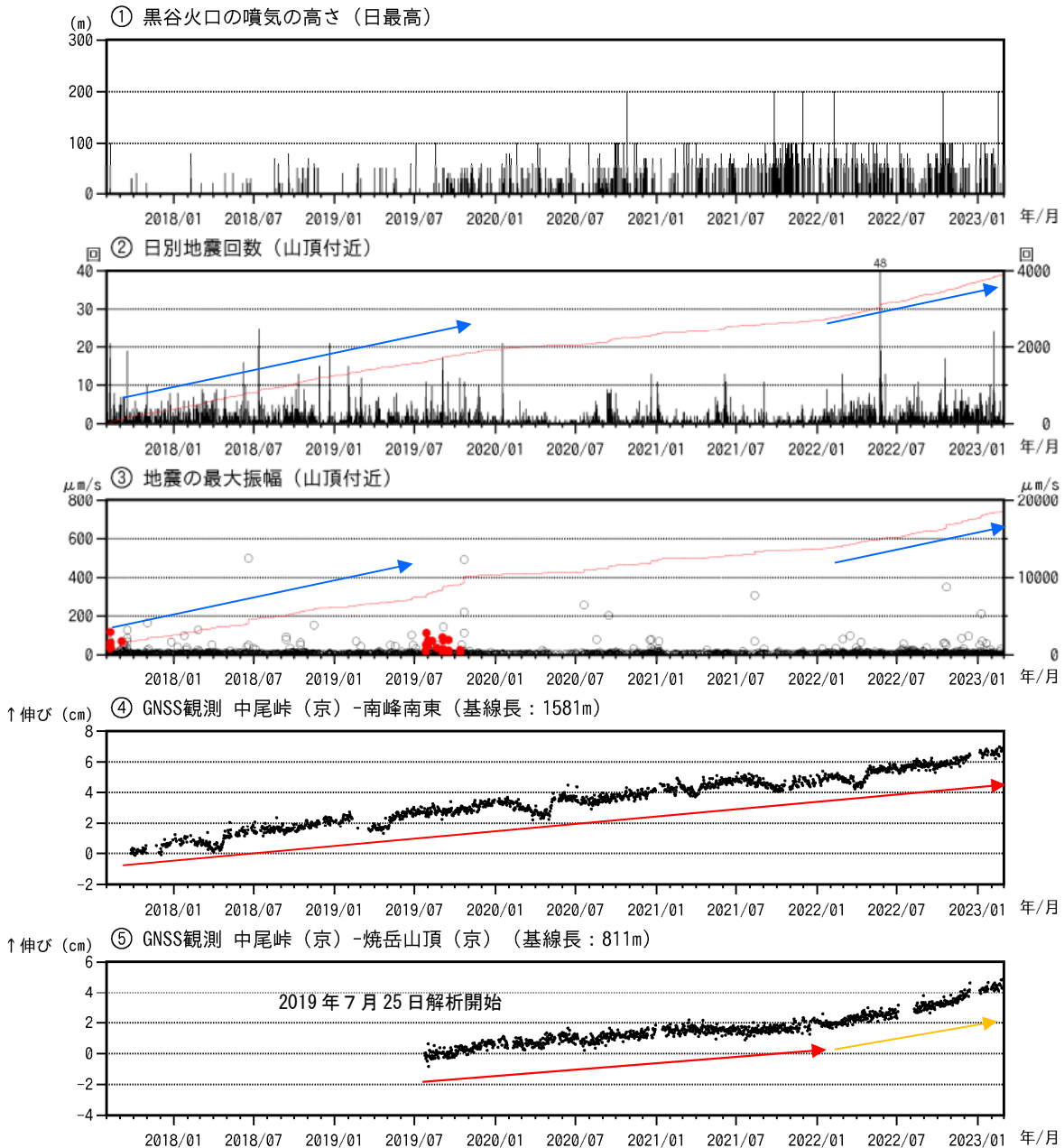
図1 焼岳 火山活動経過図（2017年8月1日～2023年2月28日）
