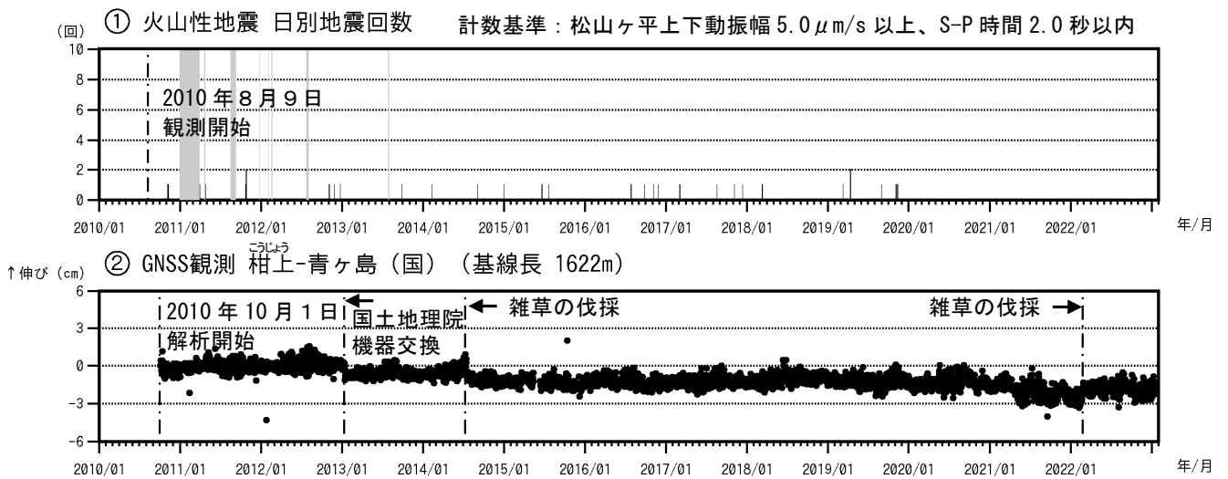
図3 青ヶ島 火山活動経過図（2010年8月9日～2023年1月31日）
