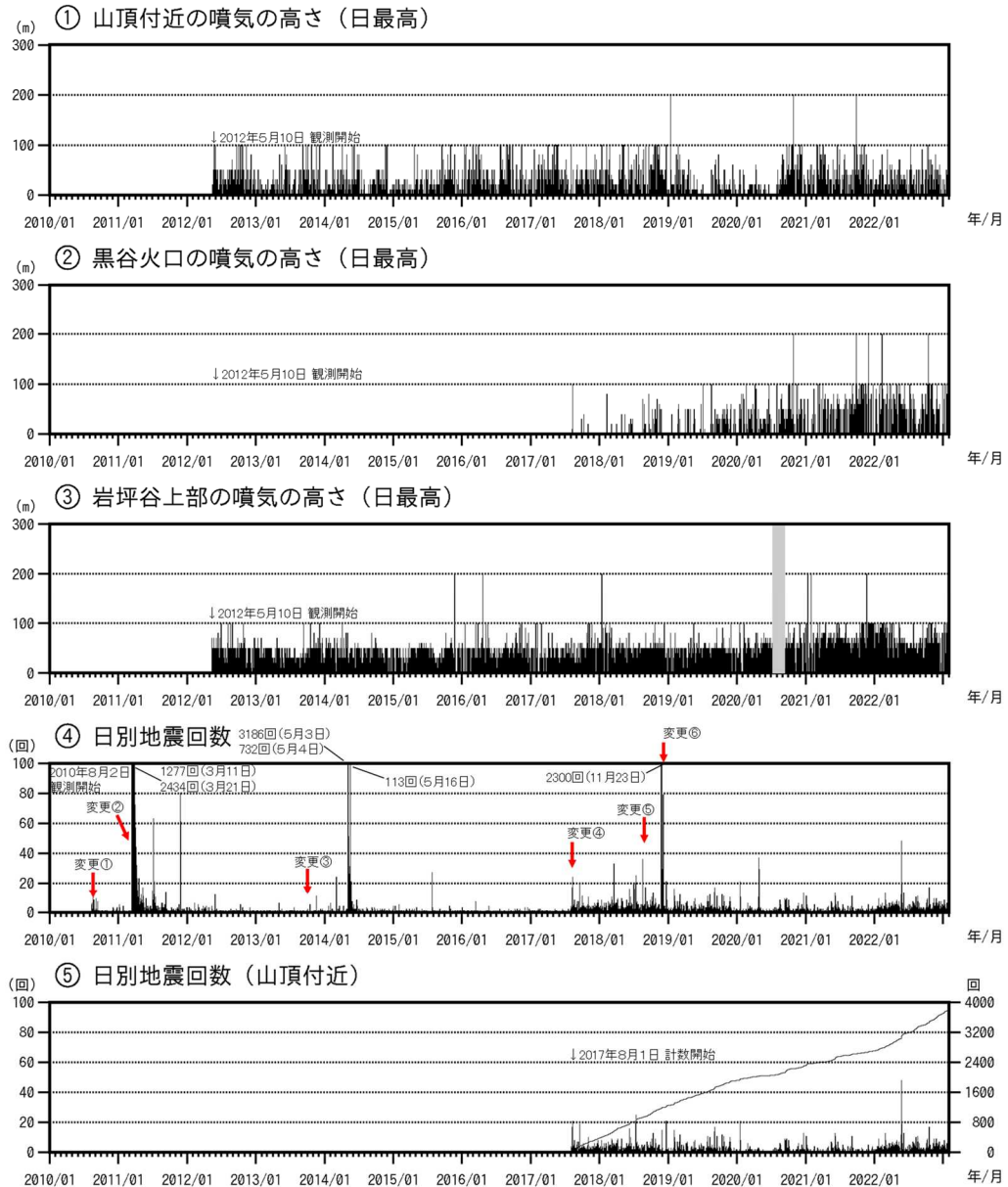
図5 焼岳 噴気の高さと地震回数の推移(2010年8月2日～2023年1月31日)
