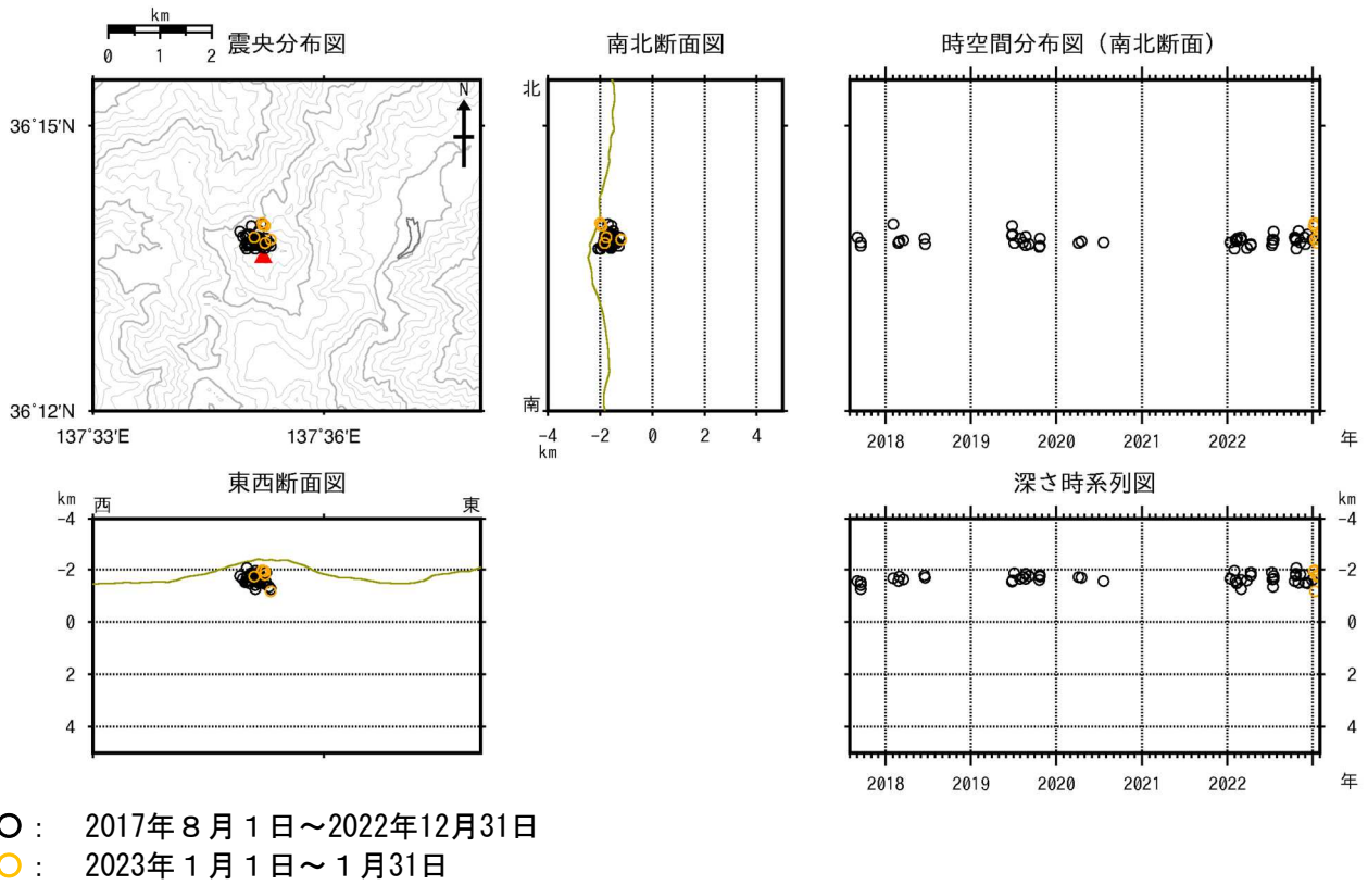
図2 焼岳 山頂付近の地震の震源分布図（2017年8月1日～2023年1月31日）
