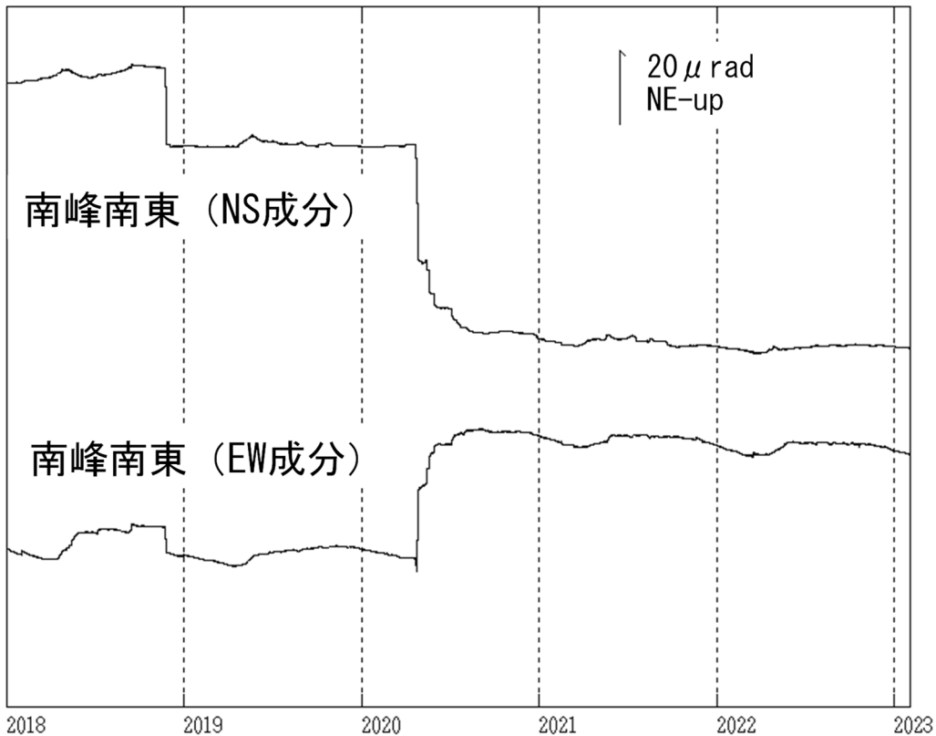
図8 焼岳 南峰南東観測点における傾斜データ（2018年1月1日～2023年1月31日）
