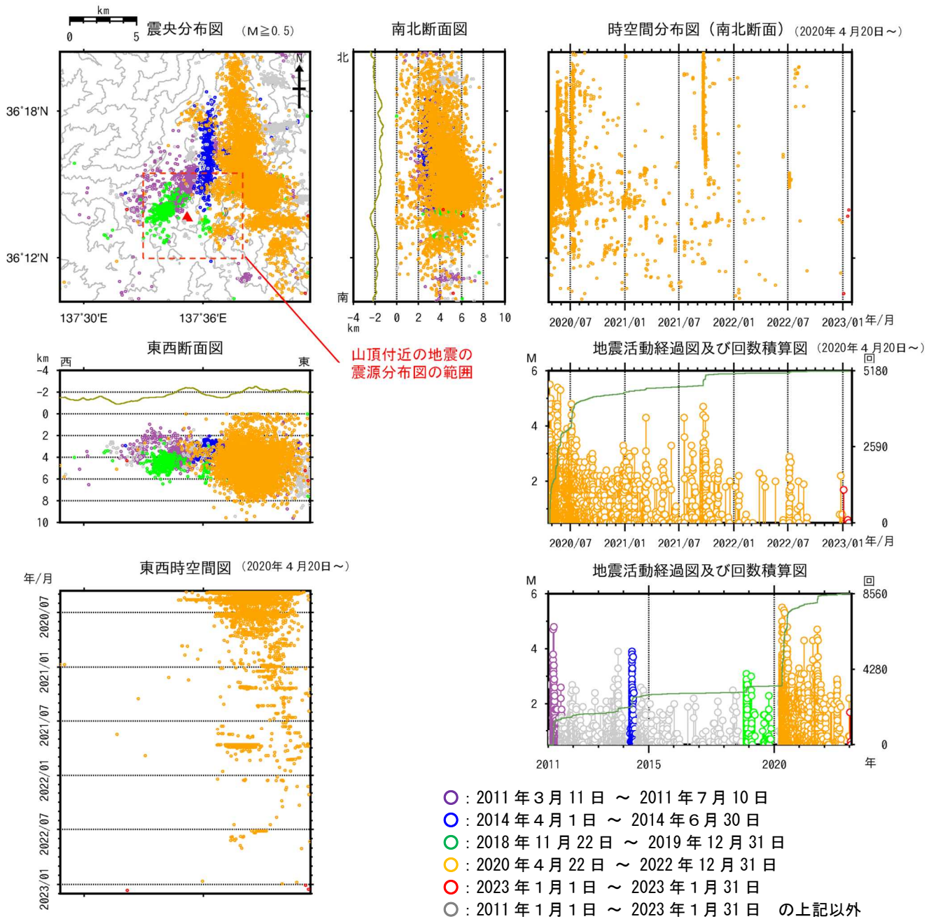
図9 焼岳 広域地震観測網による山体及び周辺の地震活動(2011年1月1日～2023年1月31日) 広域地震観測網により震源決定したもので、深さは全て海面以下として決定しています。そのため、山頂付近の浅い地震の震源も海面下に決定されています。 M (マグニチュード) は地震の規模を表します。 図中の震源要素は一部暫定値が含まれており、後日変更することがあります。 地震活動経過図及び回数積算図の緑色線は積算回数を示し、右軸で表されます。 震央分布図中の赤破線領域が、図2で示す領域に対応しています。
