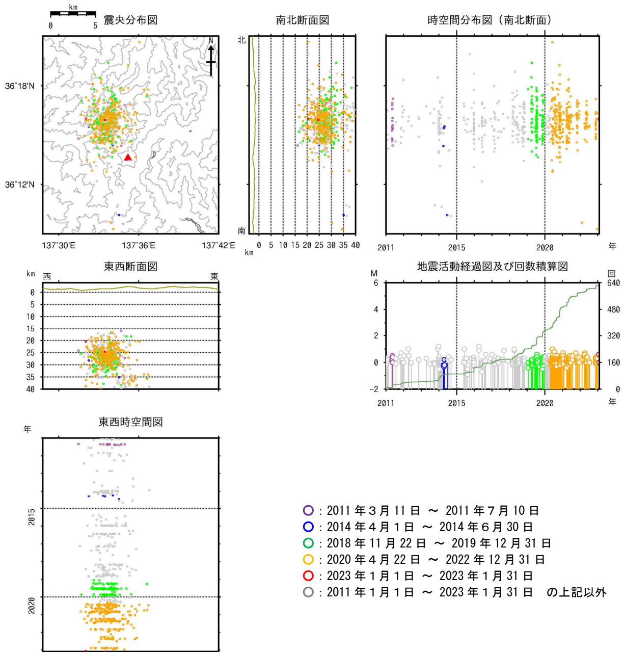
図10 焼岳 広域地震観測網による深部低周波地震の震源分布図（2011年1月1日～2023年1月31日） 広域地震観測網により震源決定したもので、深さは全て海面以下として決定しています。そのため、山頂付近の浅い地震の震源も海面下に決定されています。 M（マグニチュード）は地震の規模を表します。 図中の震源要素は一部暫定値が含まれており、後日変更することがあります。
