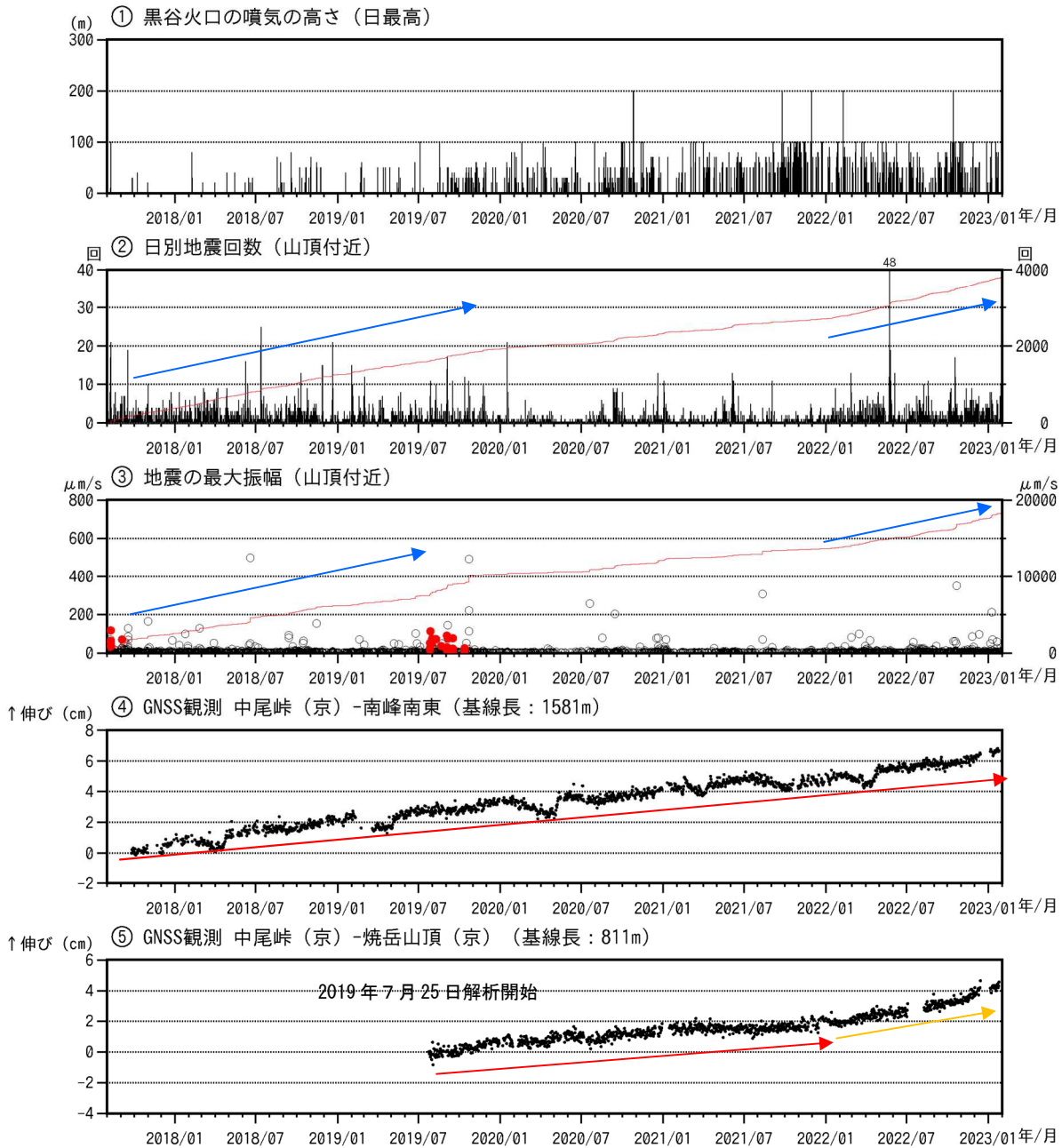
図1 焼岳 火山活動経過図（2017年8月1日～2023年1月31日）
