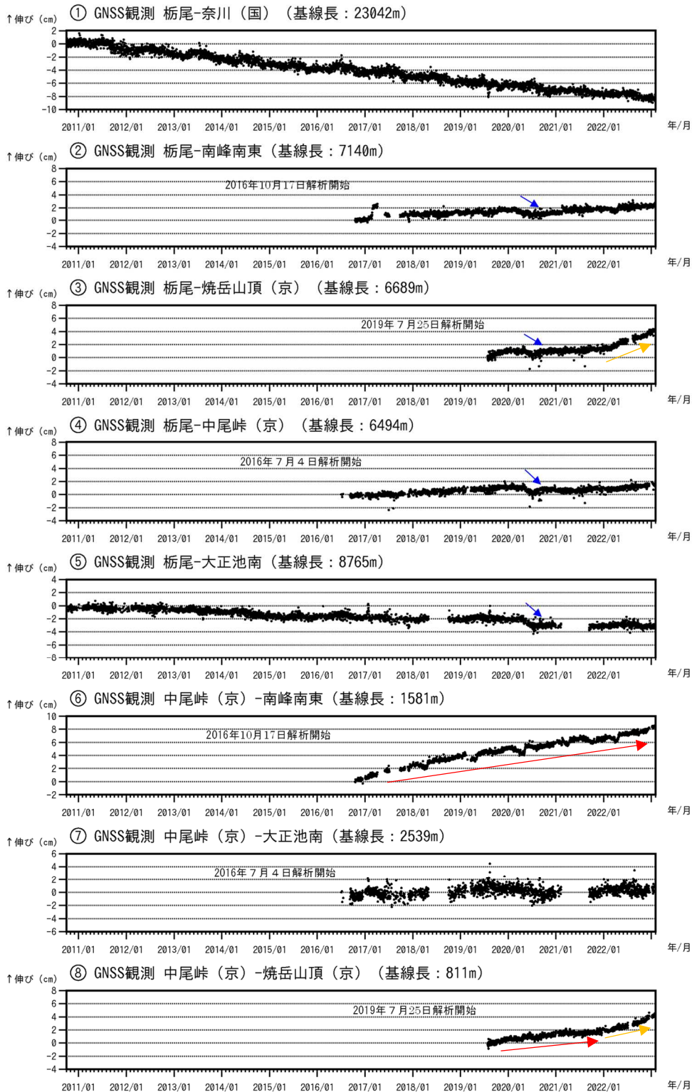
図6 焼岳 GNSS 連続観測による基線長変化（2010年10月1日～2023年1月31日）
