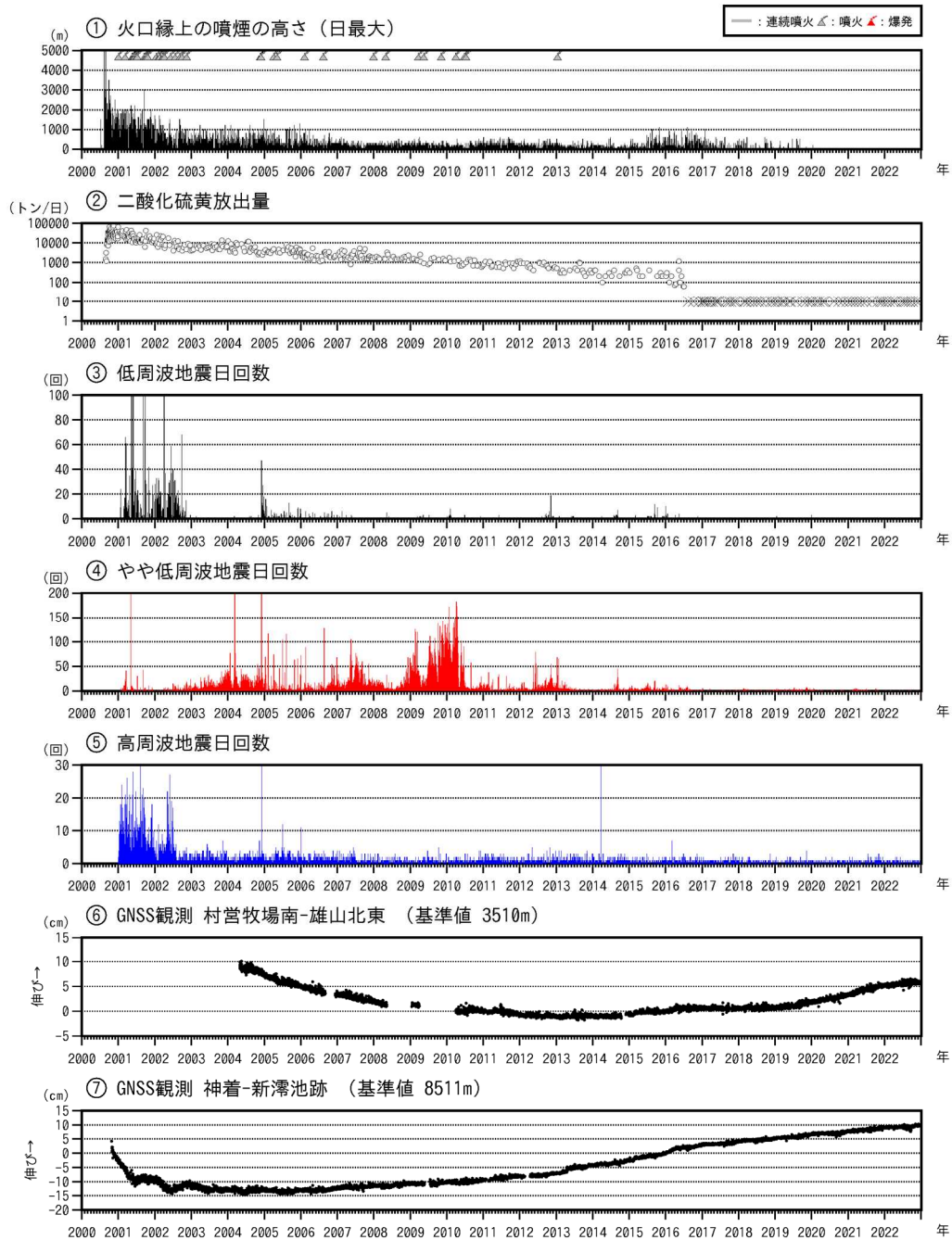
図7 三宅島 長期の火山活動経過図（2000年1月1日～2022年12月31日）
