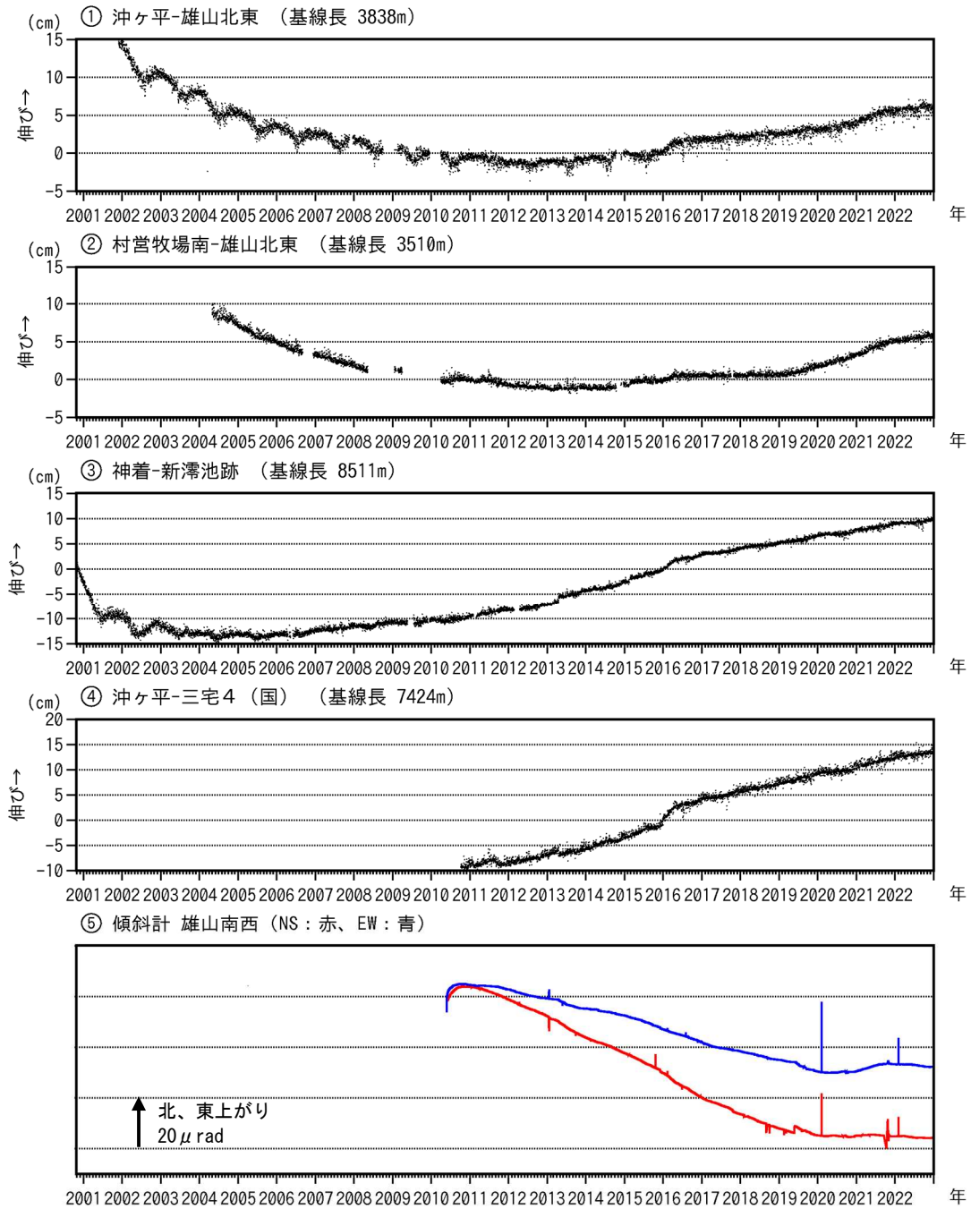
図8 三宅島 GNSS 連続観測及び傾斜計観測結果（2000年10月26日～2022年12月31日）
