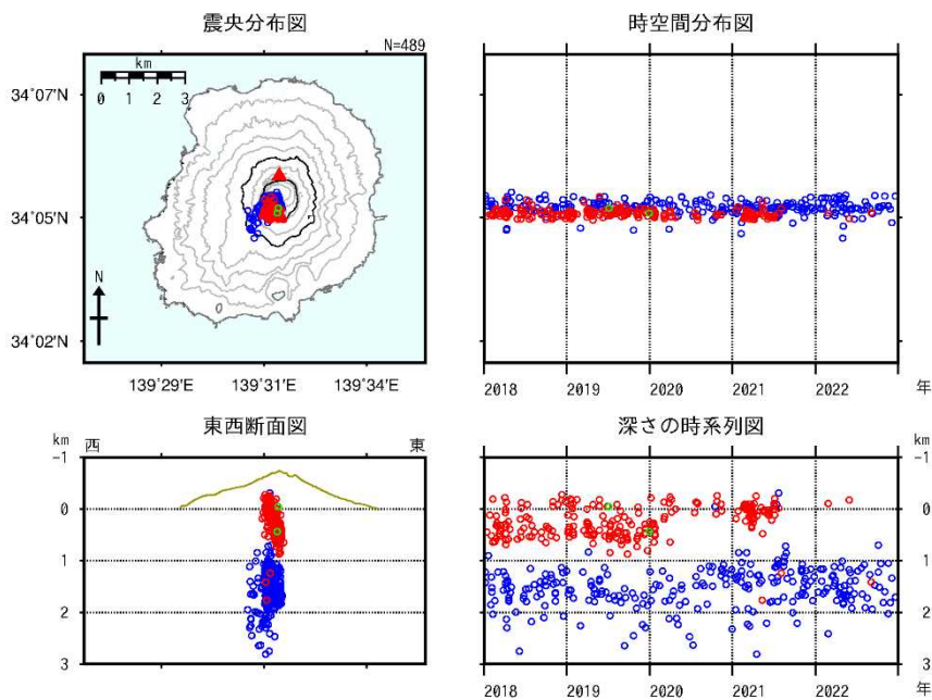
図9 三宅島 震源分布図
