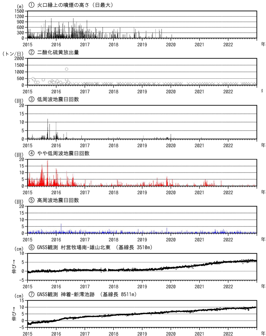
図6 三宅島 火山活動経過図（2015年1月1日～2022年12月31日）
