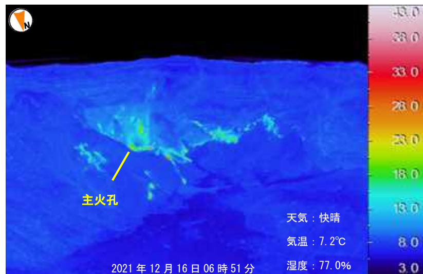
図5 三宅島 山頂火口内の地熱域の状況（スオウ穴から撮影）
