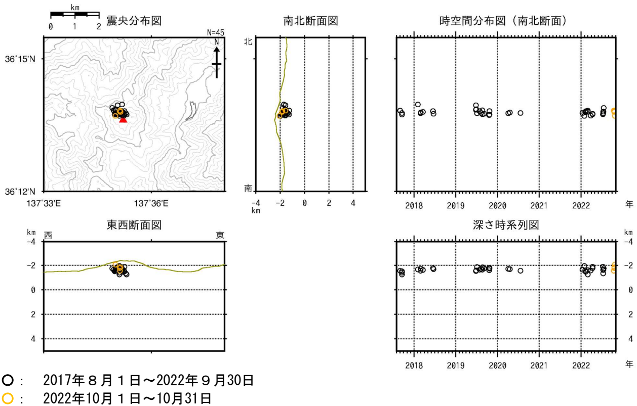
図2 焼岳 山頂付近の地震の震源分布図（2017年8月1日～2022年10月31日）
