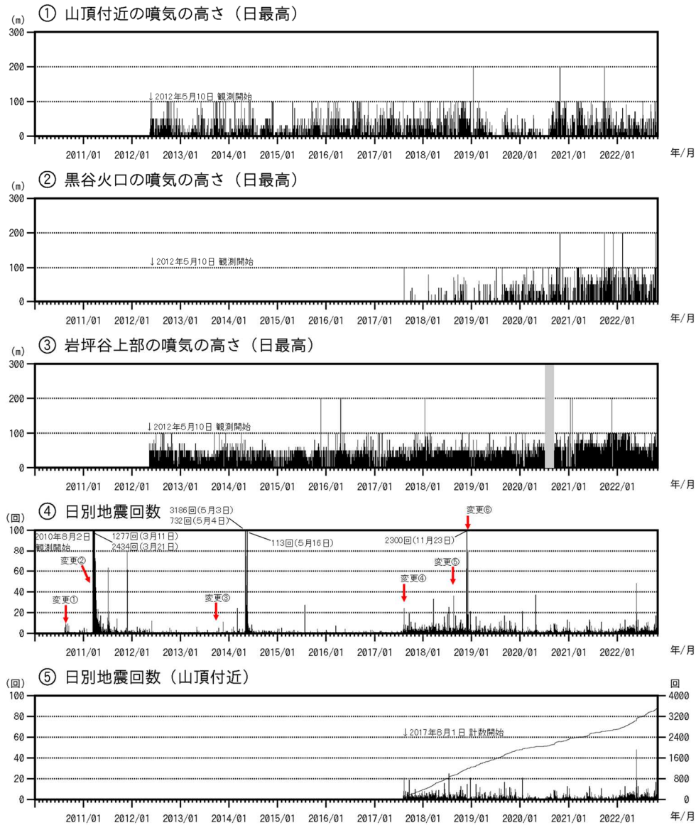
図5 焼岳 噴気の高さと地震回数の推移(2010年8月2日～2022年10月31日)
