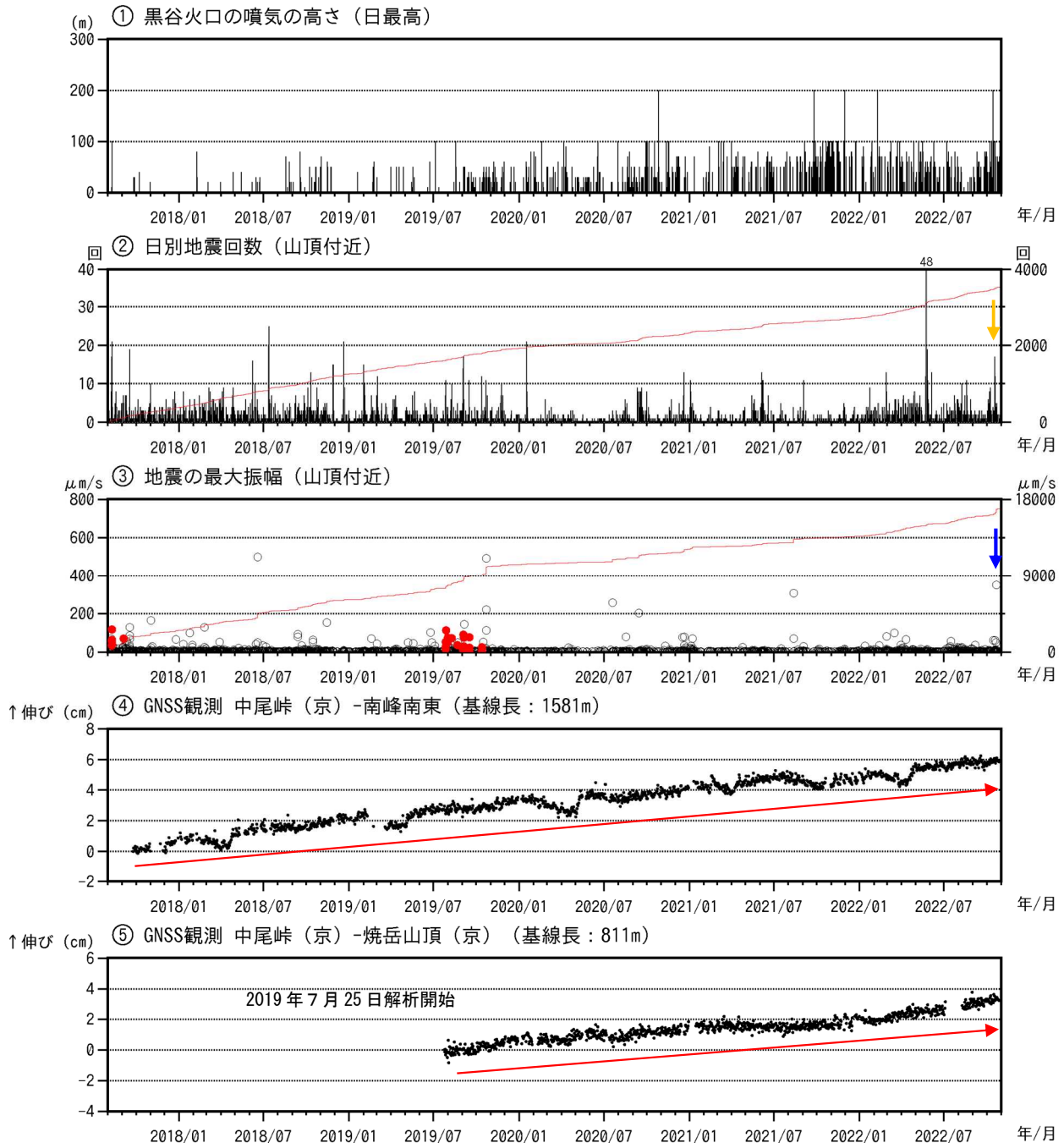
図1 焼岳 火山活動経過図（2017年8月1日～2022年10月31日）
