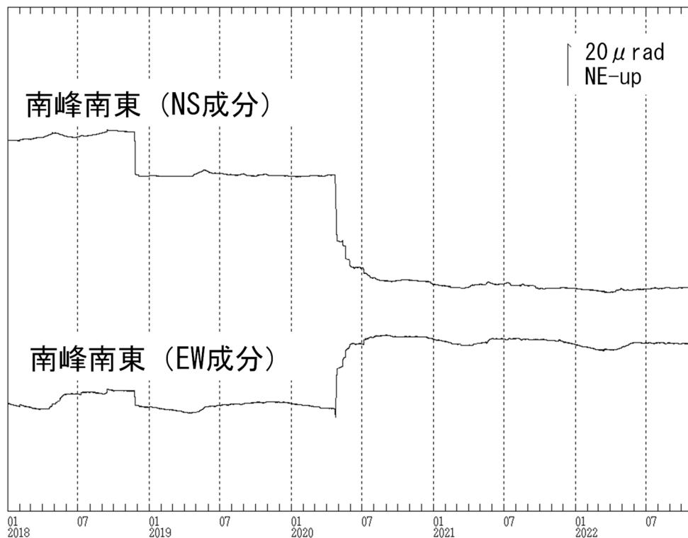
図8 焼岳 南峰南東観測点における傾斜データ（2018年1月1日～2022年10月31日）
