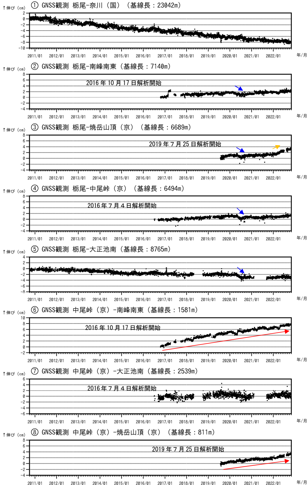
図6 焼岳 GNSS連続観測による基線長変化（2010年10月1日～2022年10月31日） 図7のGNSS基線①～⑧に対応しています。グラフの空白部分は欠測を示します。（国）は国土地理院、（京）は京都大学の観測点です。
