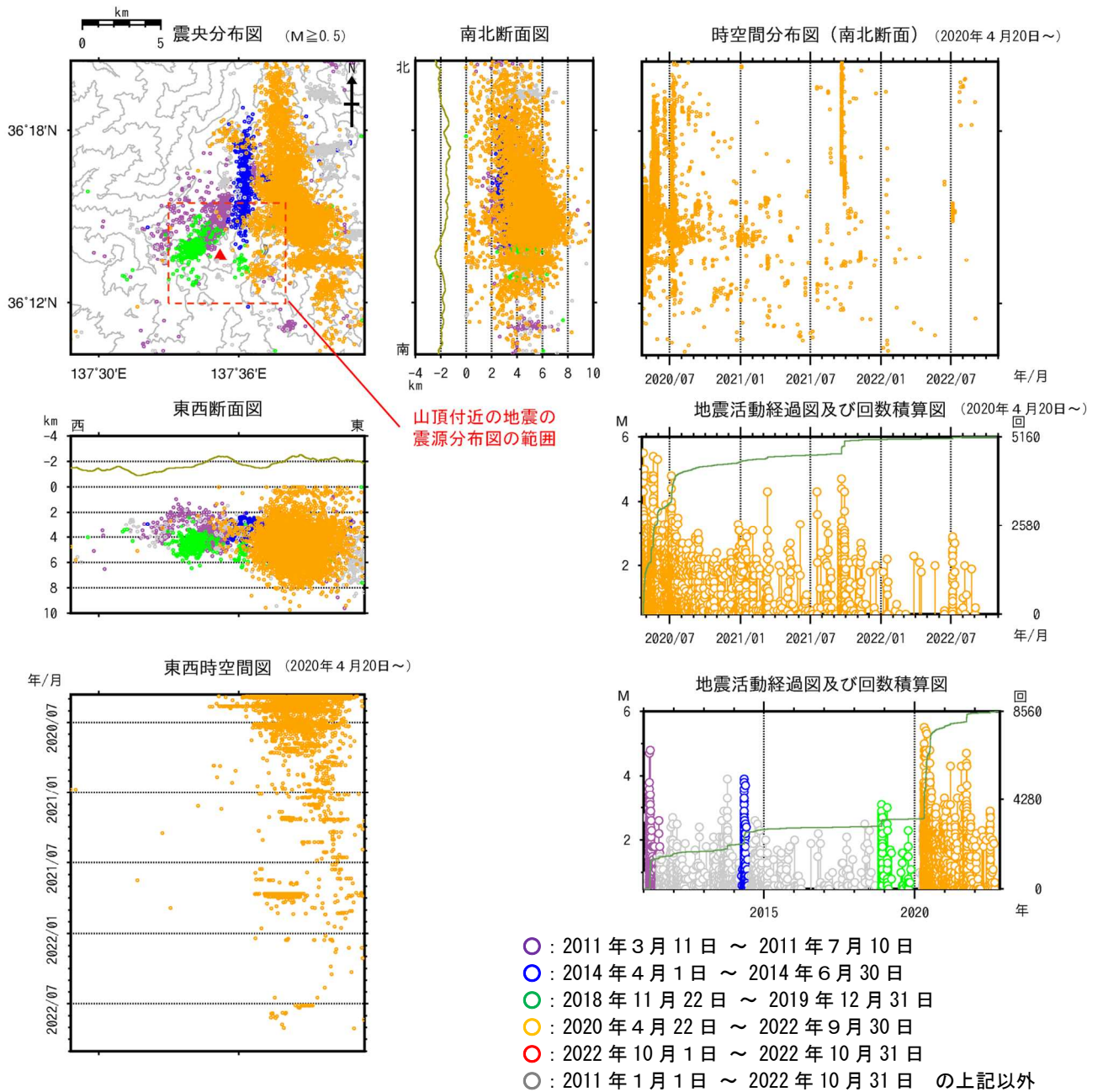
図9 焼岳 広域地震観測網による山体及び周辺の地震活動(2011年1月1日～2022年10月31日) 広域地震観測網により震源決定したもので、深さは全て海面以下として決定しています。そのため、山頂付近の浅い地震の震源も海面下に決定されています。 M (マグニチュード) は地震の規模を表します。 図中の震源要素は一部暫定値が含まれており、後日変更することがあります。 地震活動経過図及び回数積算図の緑色線は積算回数を示し、右軸で表されます。 震央分布図中の赤破線領域が、図2で示す領域に対応しています。
