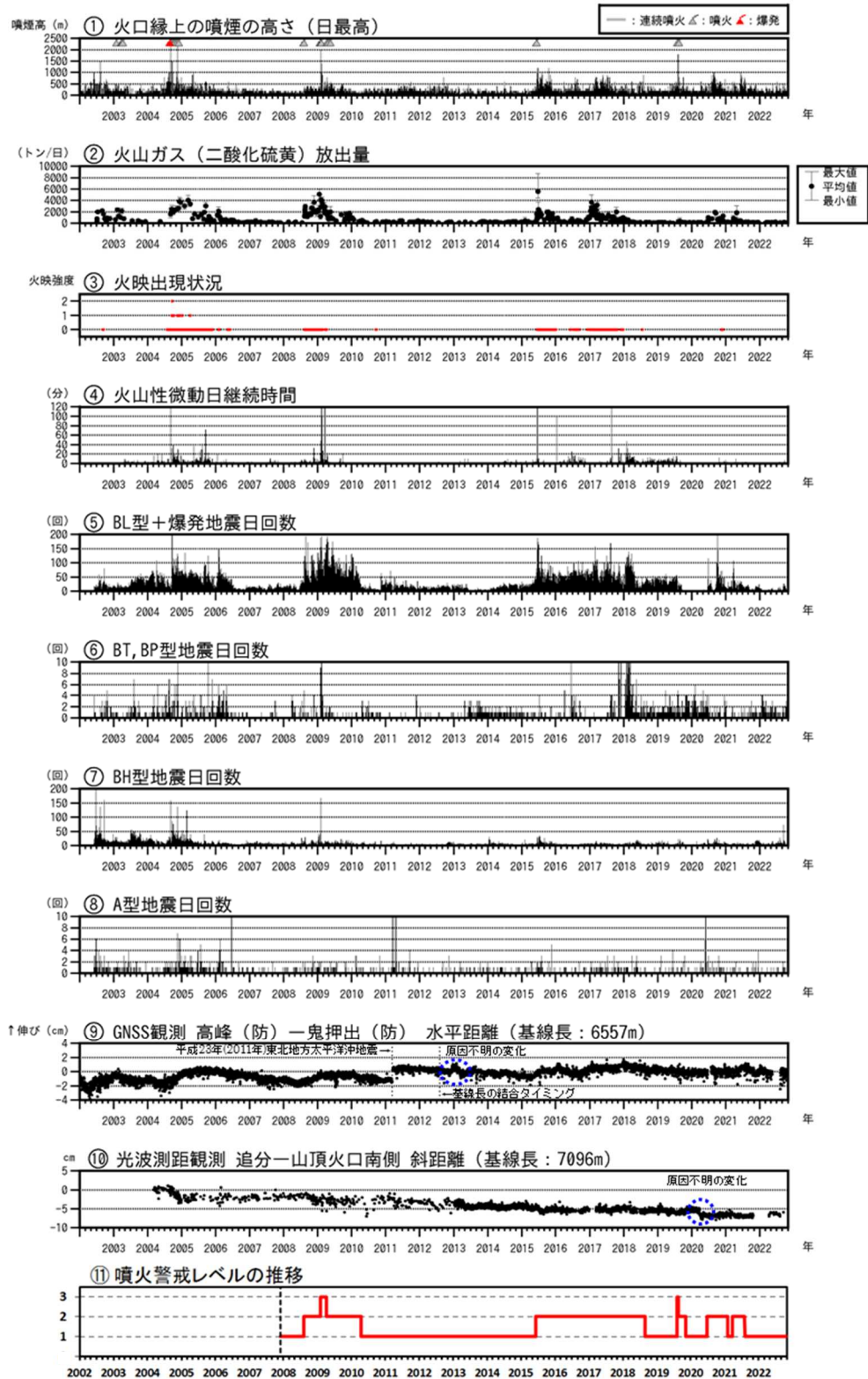
図4 浅間山 火山活動経過図（2002年1月1日～2022年10月31日）
