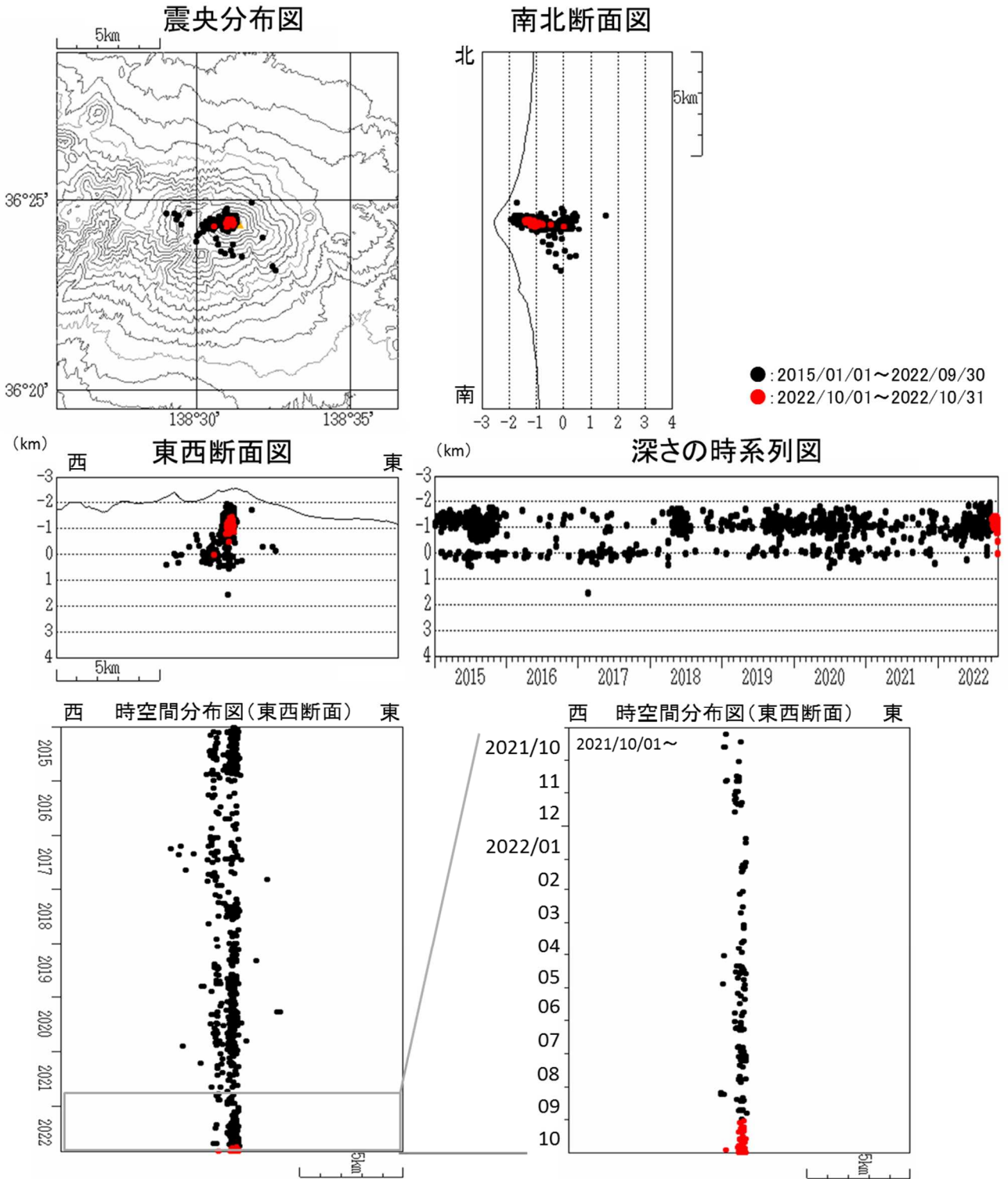
図5 浅間山 震源分布図（2015年1月1日～2022年10月31日）
