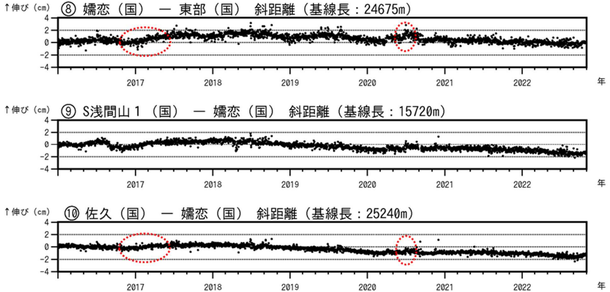
図6-2 浅間山 GNSS 連続観測結果(2016年1月1日~2022年10月31日) ⑧⑨⑩は図7の⑧⑨⑩にそれぞれ対応しています。空白部分は欠測を示します。(国)：国土地理院。 ・GNSS 連続観測では、特段の変化は認められません。 ・過去には、浅間山の西側を挟む基線などでわずかな伸びの変化がみられました(⑧⑩の基線の赤破線の期間)。これらは深部からのマグマ上昇を示す地殻変動と考えられています。
