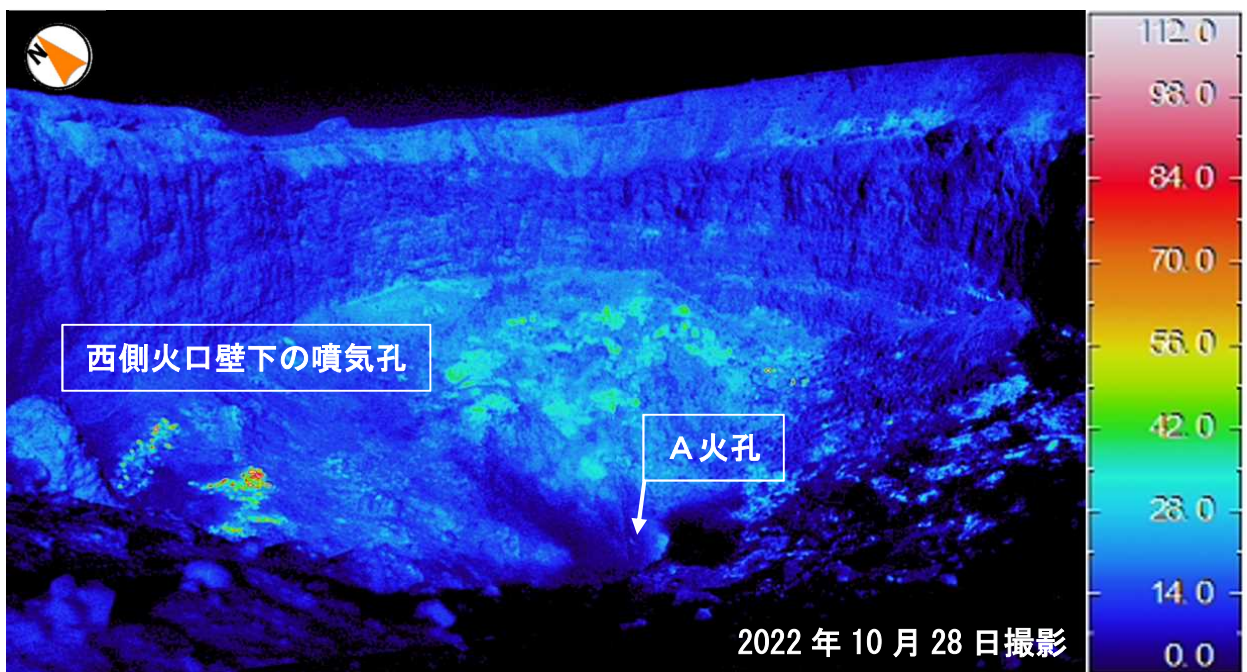
図9 浅間山 火口南西縁からみた山頂火口内の状況（2022年10月28日及び2021年10月15日） ・ 山頂火口底中央部にあるA火孔から白色の噴煙が、西側火口壁下の噴気孔から白色及び青白色の噴煙が上がっていました。 ・ 西側火口壁下では、広範囲に噴気と黄色の硫黄昇華物の付着がみられました。 ・ 赤外熱映像装置による観測では、昨年（2021年10月）の現地調査結果と比べて、火口内の地表面温度の分布に変化はみられず、高温域が拡大した様子は認められませんでした。
