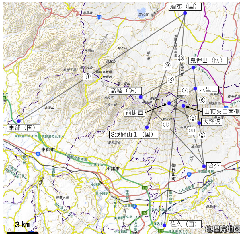
図7 浅間山 地殻変動連続観測点配置図 (防)：国立研究開発法人防災科学技術研究所、(国)：国土地理院 GNSS 基線③は図4⑨に対応しています。また、GNSS 基線①~③及び⑤~⑩は図6の①~③及び⑤~⑩にそれぞれ対応しています。 光波測距離線④は図4の⑩、図6-1の④に対応しています。
