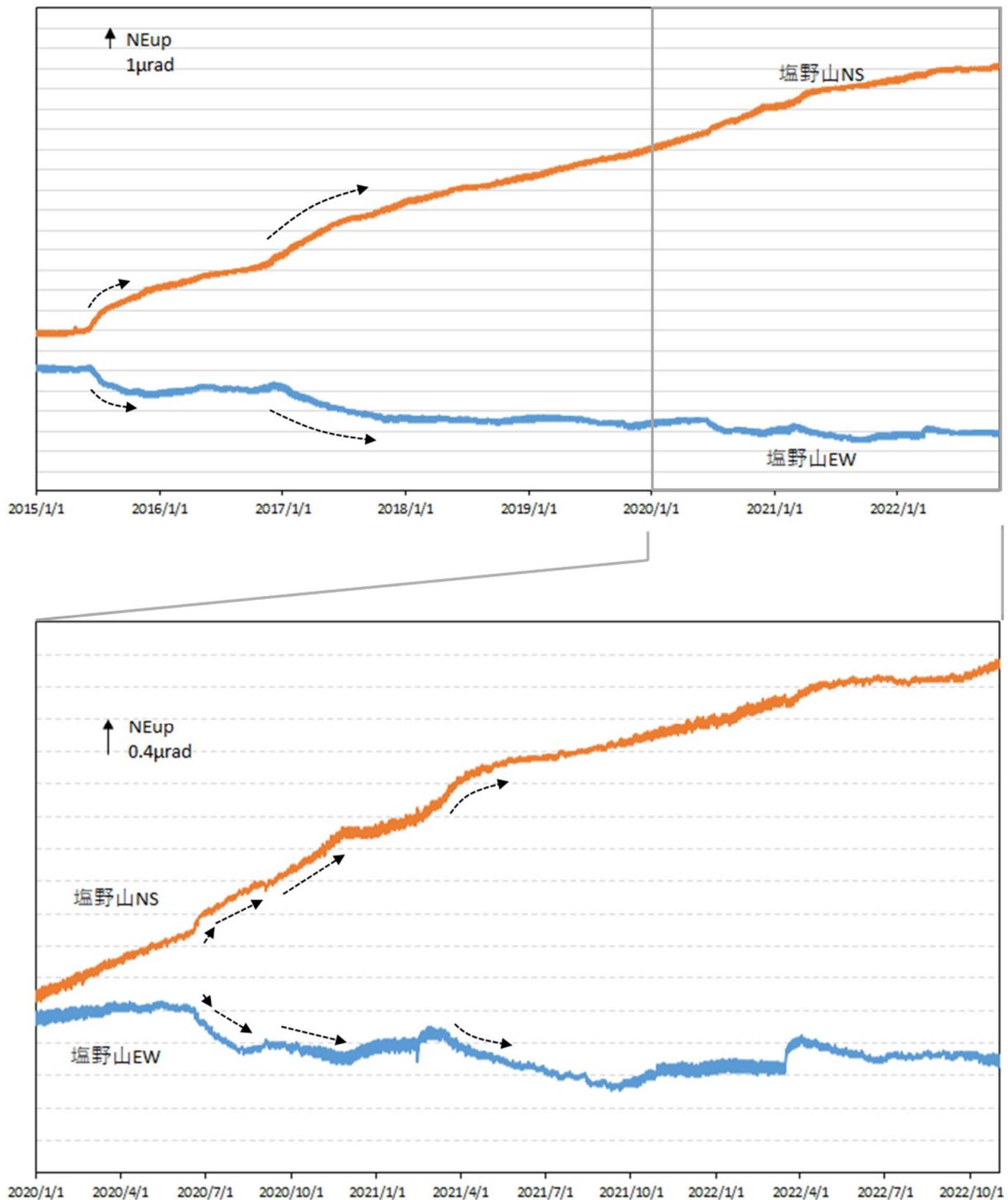
図8 浅間山 塩野山観測点における傾斜データ（2015年1月1日～2022年10月31日）
