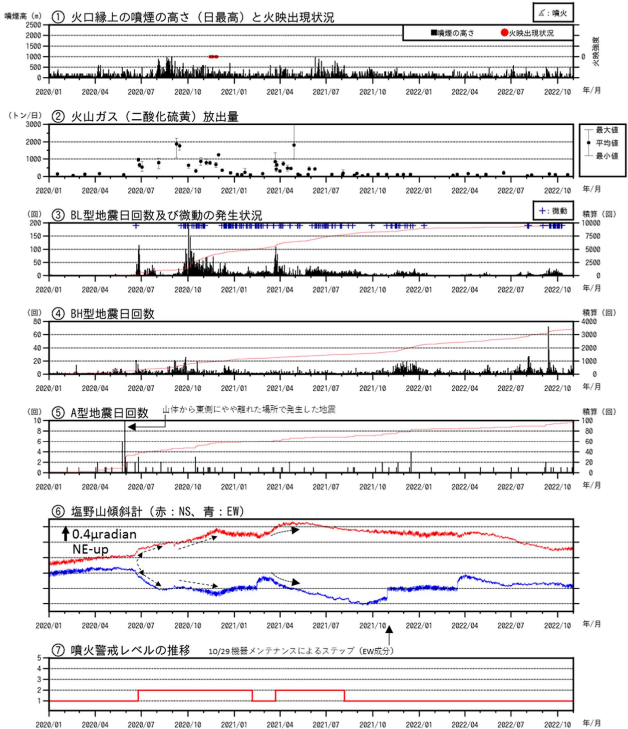
図3 浅間山 火山活動経過図（2020年1月1日～2022年10月31日）
