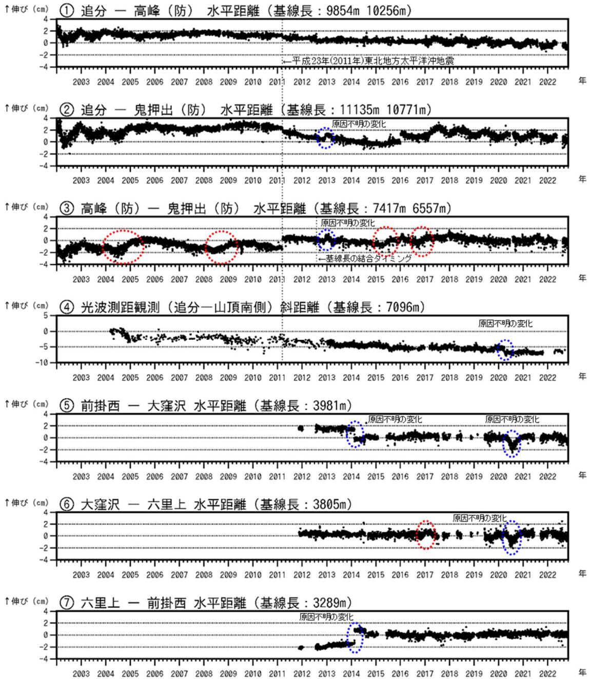
図6-1 浅間山 GNSS 連続観測及び光波測距観測の結果(2002年1月1日~2022年10月31日)
