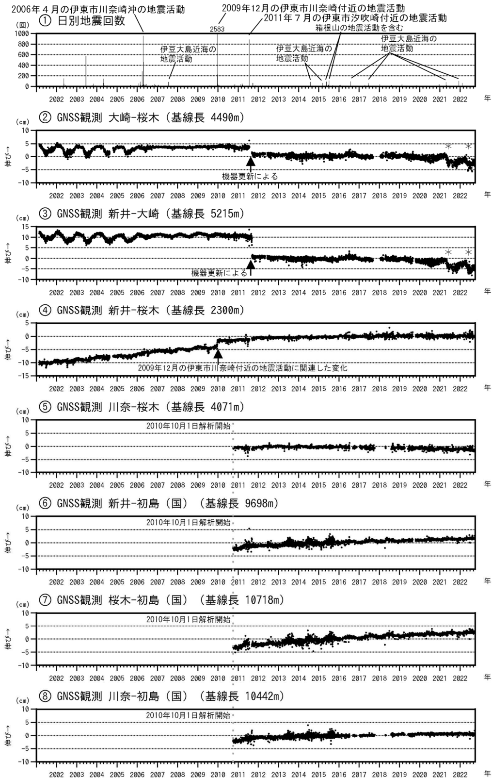
図3 伊豆東部火山群 火山活動経過図（2001年1月1日～2022年9月30日）
