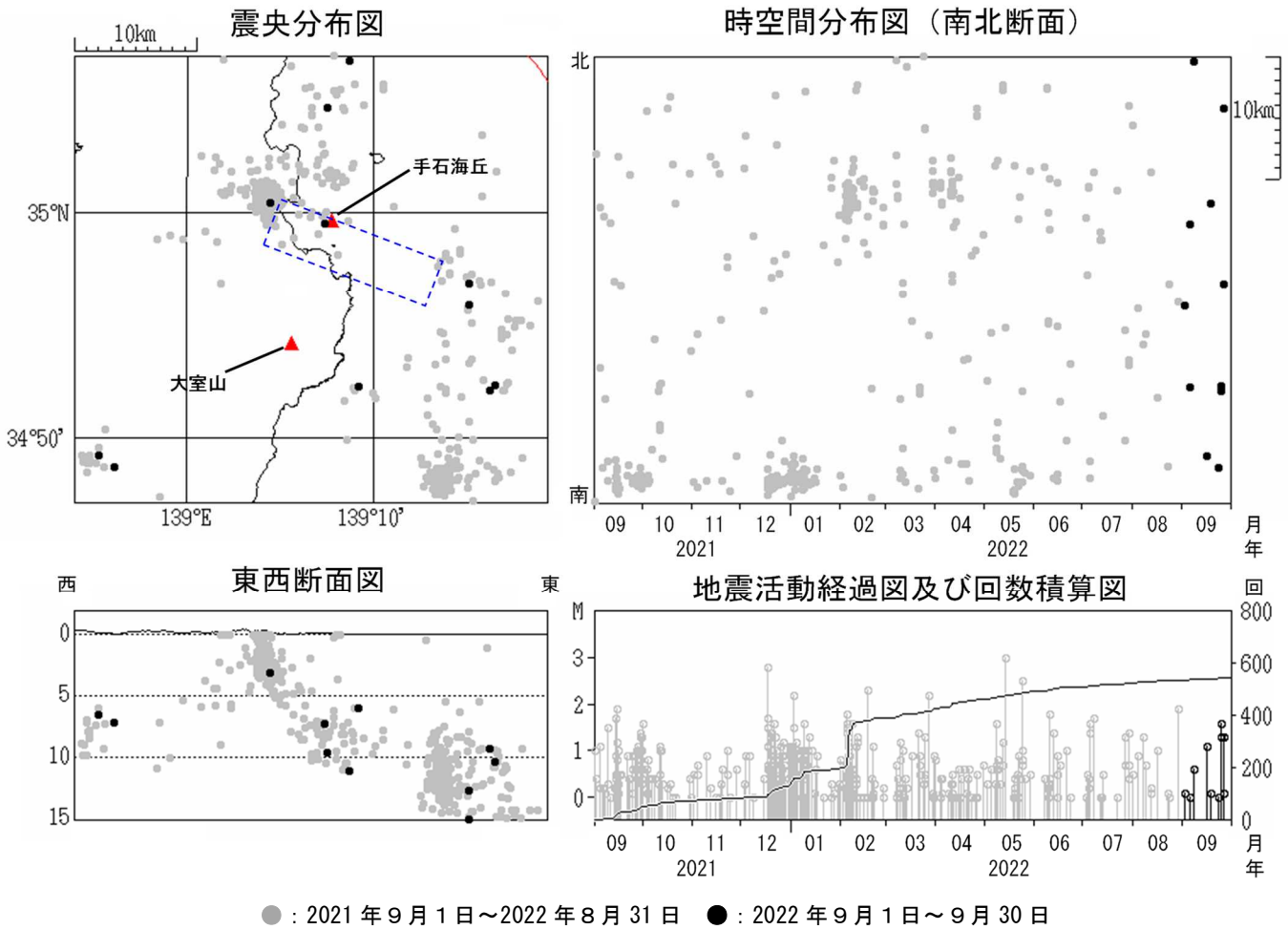
図2 伊豆東部火山群 広域地震観測網による震源分布図（2021年9月1日～2022年9月30日） □の領域は群発地震活動の発生する可能性がある範囲（火口が出現する可能性のある範囲）を示しています。 ( https://www.data.jma.go.jp/vois/data/tokyo/STOCK/level/PDF/level_316.pdf ) 広域地震観測網により震源決定したもので、深さは全て海面以下として決定しています。 M（マグニチュード）は地震の規模を表し、M0.0以上を表示しています。 図中の震源要素は一部暫定値が含まれており、後日変更することがあります。 この図では、関係機関の地震波形を一元的に処理し、地震観測点の標高を考慮する等した手法で得られた震源を用いています。
