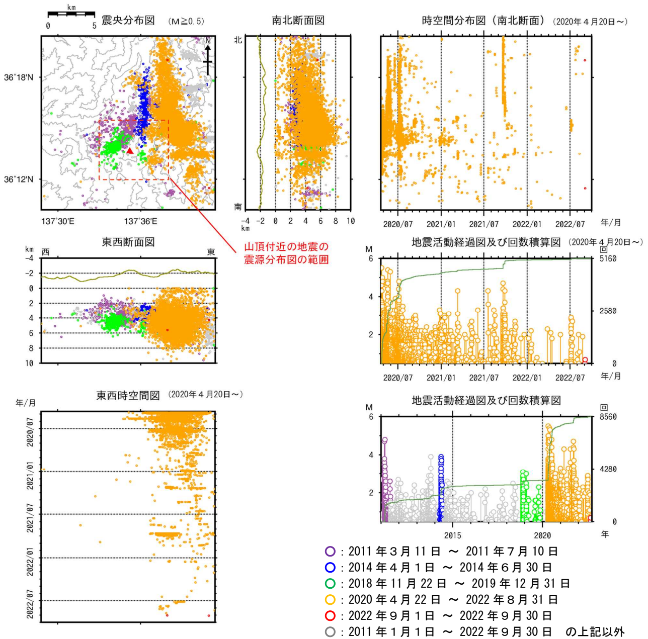
図9 焼岳 広域地震観測網による山体及び周辺の地震活動(2011年1月1日～2022年9月30日) 広域地震観測網により震源決定したもので、深さは全て海面以下として決定しています。そのため、山頂付近の浅い地震の震源も海面下に決定されています。 M(マグニチュード)は地震の規模を表します。 図中の震源要素は一部暫定値が含まれており、後日変更することがあります。 地震活動経過図及び回数積算図の緑色線は積算回数を示し、右軸で表されます。 震央分布図中の赤破線領域が、図2で示す領域に対応しています。
