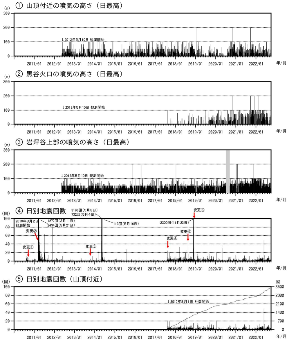
図5 焼岳 噴気の高さと地震回数の推移(2010年8月2日～2022年9月30日)
