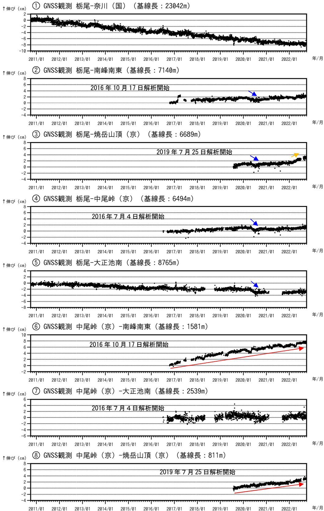
図6 焼岳 GNSS 連続観測による基線長変化（2010年10月1日～2022年9月30日） 図7のGNSS基線①～⑧に対応しています。グラフの空白部分は欠測を示します。（国）は国土地理院、（京）は京都大学の観測点です。
