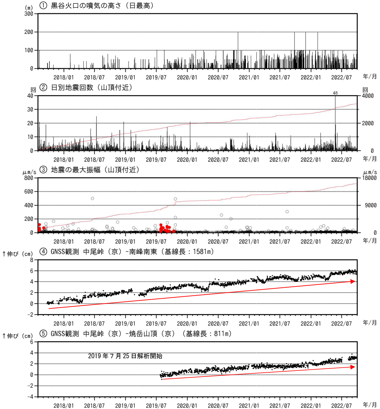
図1 焼岳 火山活動経過図（2017年8月1日～2022年9月30日）
