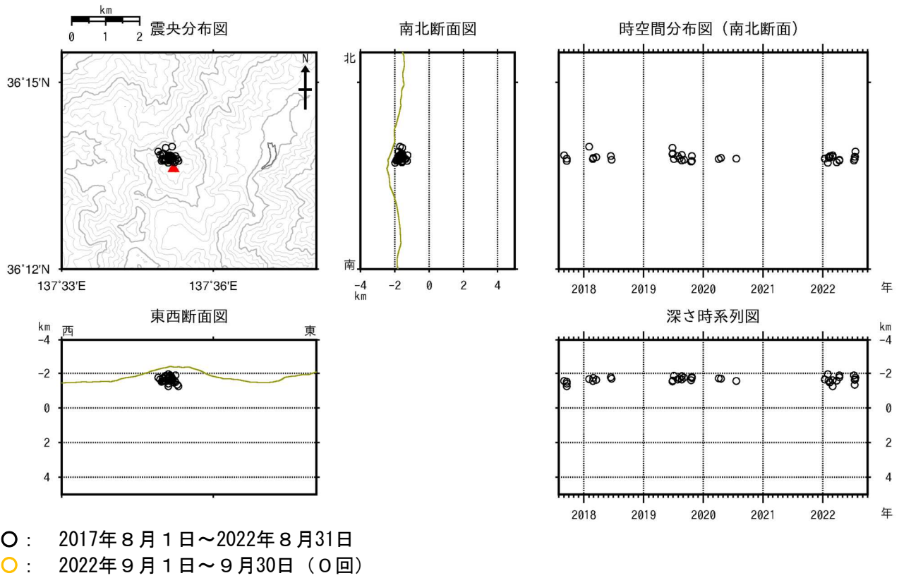
図2 焼岳 山頂付近の地震の震源分布図（2017年8月1日～2022年9月30日）
