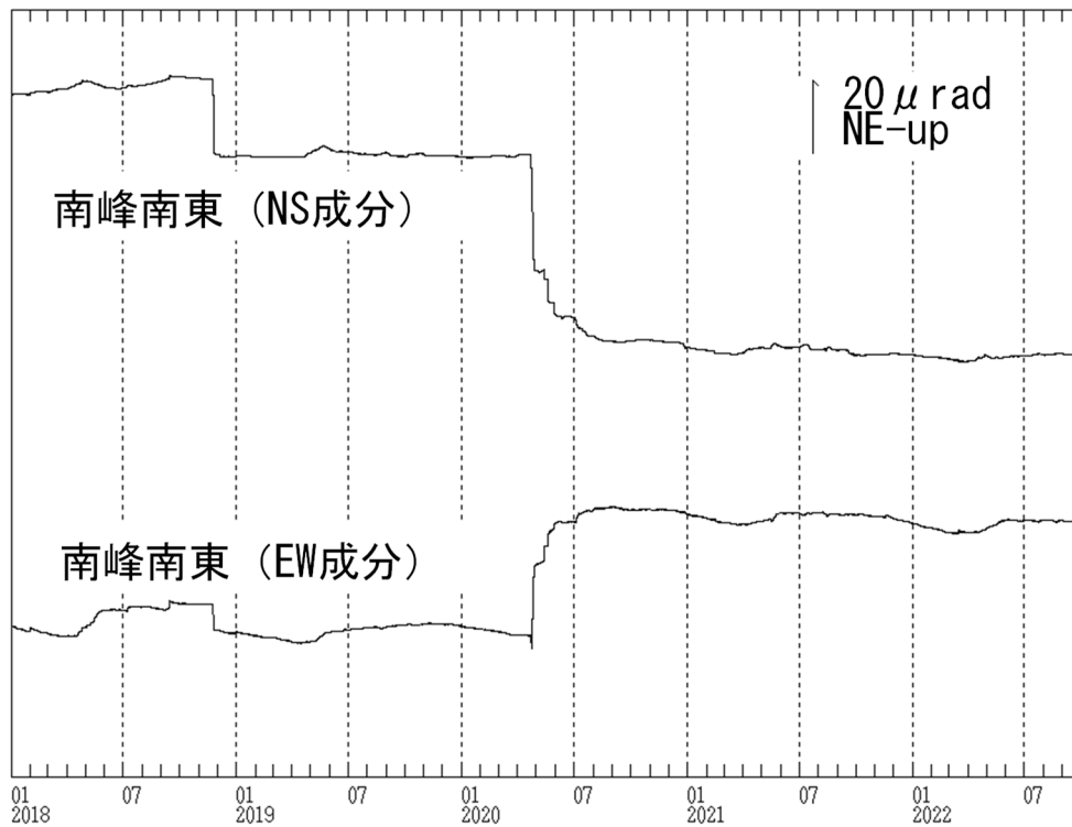
図8 焼岳 南峰南東観測点における傾斜データ（2018年1月1日～2022年9月30日）
