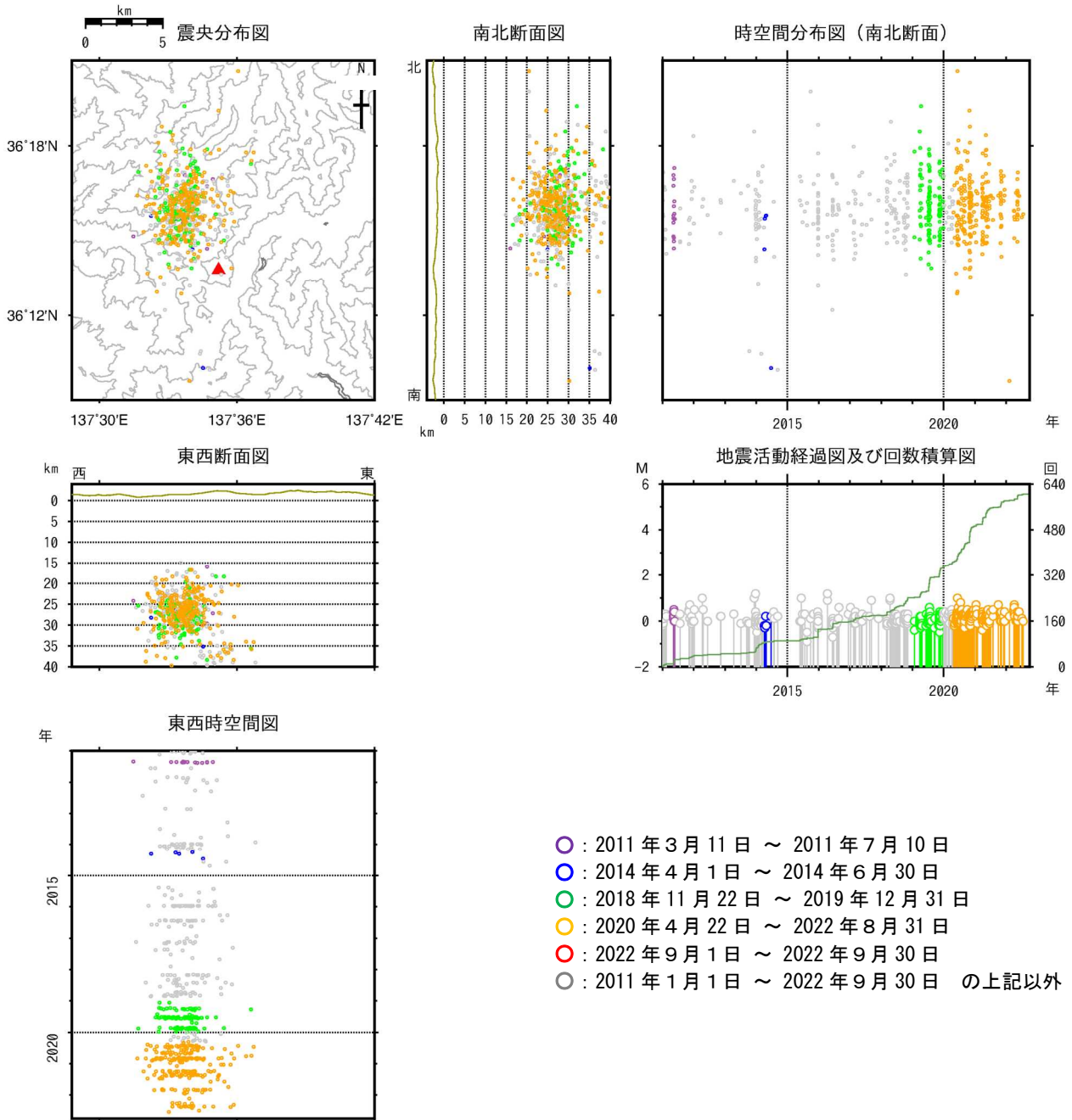
図10 焼岳 広域地震観測網による深部低周波地震の震源分布図（2011年1月1日～2022年9月30日） 広域地震観測網により震源決定したもので、深さは全て海面以下として決定しています。そのため、山頂付近の浅い地震の震源も海面下に決定されています。 M（マグニチュード）は地震の規模を表します。 図中の震源要素は一部暫定値が含まれており、後日変更することがあります。
