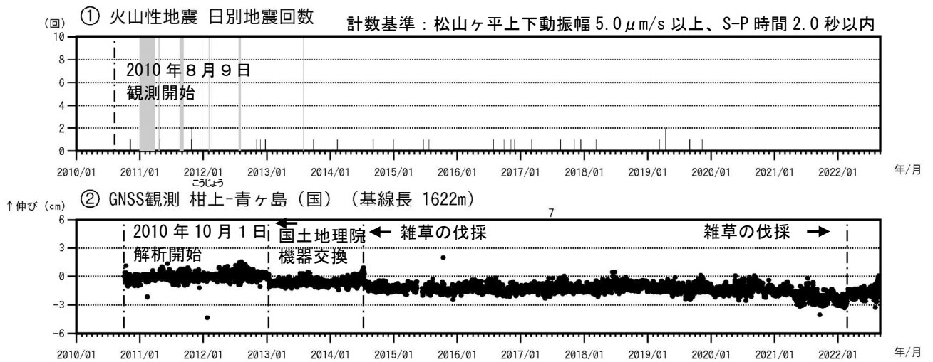
図3 青ヶ島 火山活動経過図（2010年8月9日～2022年8月31日）
