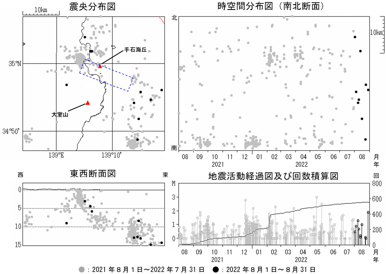
図2 伊豆東部火山群 広域地震観測網による震源分布図（2021年8月1日～2022年8月31日） □の領域は群発地震活動の発生する可能性がある範囲（火口が出現する可能性のある範囲）を示しています。 ( https://www.data.jma.go.jp/vois/data/tokyo/STOCK/level/PDF/level_316.pdf ) 広域地震観測網により震源決定したもので、深さは全て海面以下として決定しています。 M（マグニチュード）は地震の規模を表し、M0.0以上を表示しています。 図中の震源要素は一部暫定値が含まれており、後日変更することがあります。 この図では、関係機関の地震波形を一元的に処理し、地震観測点の標高を考慮する等した手法で得られた震源を用いています。
