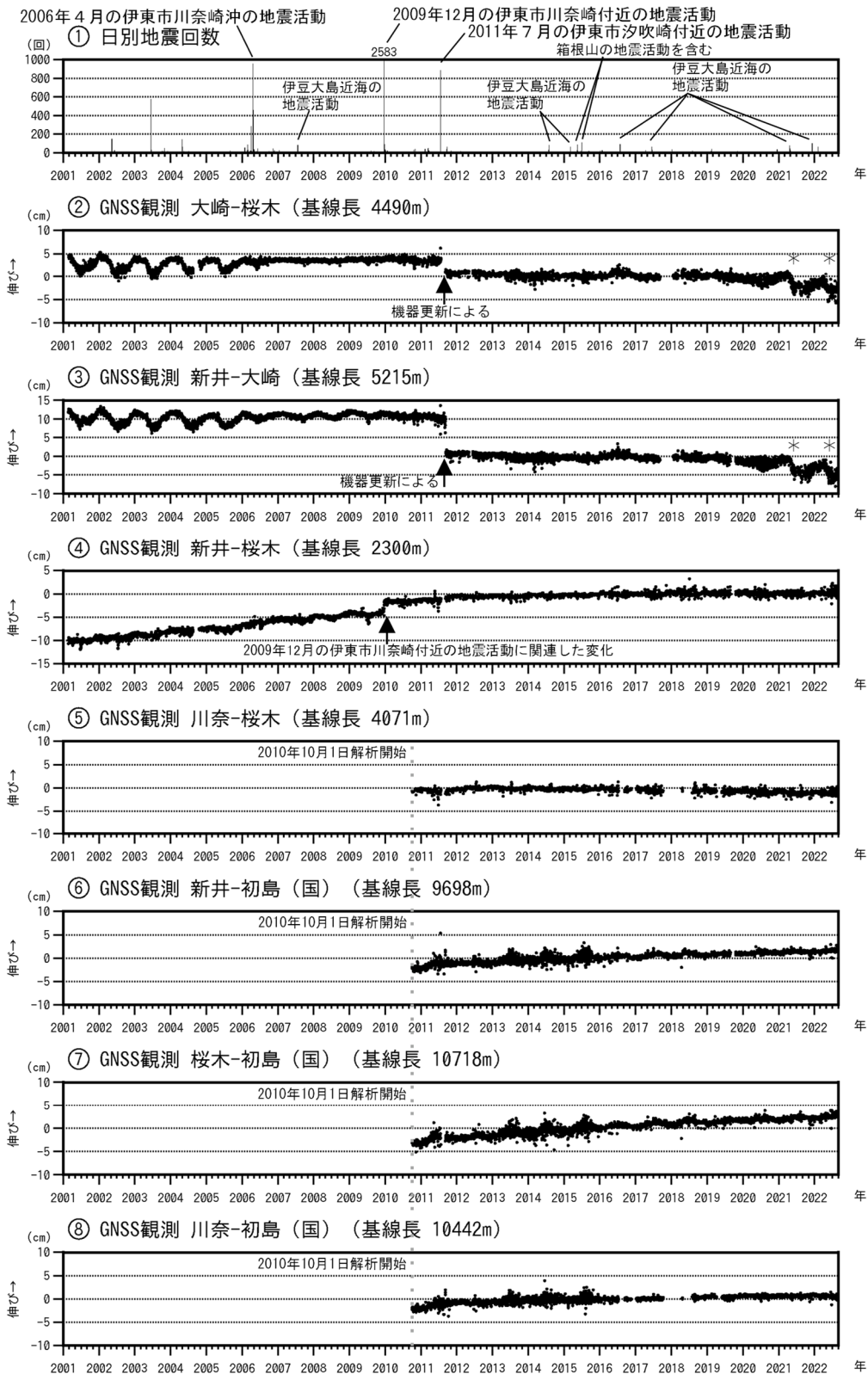
図3 伊豆東部火山群 火山活動経過図（2001年1月1日～2022年8月31日）
