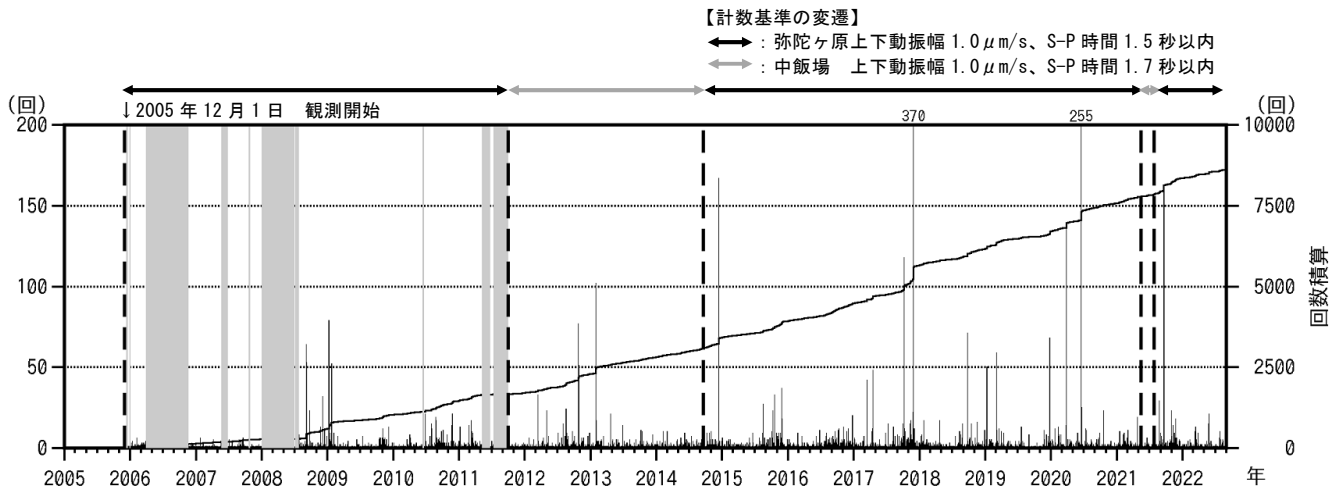
図3 白山 日別地震回数と積算回数（2005年12月1日～2022年8月31日） 図の灰色部分は機器障害による欠測期間
