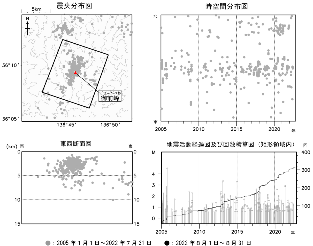
図4 白山 広域地震観測網による山体・周辺の地震活動（2005年1月1日～2022年8月31日）
