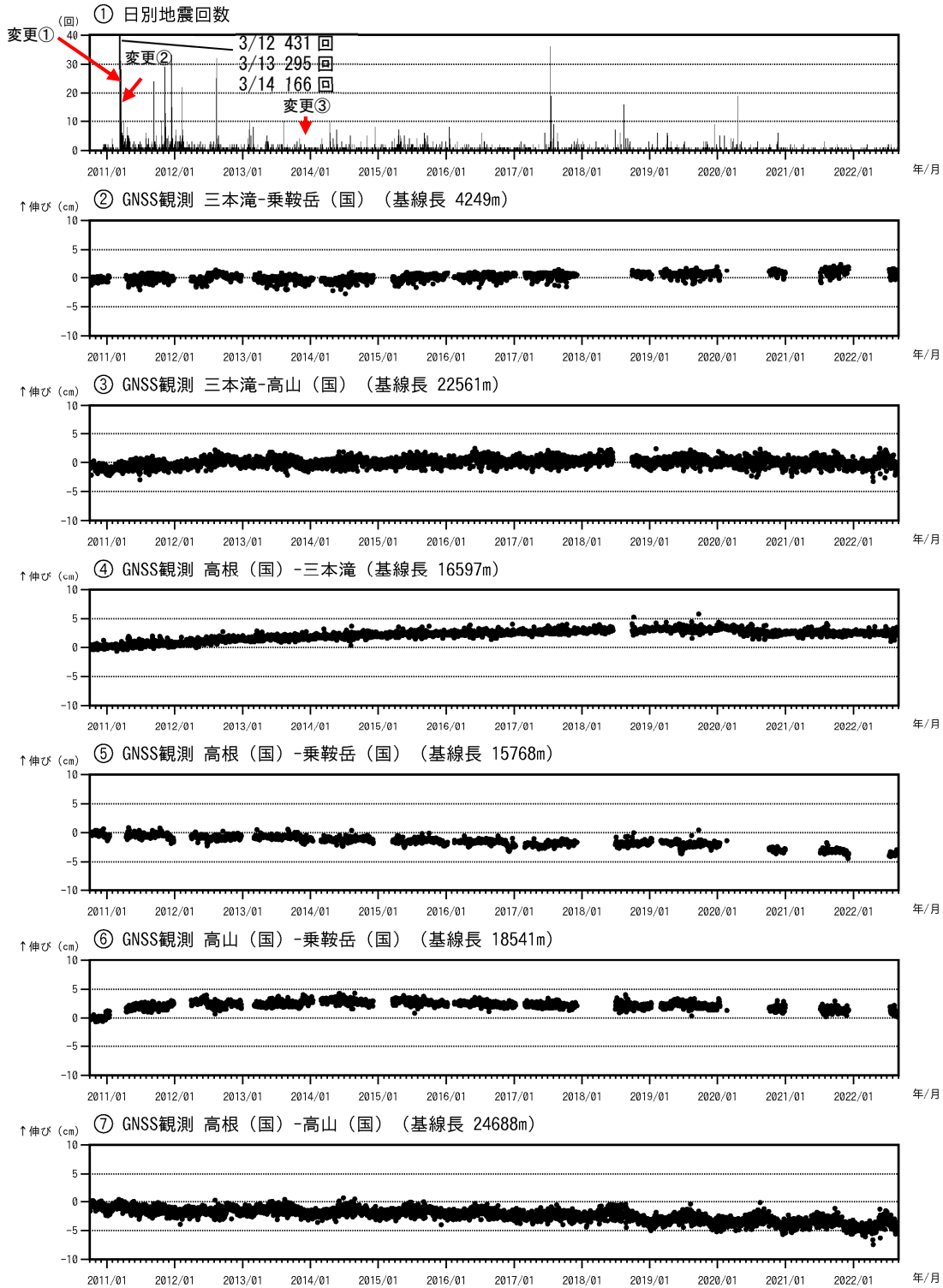
図2 乗鞍岳 火山活動経過図（2010年10月1日～2022年8月31日）
