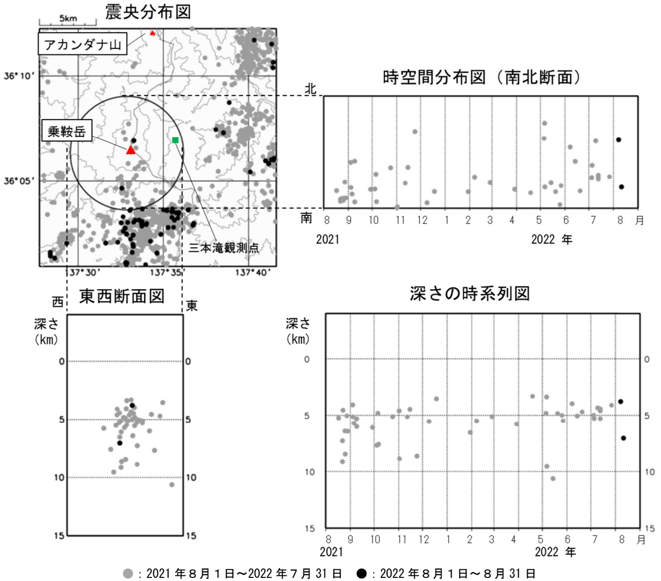
図3 乗鞍岳 広域地震観測網による山体・周辺の地震活動(2021年8月1日～2022年8月31日) 広域地震観測網により震源決定したもので、深さは全て海面以下として決定しています。図中の震源要素は一部暫定値が含まれており、後日変更することがあります。 この図では、関係機関の地震波形を一元的に処理し、地震観測点の標高を考慮する等した手法で得られた震源を用いています。 東西断面図、時空間分布図及び深さの時系列図には、乗鞍岳付近（震央分布図中の黒線円の範囲）の地震を示しています。
