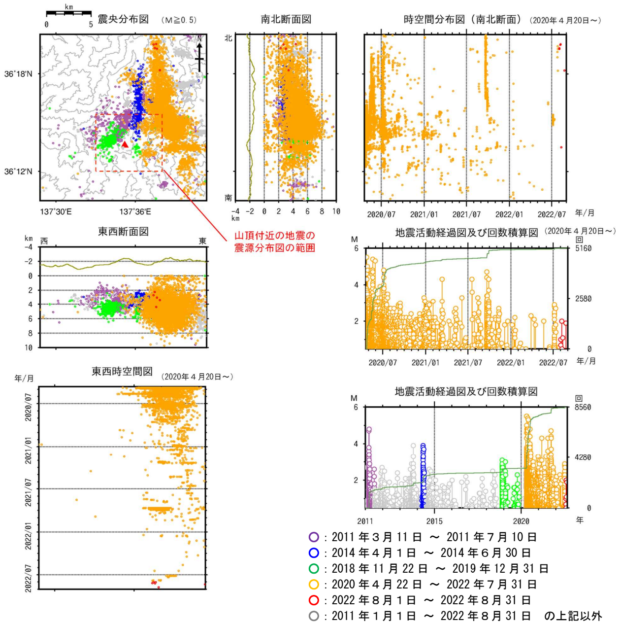
図13 焼岳 広域地震観測網による山体及び周辺の地震活動(2011年1月1日~2022年8月31日) 広域地震観測網により震源決定したもので、深さは全て海面以下として決定しています。そのため、山頂付近の浅い地震の震源も海面下に決定されています。 M (マグニチュード) は地震の規模を表します。 図中の震源要素は一部暫定値が含まれており、後日変更することがあります。 地震活動経過図及び回数積算図の緑色線は積算回数を示し、右軸で表されます。 震央分布図中の赤破線領域が、図2で示す領域に対応しています。
