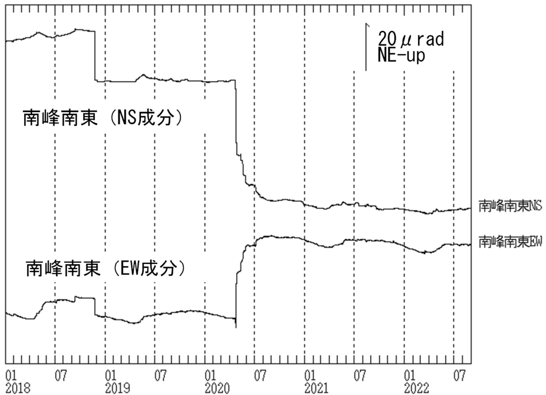
図 12 焼岳 南峰南東観測点における傾斜データ (2018年1月1日～2022年8月31日)
