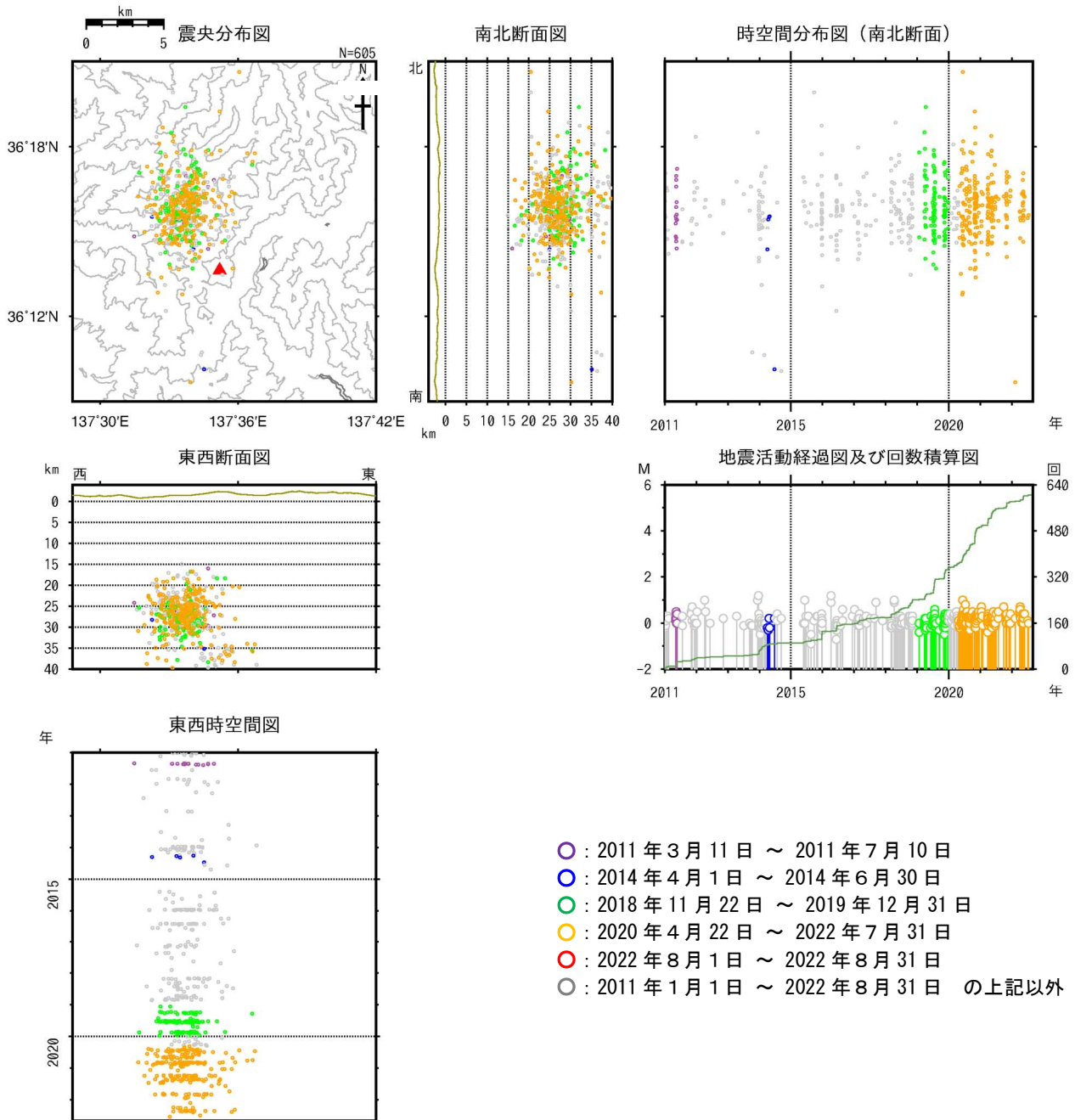
図14 焼岳 広域地震観測網による深部低周波地震の震源分布図（2011年1月1日～2022年8月31日） 広域地震観測網により震源決定したもので、深さは全て海面以下として決定しています。そのため、山頂付近の浅い地震の震源も海面下に決定されています。 M（マグニチュード）は地震の規模を表します。 図中の震源要素は一部暫定値が含まれており、後日変更することがあります。
