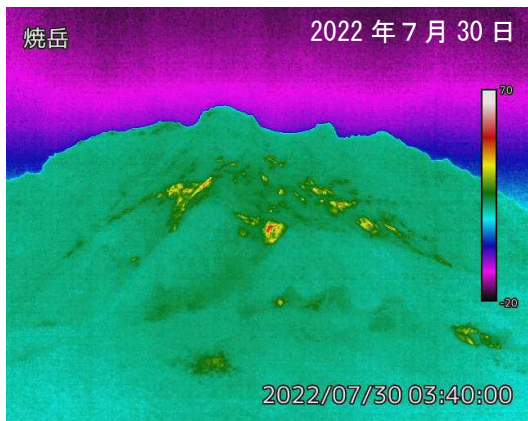
図4 焼岳 中尾峠赤外熱映像カメラによる焼岳の北側斜面の地表面温度分布と可視画像 撮影場所と撮影方向は図15を参照下さい。
