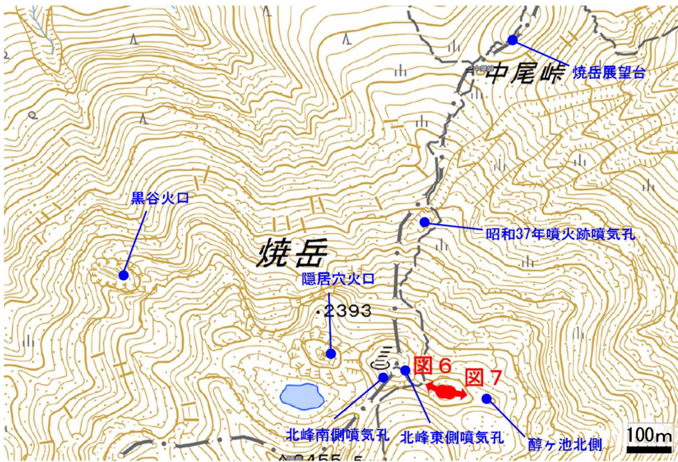
図5 焼岳 噴気孔位置および撮影位置（矢印は撮影方向を示す）
