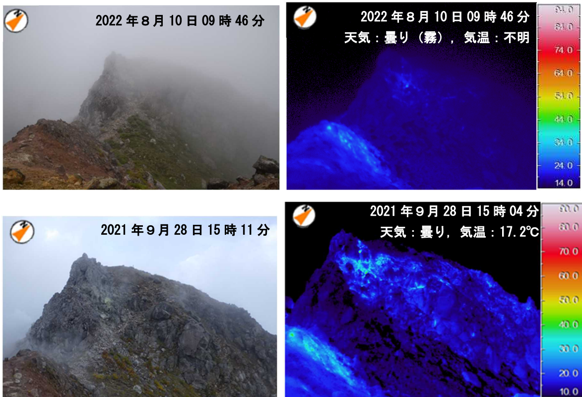
図6 焼岳 北峰東斜面の地表面温度分布
