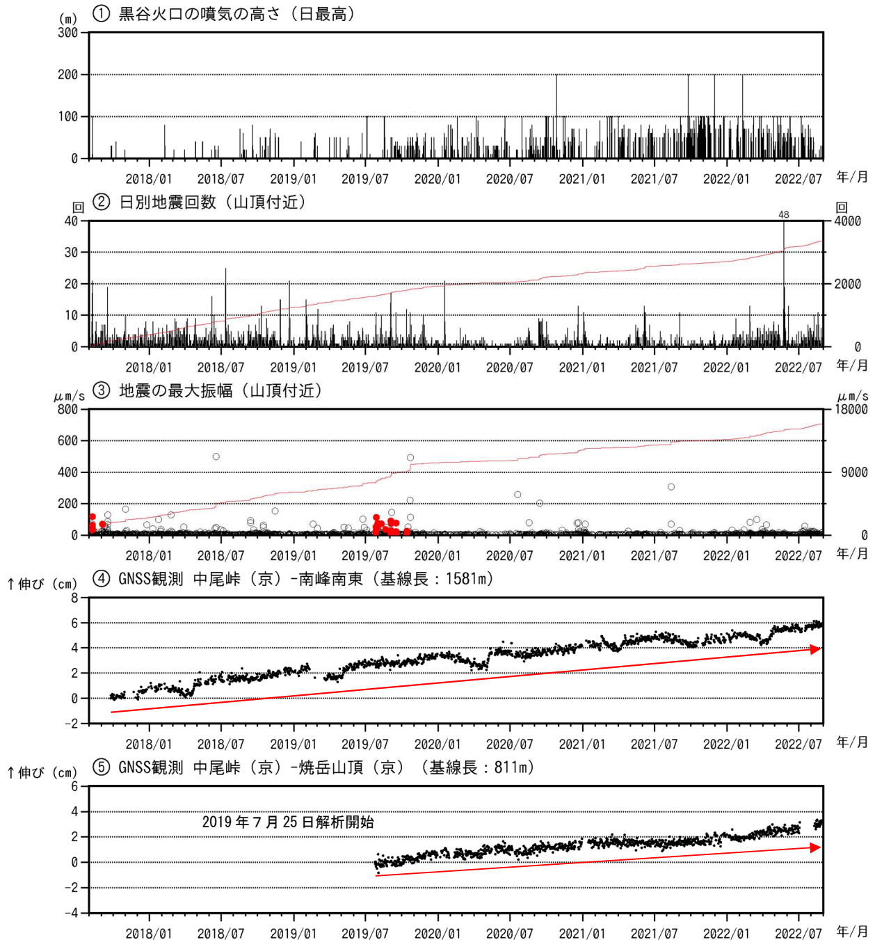
図1 焼岳 火山活動経過図（2017年8月1日～2022年8月31日）
