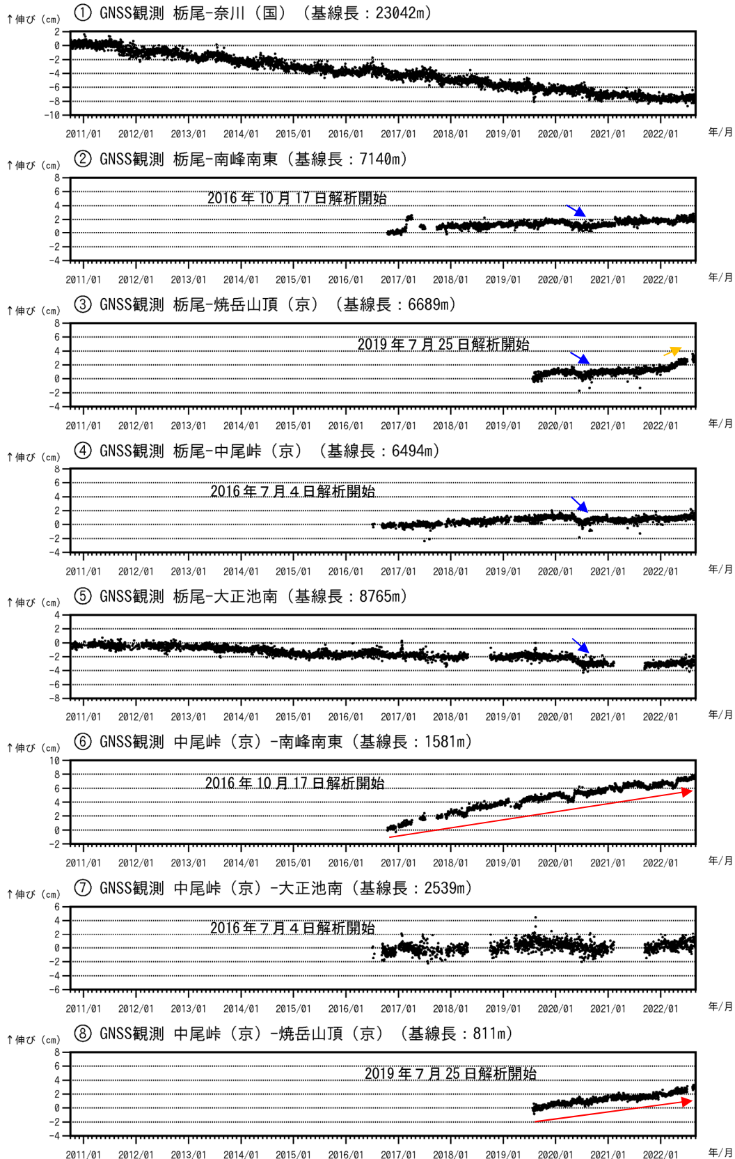
図10 焼岳 GNSS連続観測による基線長変化（2010年10月1日～2022年8月31日）
