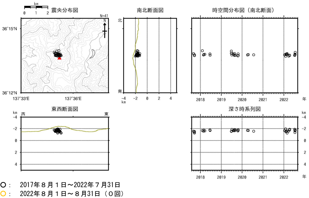
図2 焼岳 山頂付近の地震の震源分布図（2017年8月1日～2022年8月31日）
