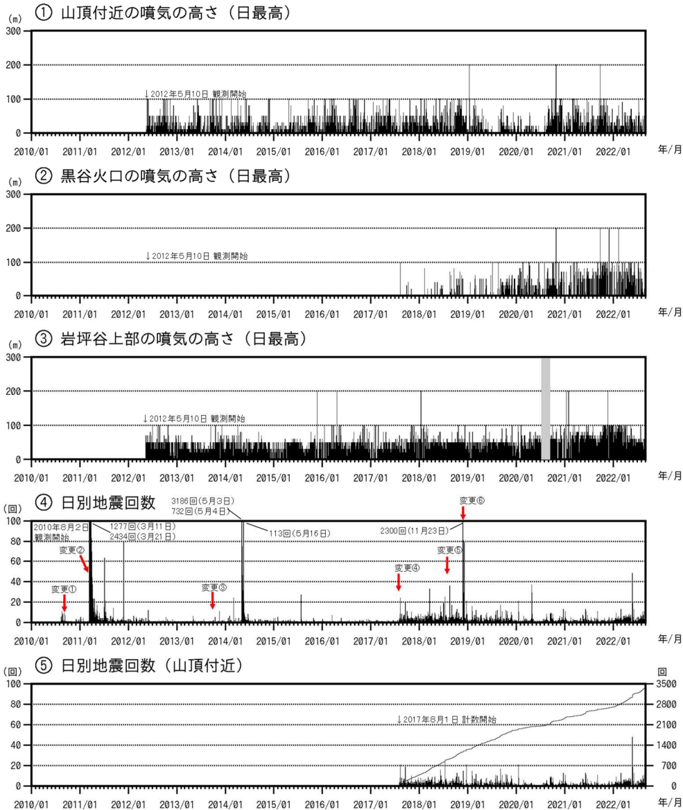
図9 焼岳 噴気の高さと地震回数の推移(2010年8月2日～2022年8月31日)
