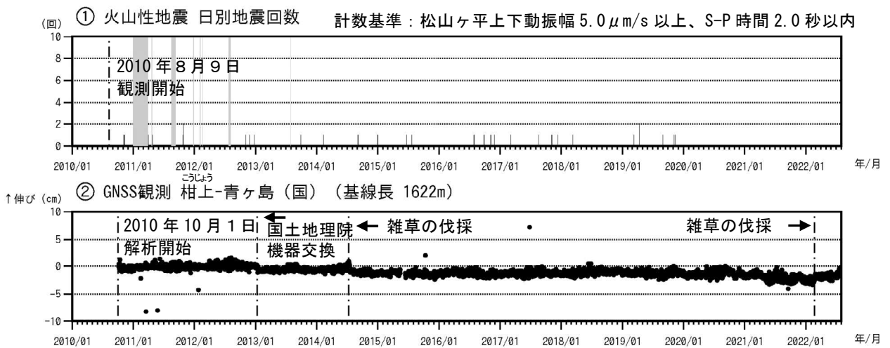
図3 青ヶ島 火山活動経過図（2010年8月9日～2022年7月31日）
