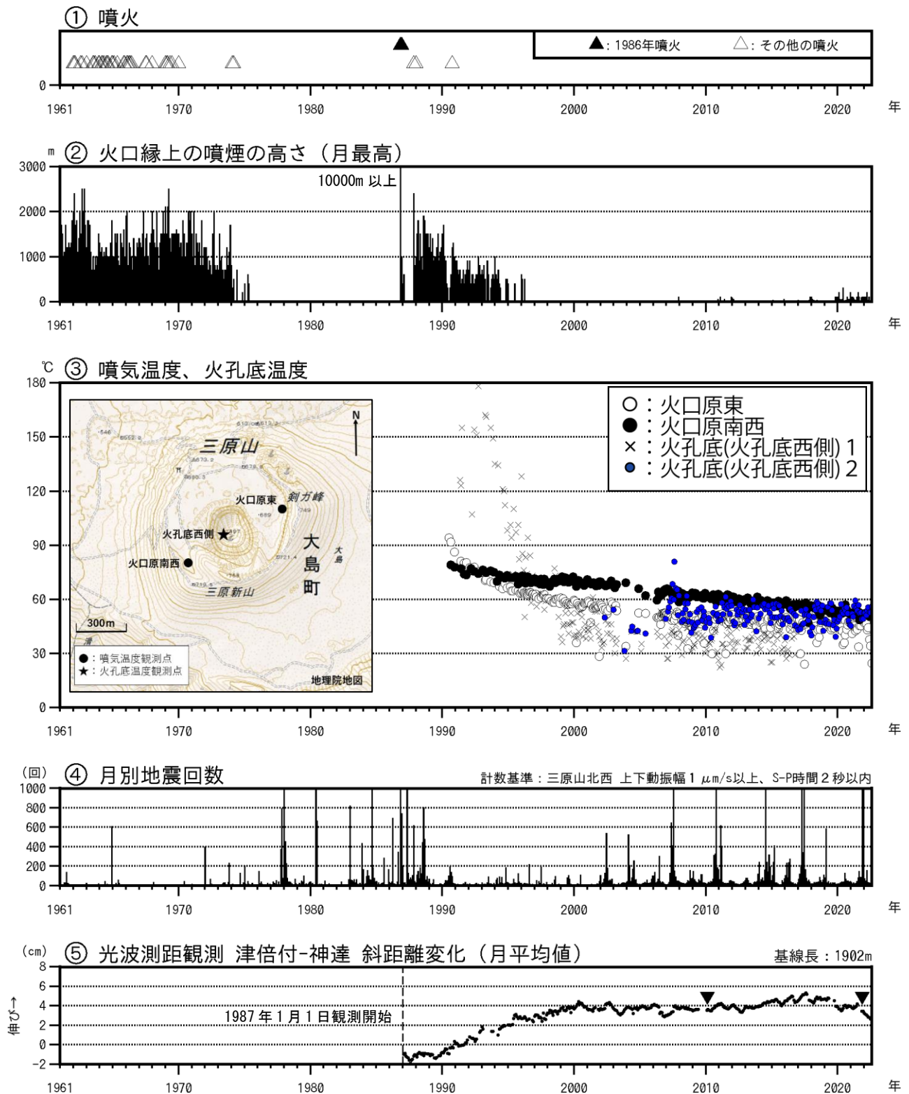
図1 伊豆大島 長期間の火山活動経過図（1961年1月～2022年7月31日）
