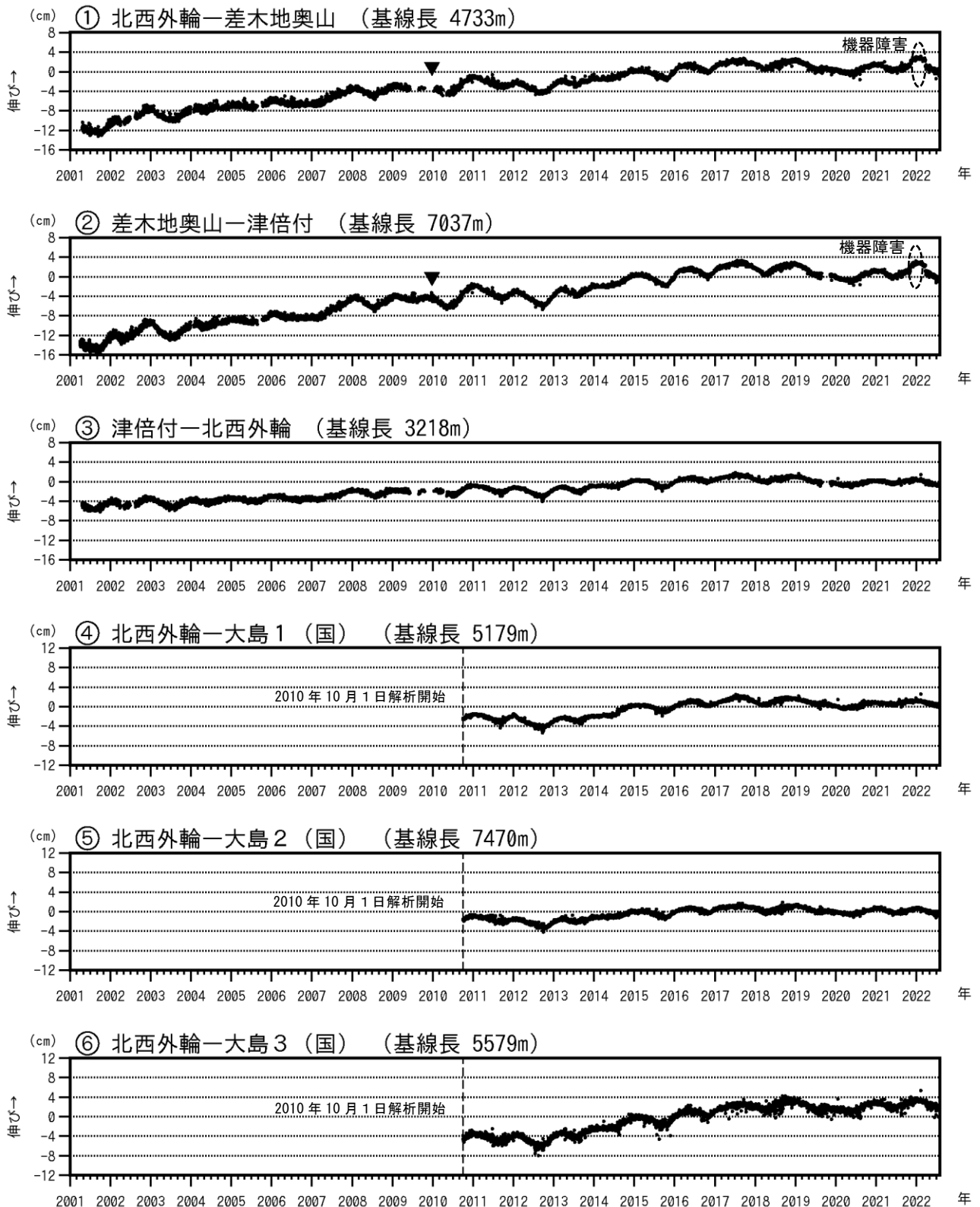
図3-1 伊豆大島 GNSS 連続観測による基線長変化(2001年1月～2022年7月31日)
