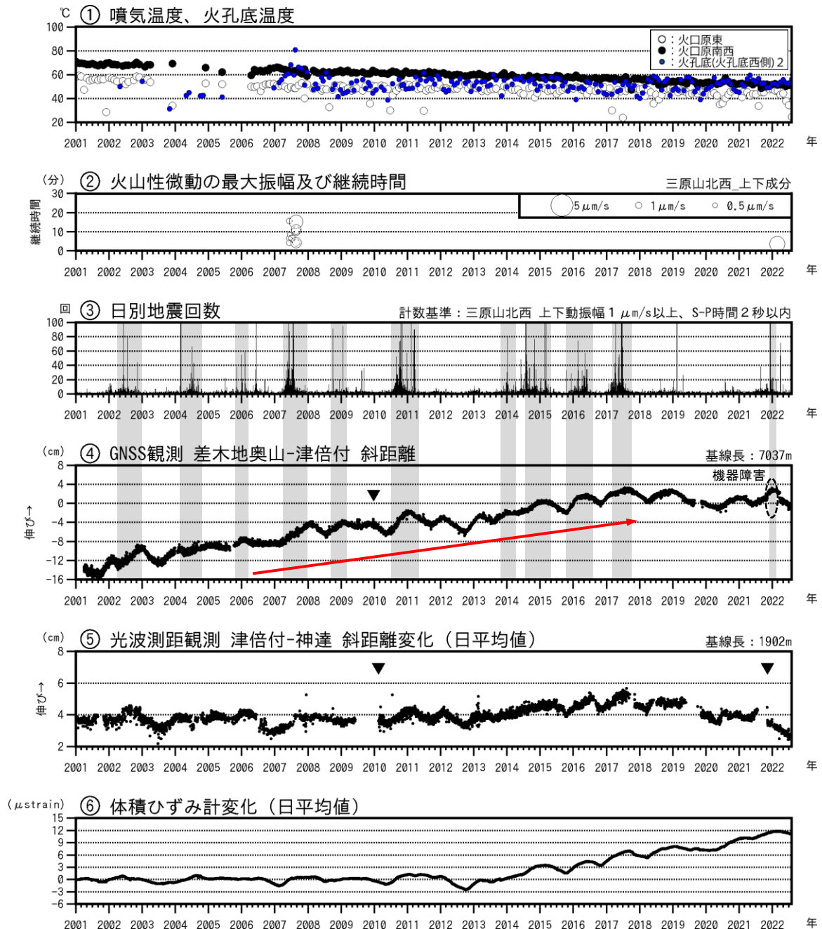
図2 伊豆大島 最近の火山活動経過図（2001年1月～2022年7月31日）
