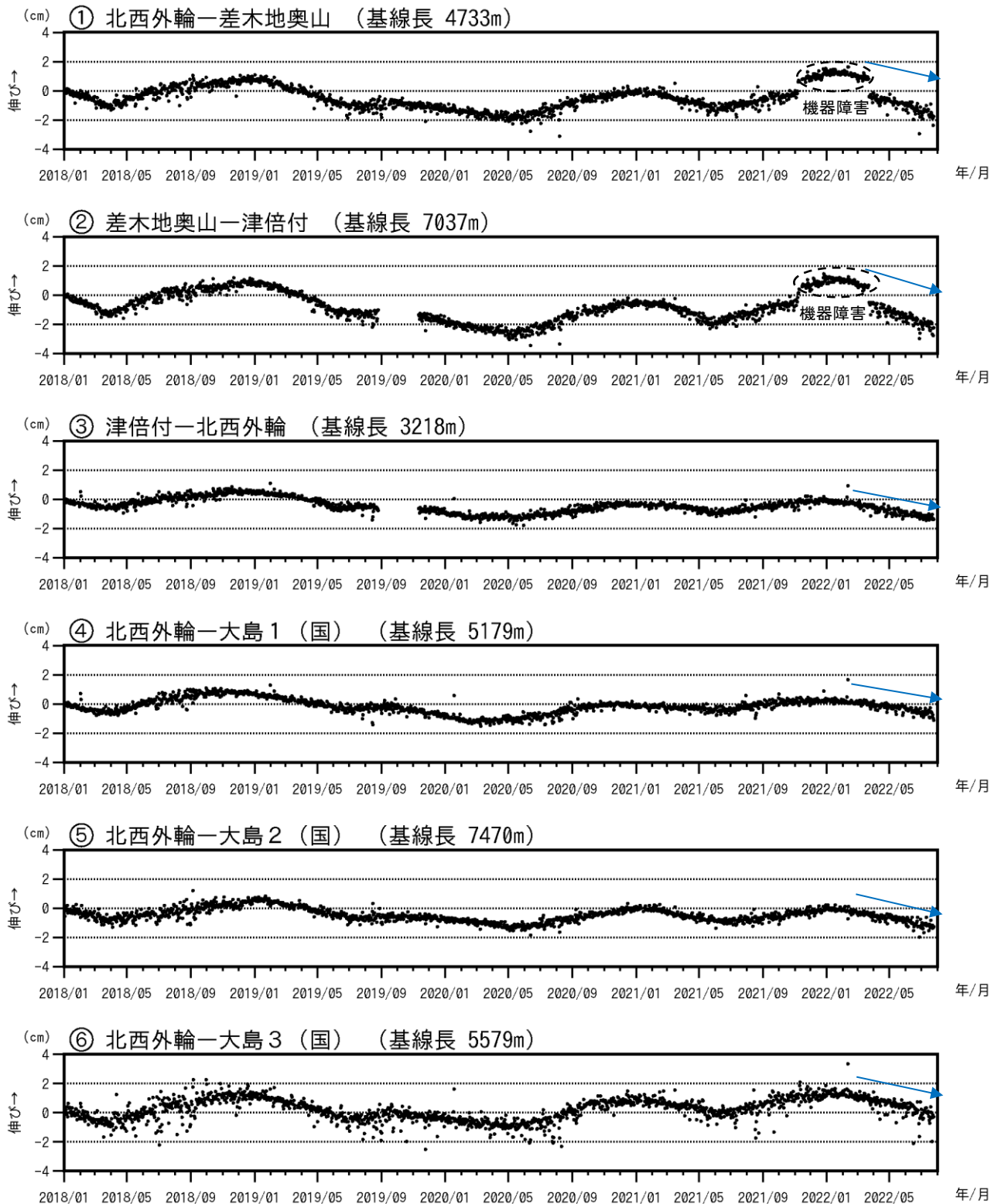
図3-2 伊豆大島 GNSS 連続観測による基線長変化(2018年1月～2022年7月31日)
