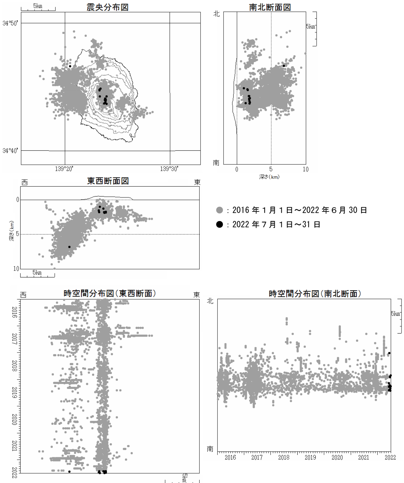
図4 伊豆大島 震源分布図（2016 年 1 月 1 日～2022 年 7 月 31 日）
