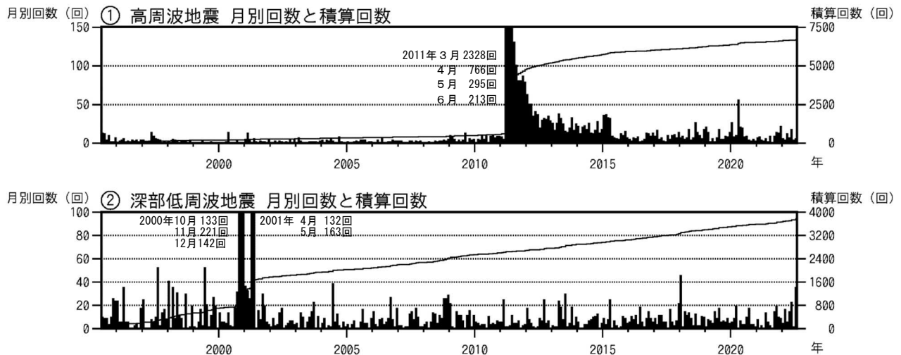
図2 富士山 月別地震回数（1995年6月1日～2022年7月31日）
