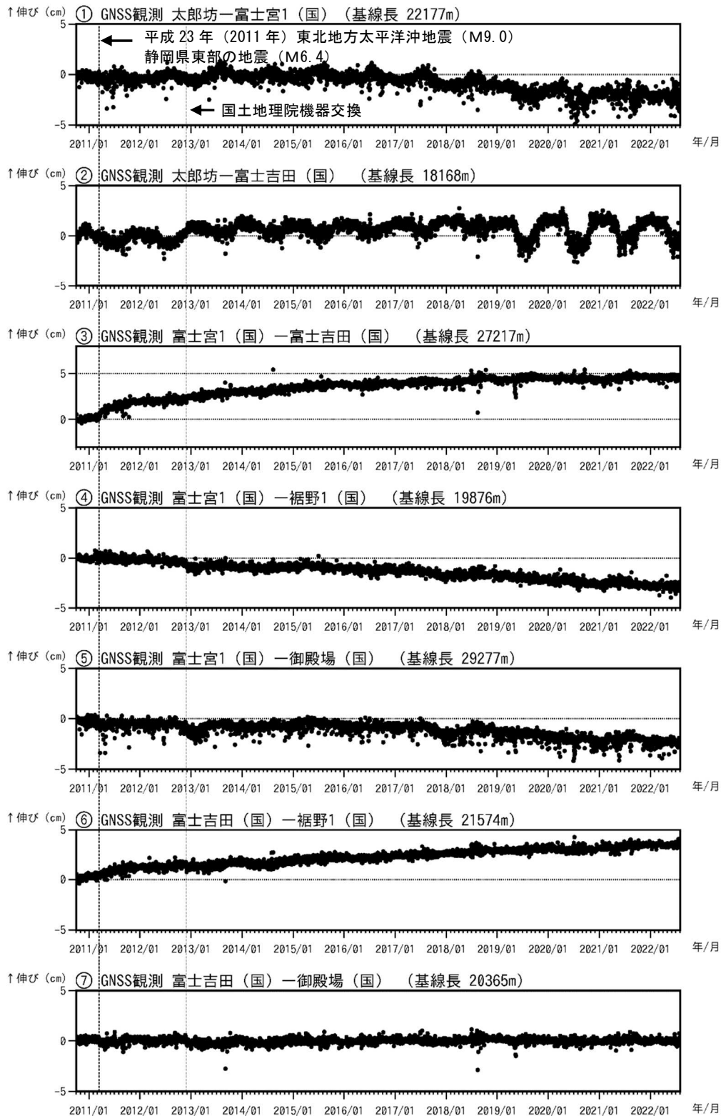
図4 富士山 GNSS 連続観測による基線長変化（2010年10月1日～2022年7月31日） （国）：国土地理院 「平成23年（2011年）東北地方太平洋沖地震」及び2011年3月15日に発生した静岡県東部の地震（M6.4）によるステップ状の変化を補正しています。 ①～⑦は図5のGNSS基線①～⑦に対応しています。
