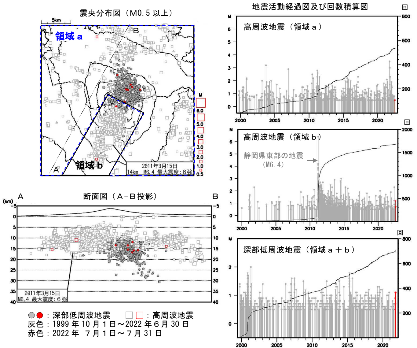
図3 富士山 広域地震観測網による山体及び周辺の地震活動（1999年10月1日～2022年7月31日）
