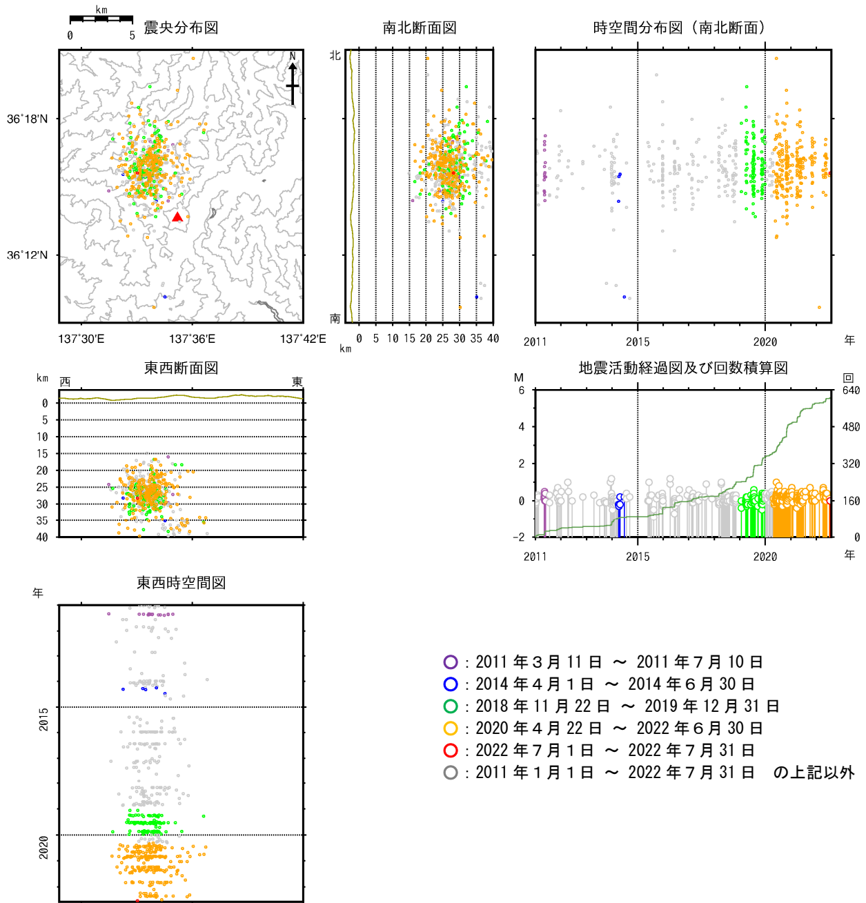
図11 焼岳 広域地震観測網による深部低周波地震の震源分布図（2011年1月1日～2022年7月31日） 広域地震観測網により震源決定したもので、深さは全て海面以下として決定しています。そのため、山頂付近の浅い地震の震源も海面下に決定されています。 M（マグニチュード）は地震の規模を表します。 図中の震源要素は一部暫定値が含まれており、後日変更することがあります。
