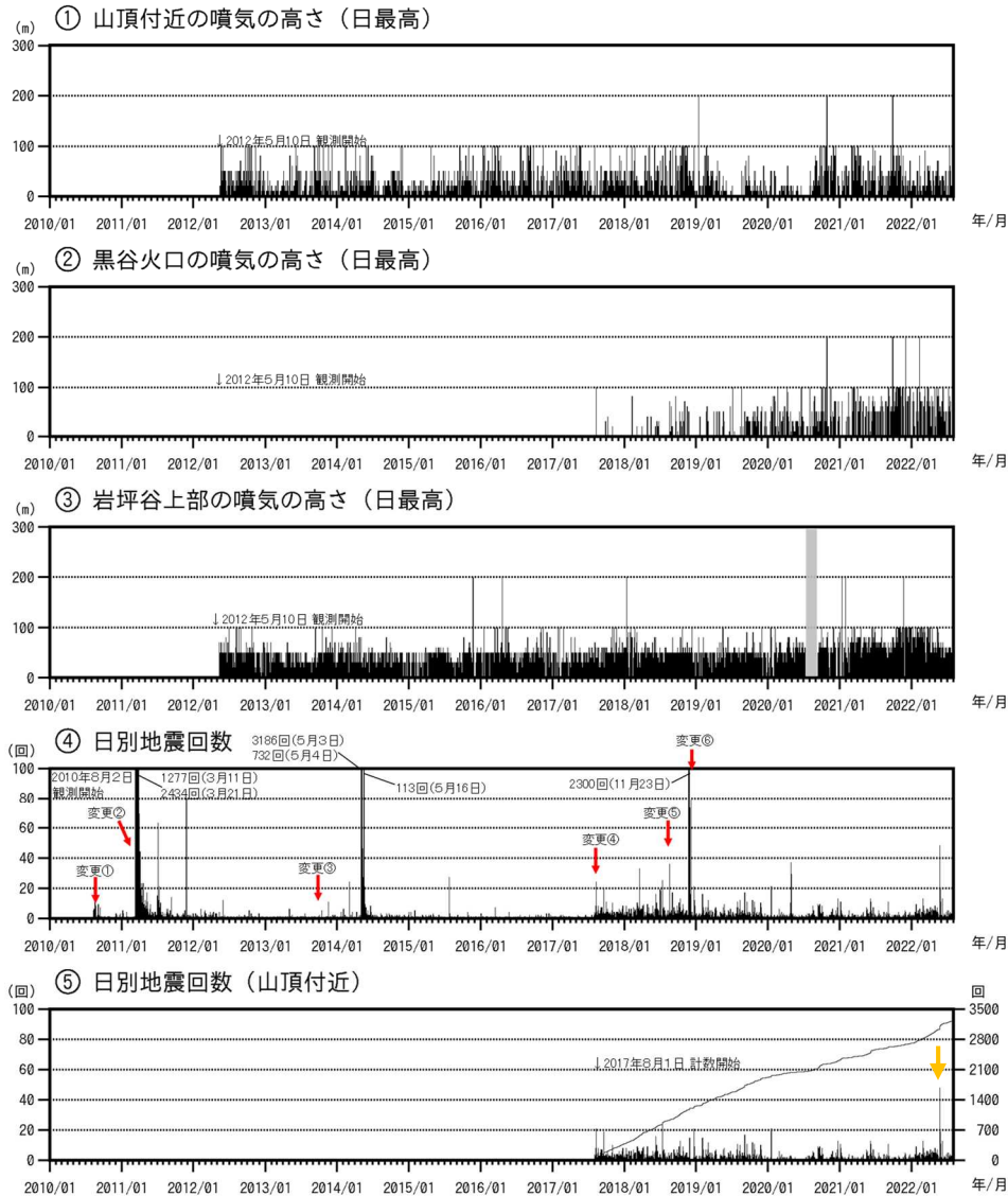
図6 焼岳 噴気の高さと地震回数の推移(2010年8月2日～2022年7月31日)
