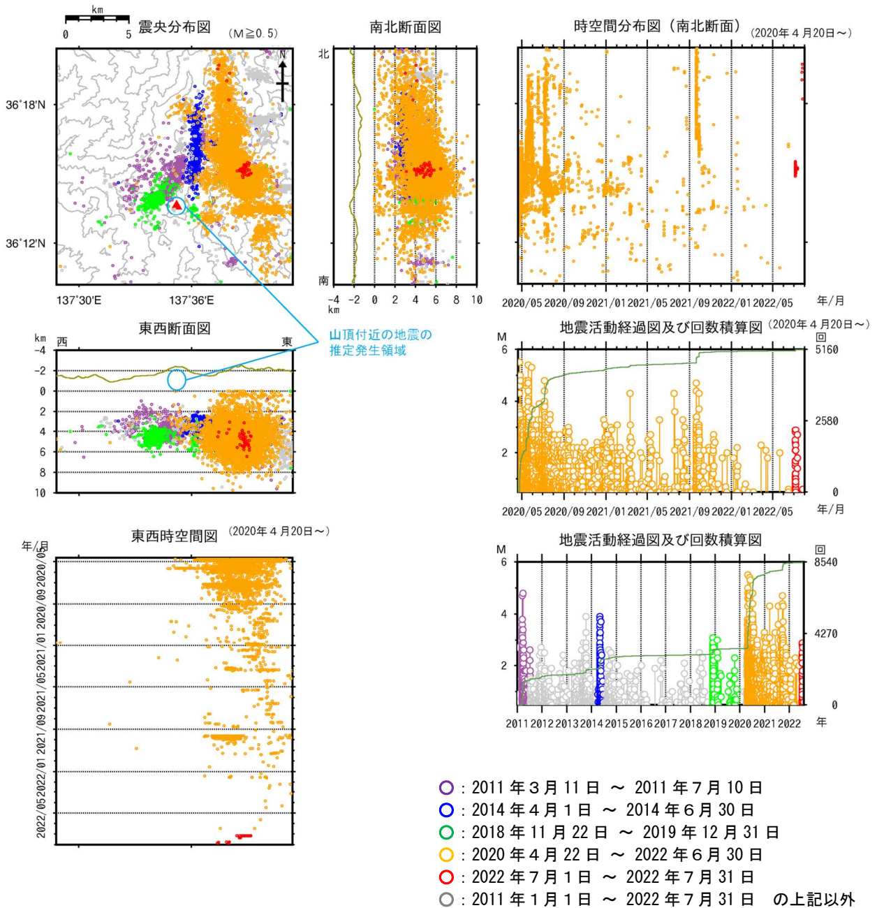
図10 焼岳 広域地震観測網による山体及び周辺の地震活動(2011年1月1日～2022年7月31日) 広域地震観測網により震源決定したもので、深さは全て海面以下として決定しています。そのため、山頂付近の浅い地震の震源も海面下に決定されています。 M (マグニチュード) は地震の規模を表します。 図中の震源要素は一部暫定値が含まれており、後日変更することがあります。 地震活動経過図及び回数積算図の緑色線は積算回数を示し、右軸で表されます。
