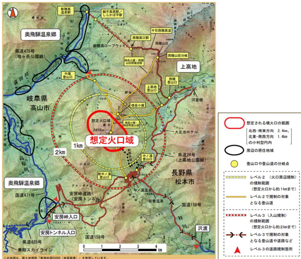
図1 焼岳 想定火口域
