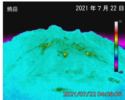
図5 焼岳 中尾峠赤外熱映像カメラによる焼岳の北側斜面の地表面温度分布と可視画像 撮影場所と撮影方向は図12を参照下さい。
