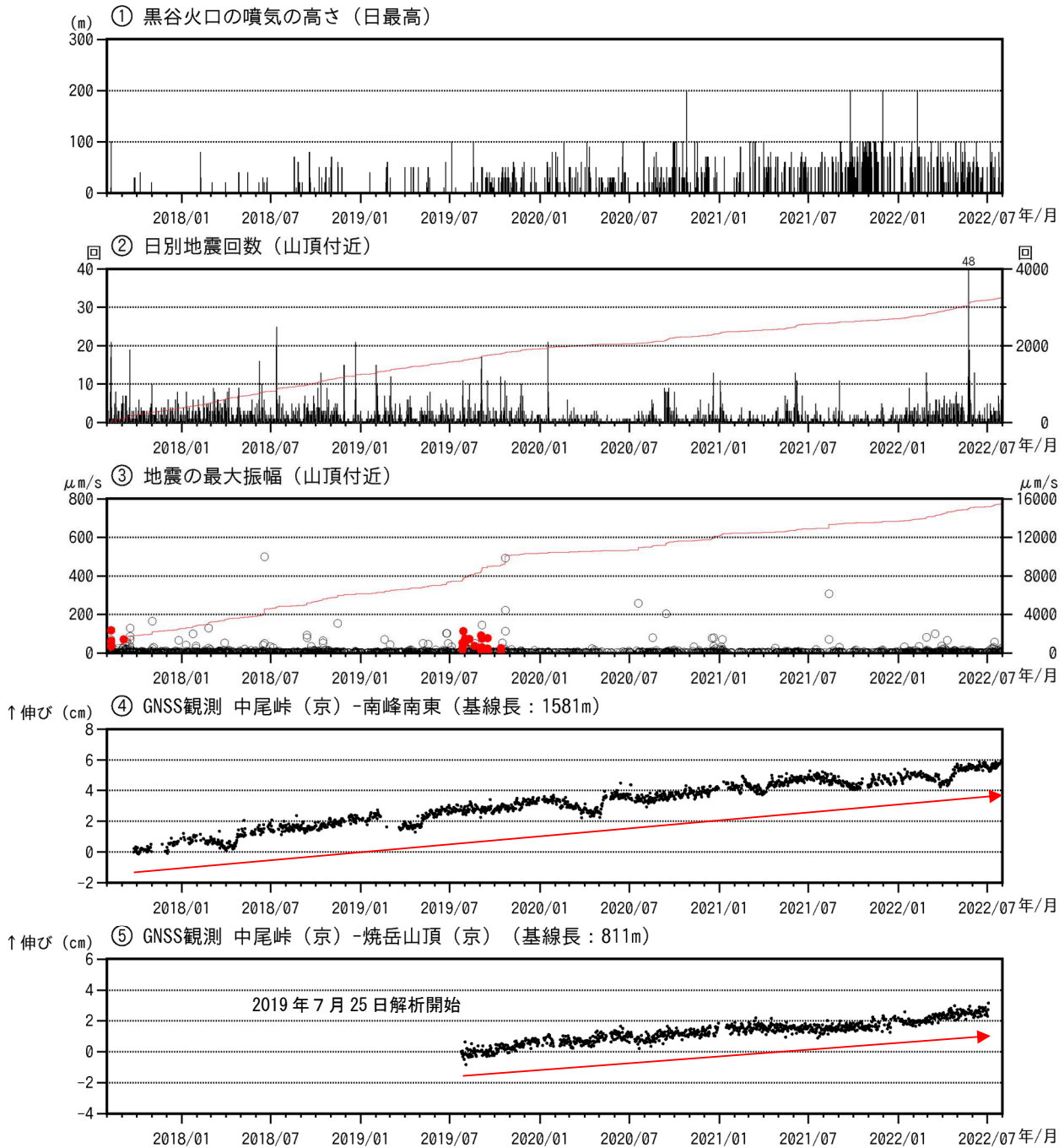
図3 焼岳 火山活動経過図（2017年8月1日～2022年7月31日）
