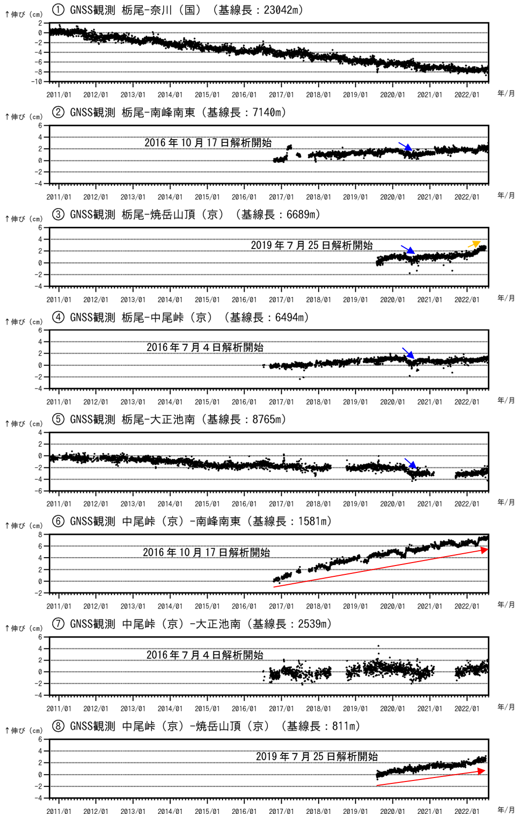
図7 焼岳 GNSS 連続観測による基線長変化（2010年10月1日～2022年7月31日）
