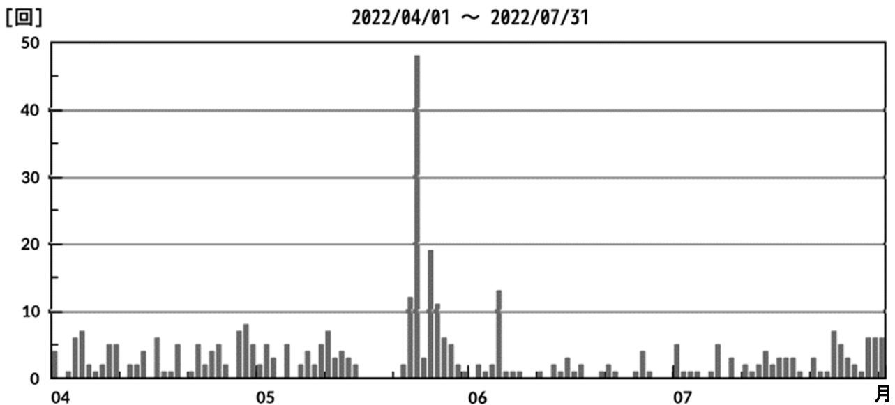
図2 焼岳 山頂付近の日別地震回数（2022年4月1日～7月31日）
