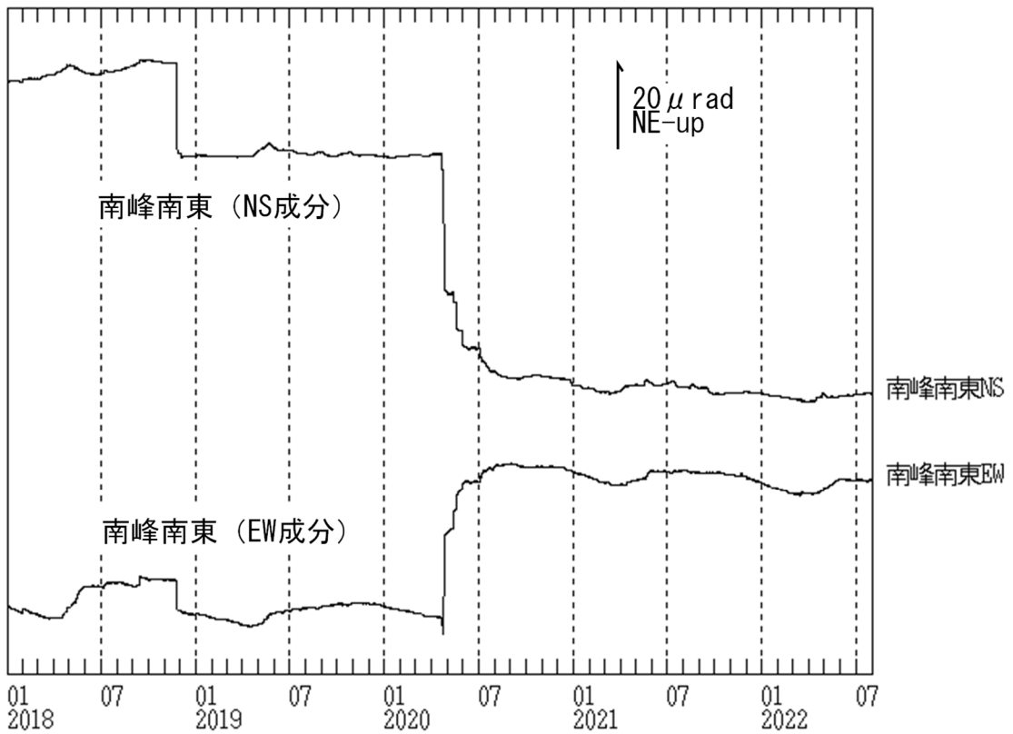
図9 焼岳 南峰南東観測点における傾斜データ（2018年1月1日～2022年7月31日）
