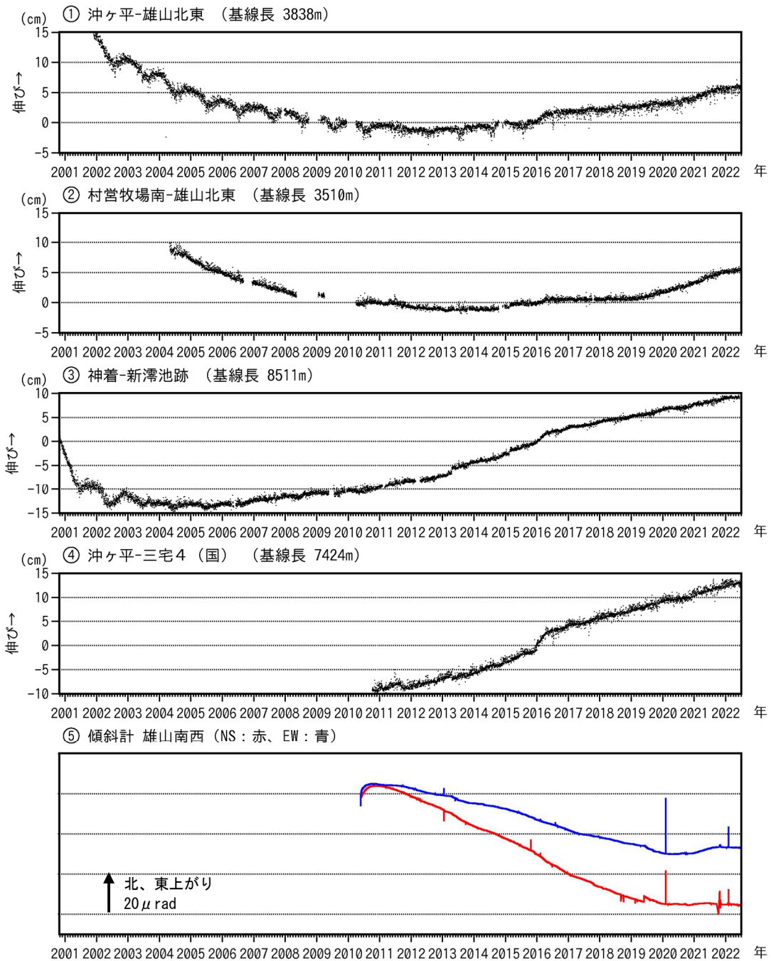
図6 三宅島 GNSS 連続観測及び傾斜計観測結果（2000年10月26日～2022年6月30日）
