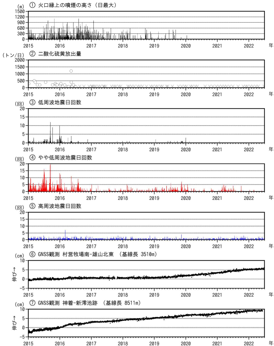
図5 三宅島 短期の火山活動経過図（2015年1月1日～2022年6月30日）
