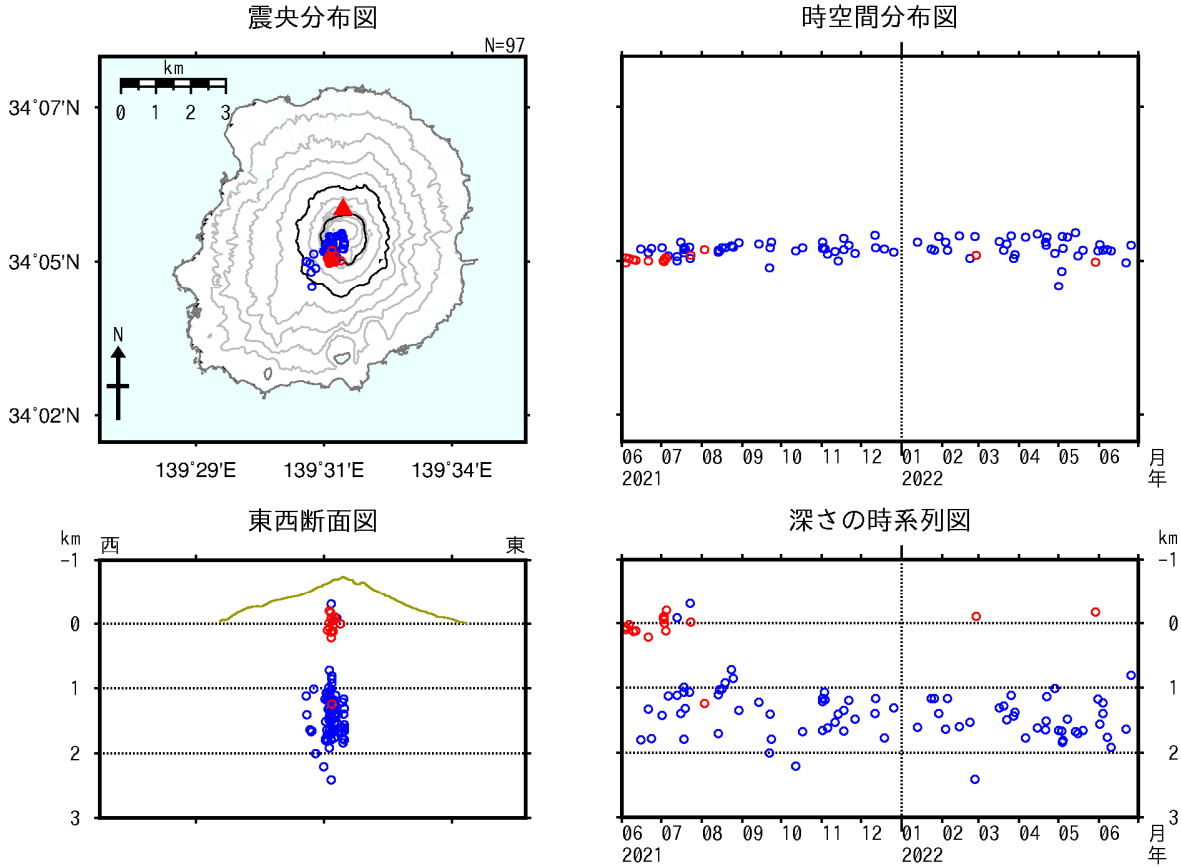
図7 三宅島 震源分布図（2021年6月1日～2022年6月30日）
