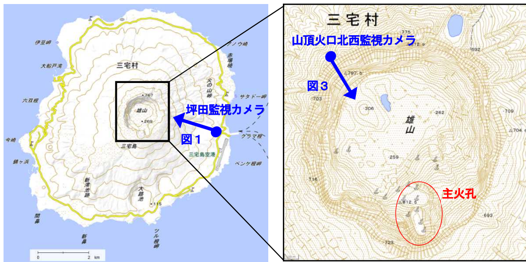
図2 三宅島 監視カメラ（坪田・山頂火口北西）の撮影位置・撮影方向
