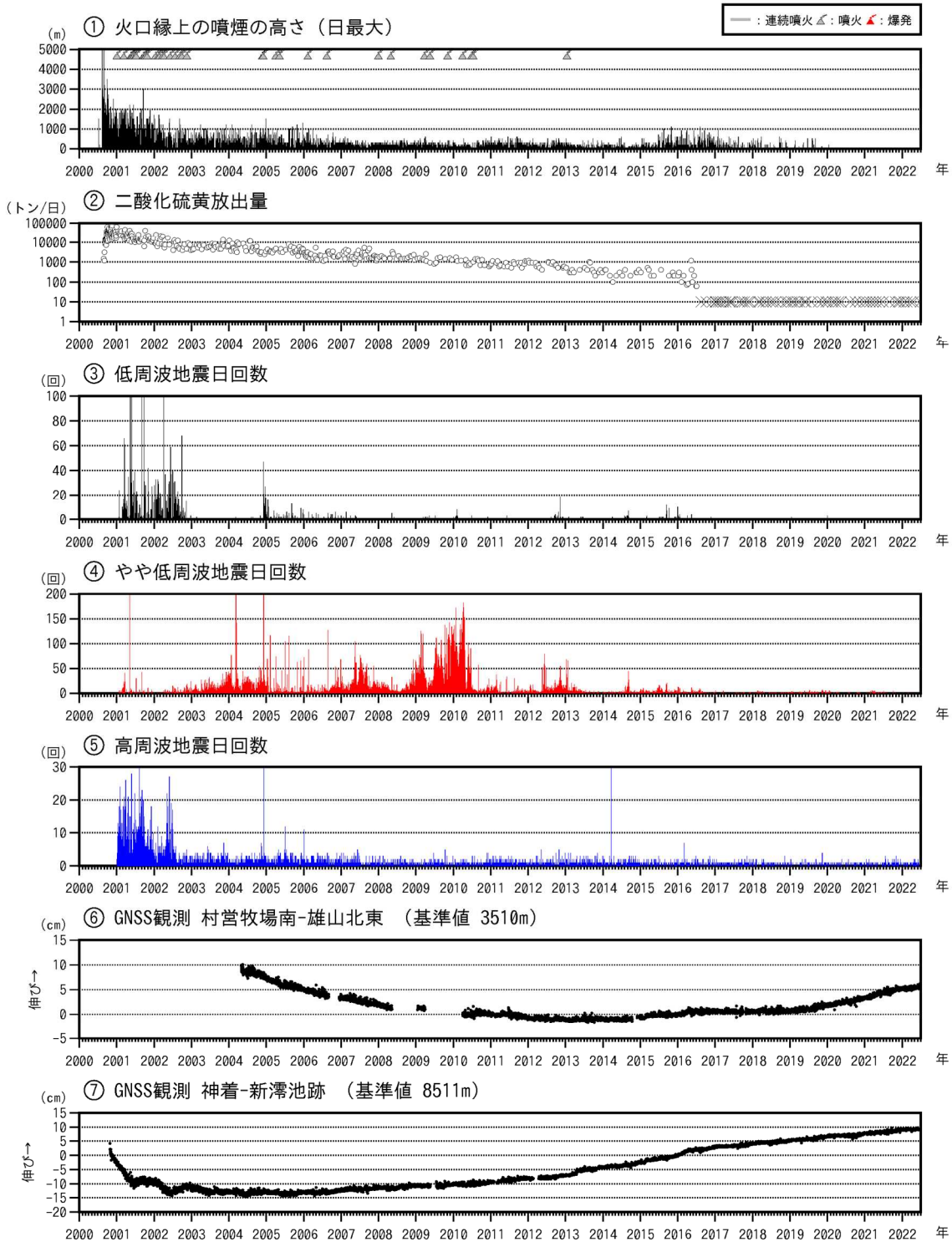
図4 三宅島 長期の火山活動経過図（2000年1月1日～2022年6月30日） ※図4の説明は次ページに掲載。
