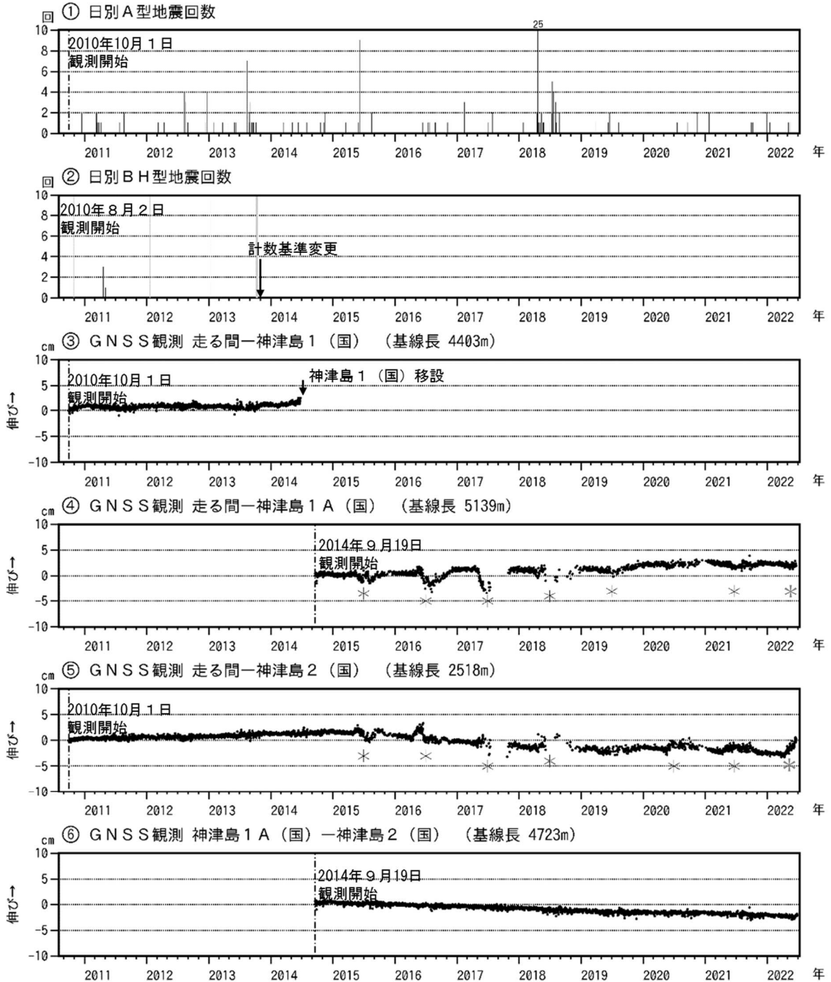
図2 神津島 火山活動経過図(2010年8月2日～2022年6月30日)
