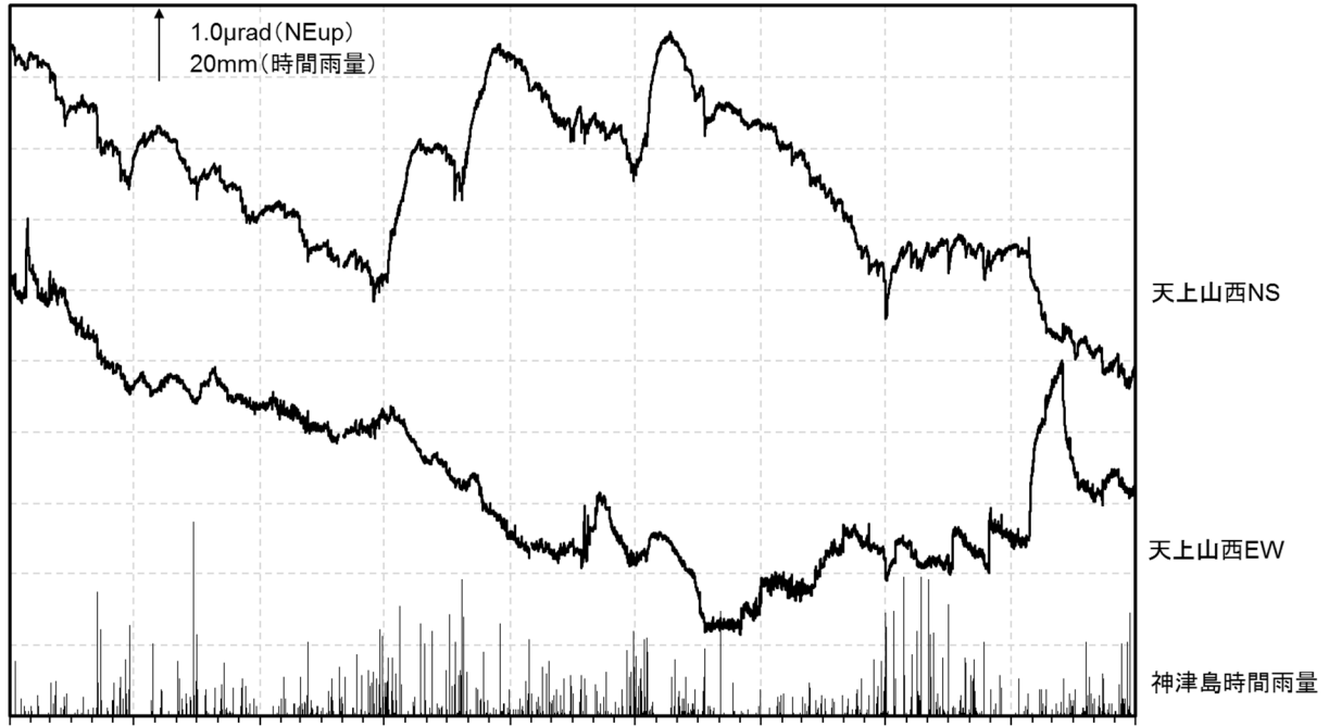
2018/01 2018/07 2019/01 2019/07 2020/01 2020/07 2021/01 2021/07 2022/01 図4 神津島 天上山西観測点の傾斜変動（2018年1月1日～2022年6月30日） 地震等による一部のステップを除去しています。図中の空白部分は欠測を示します。 ・火山活動によるとみられる変動は認められません。
