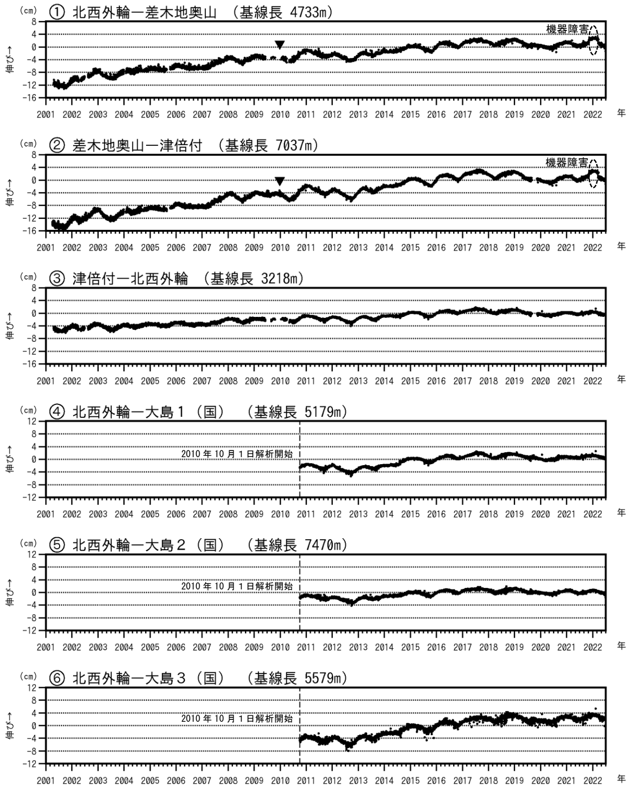
図3-1 伊豆大島 GNSS 連続観測による基線長変化(2001年1月～2022年6月30日)
