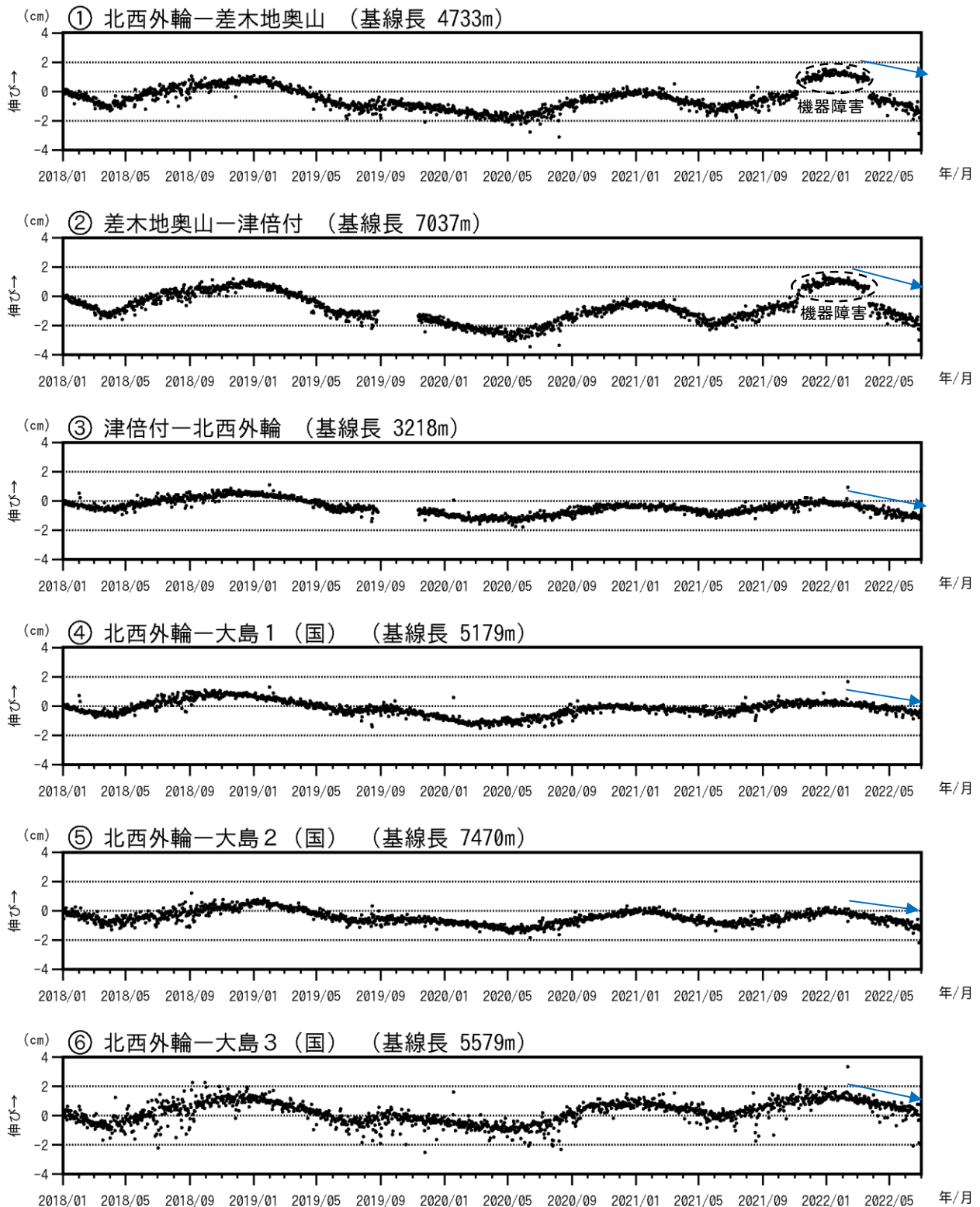
図3-2 伊豆大島 GNSS 連続観測による基線長変化(2018年1月～2022年6月30日)
