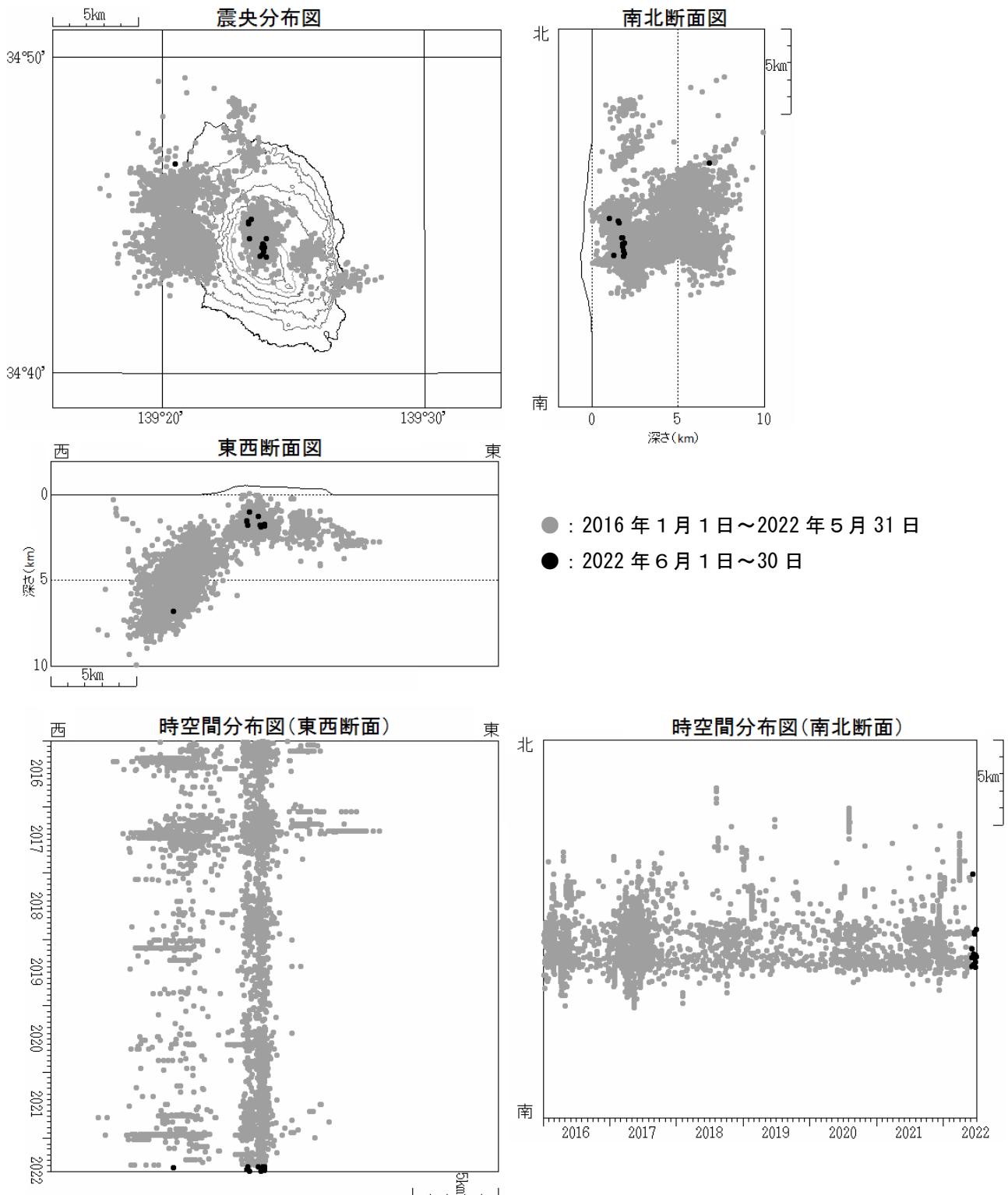
図4 伊豆大島 震源分布図（2016 年 1 月 1 日～2022 年 6 月 30 日）
