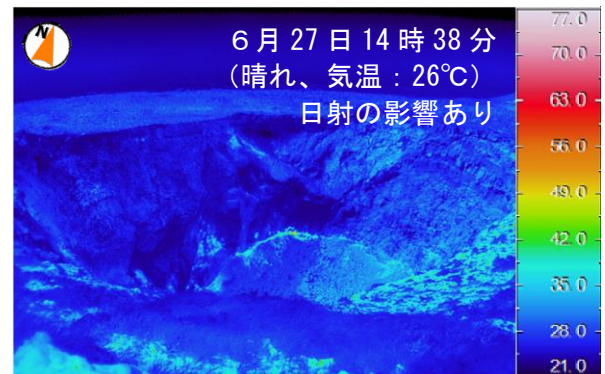
図5 伊豆大島 三原山山頂部及び山頂火口の状況（撮影方向は図8参照）
