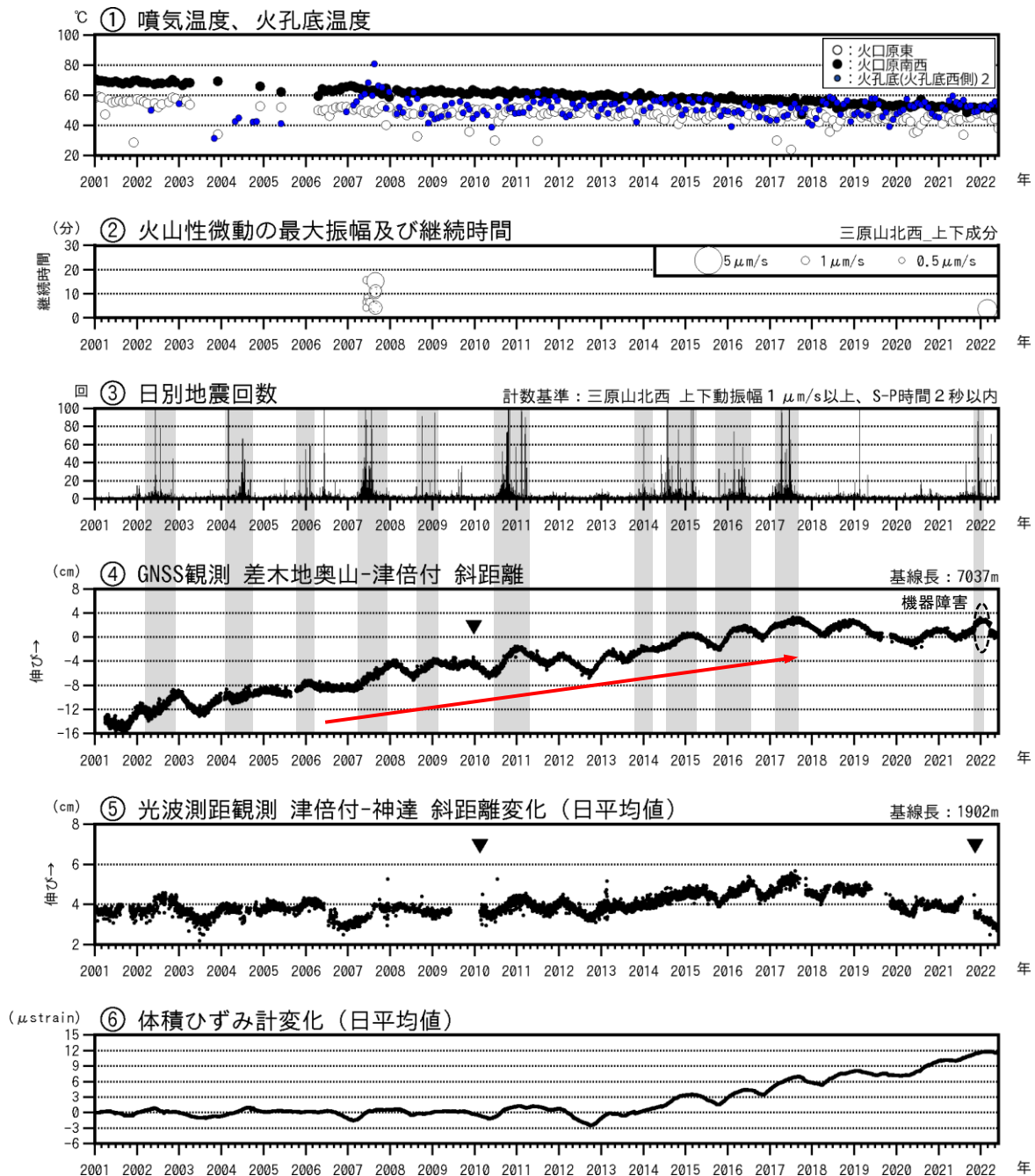
図2 伊豆大島 最近の火山活動経過図（2001年1月～2022年6月30日）
