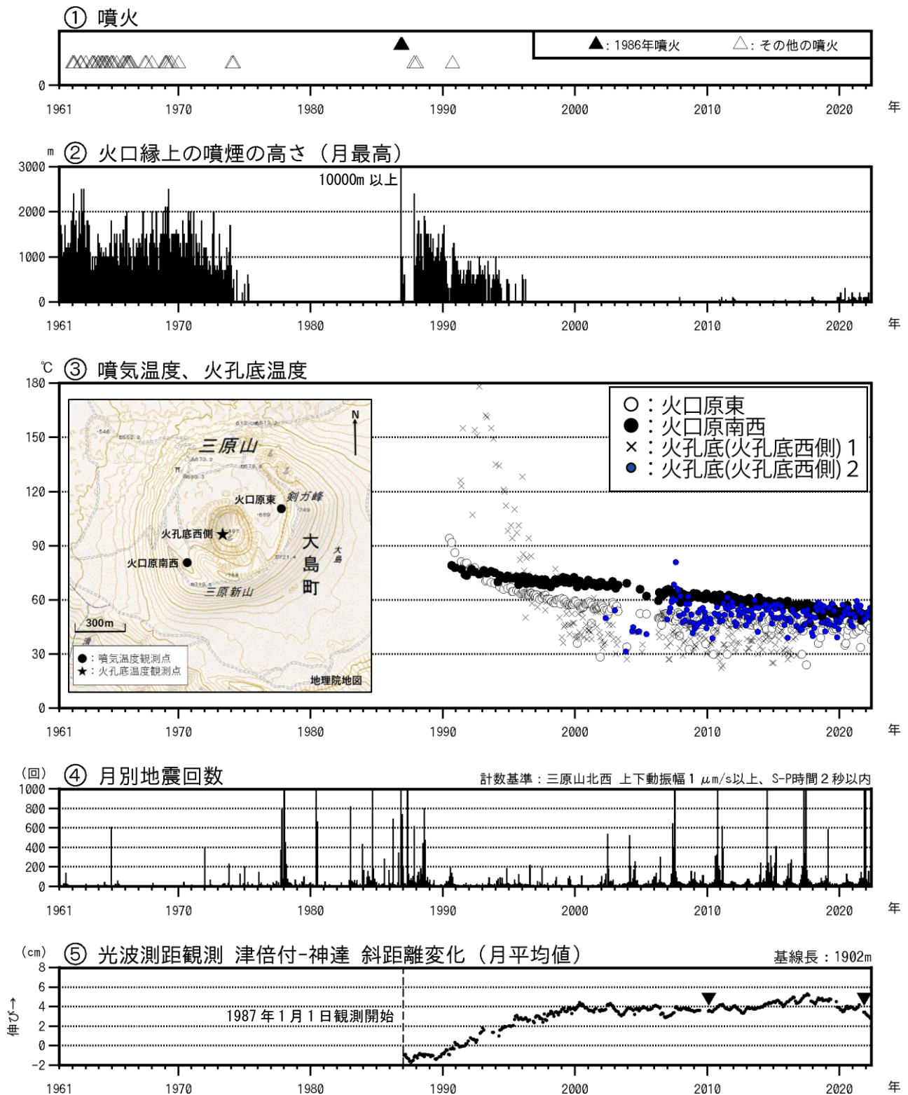
図1 伊豆大島 長期間の火山活動経過図（1961年1月～2022年6月30日）
