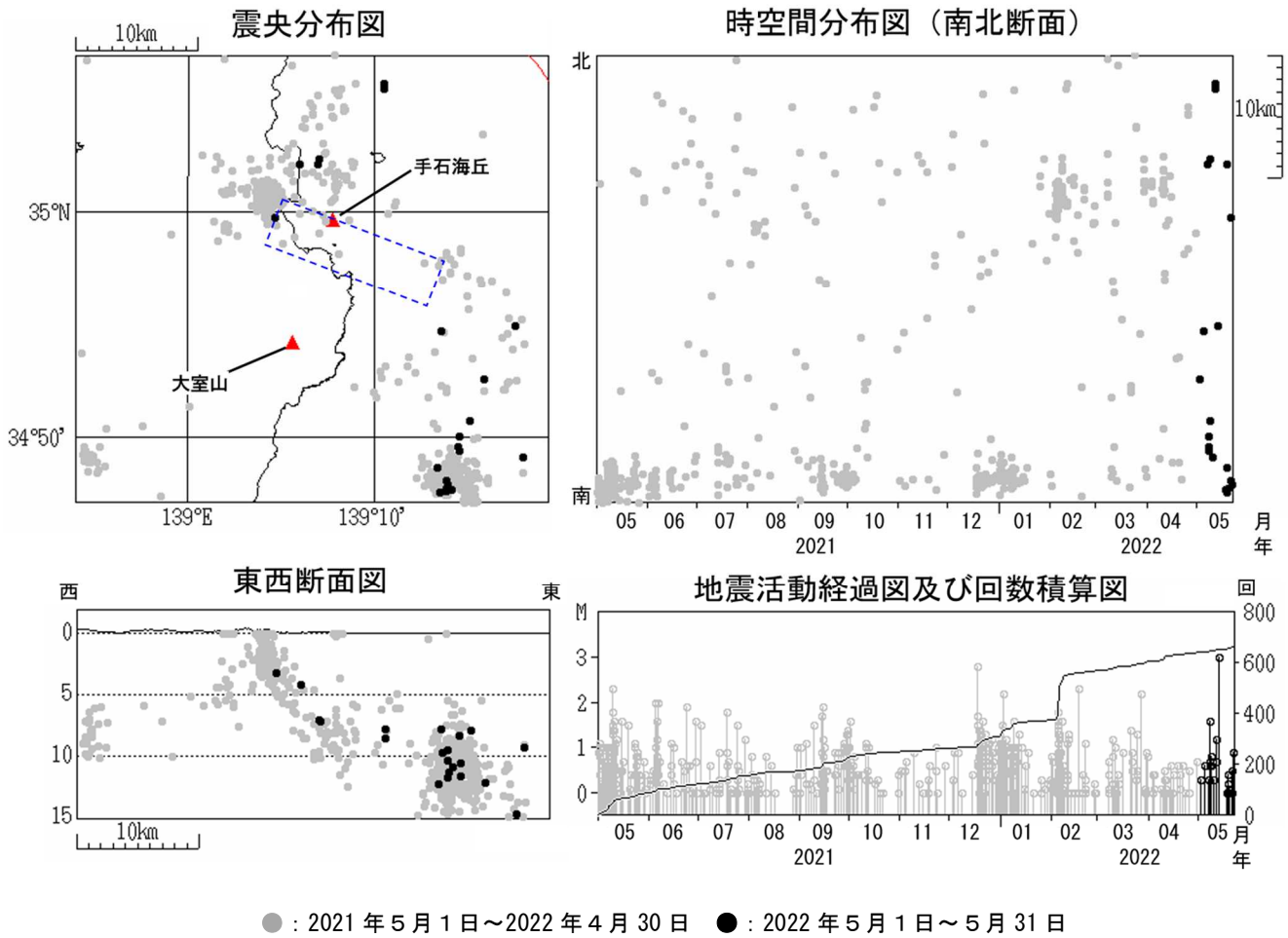
図2 伊豆東部火山群 広域地震観測網による震源分布図（2021年5月1日～2022年5月31日） □の領域は群発地震活動の発生する可能性がある範囲（火口が発生する可能性のある範囲）を示しています。 ( https://www.data.jma.go.jp/vois/data/tokyo/STOCK/level/PDF/level_316.pdf ) 広域地震観測網により震源決定したもので、深さは全て海面以下として決定しています。 M（マグニチュード）は地震の規模を表し、M0.0以上を表示しています。 図中の震源要素は一部暫定値が含まれており、後日変更することがあります。 この図では、関係機関の地震波形を一元的に処理し、地震観測点の標高を考慮する等した手法で得られた震源を用いています。
