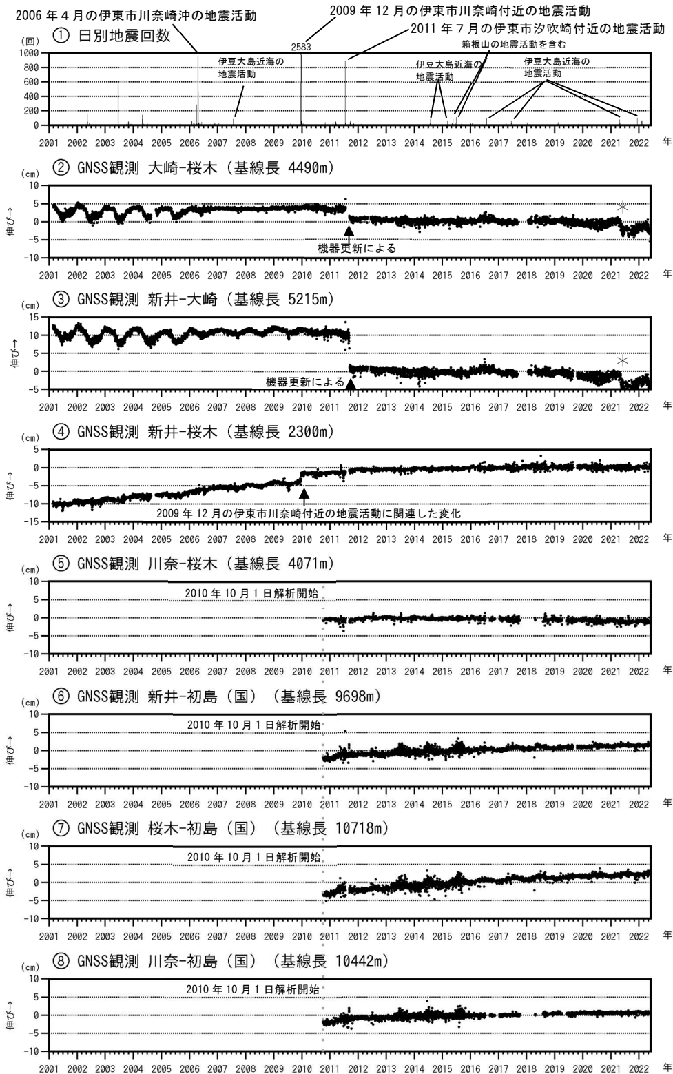
図3 伊豆東部火山群 火山活動経過図（2001年1月1日～2022年5月31日）
