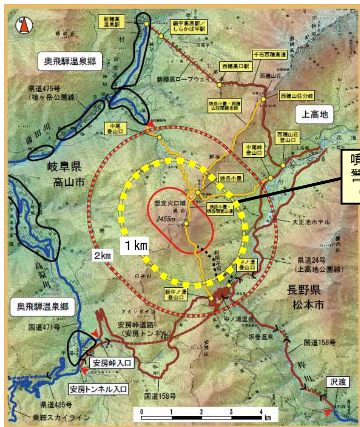
図1 焼岳 噴火警戒レベル2に対応した警戒が必要な範囲（黄破線内）
