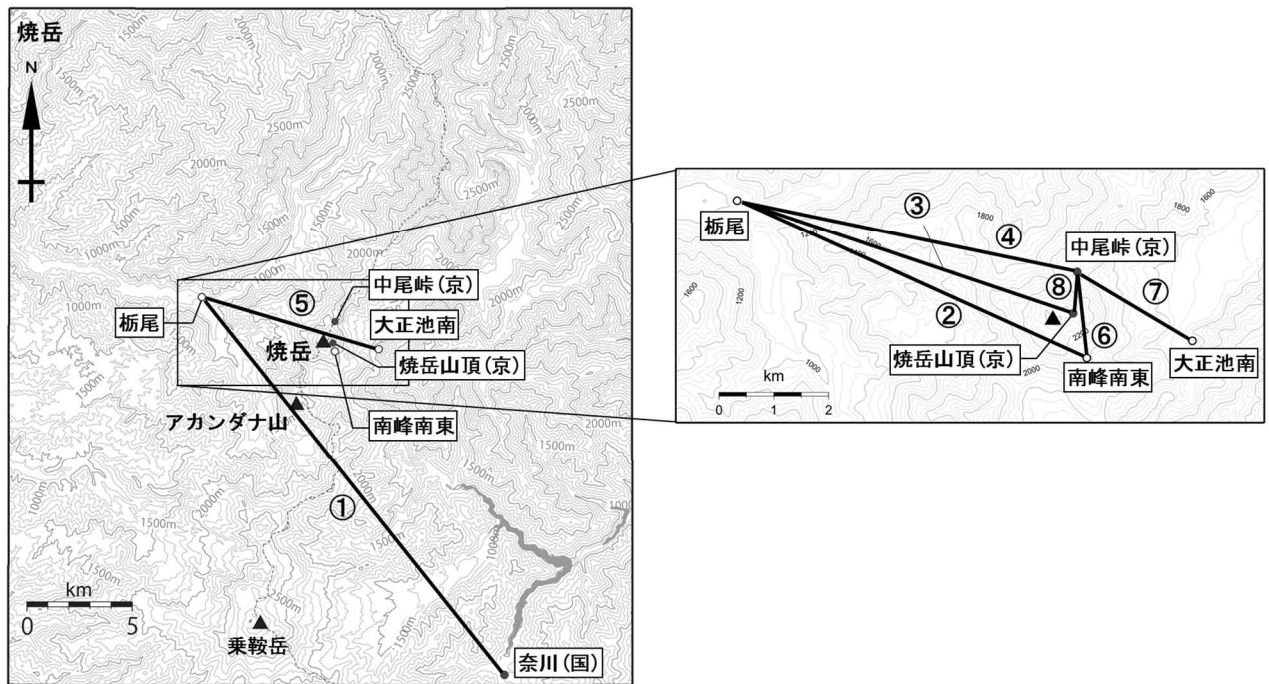
図 12 焼岳 GNSS 連続観測点配置
