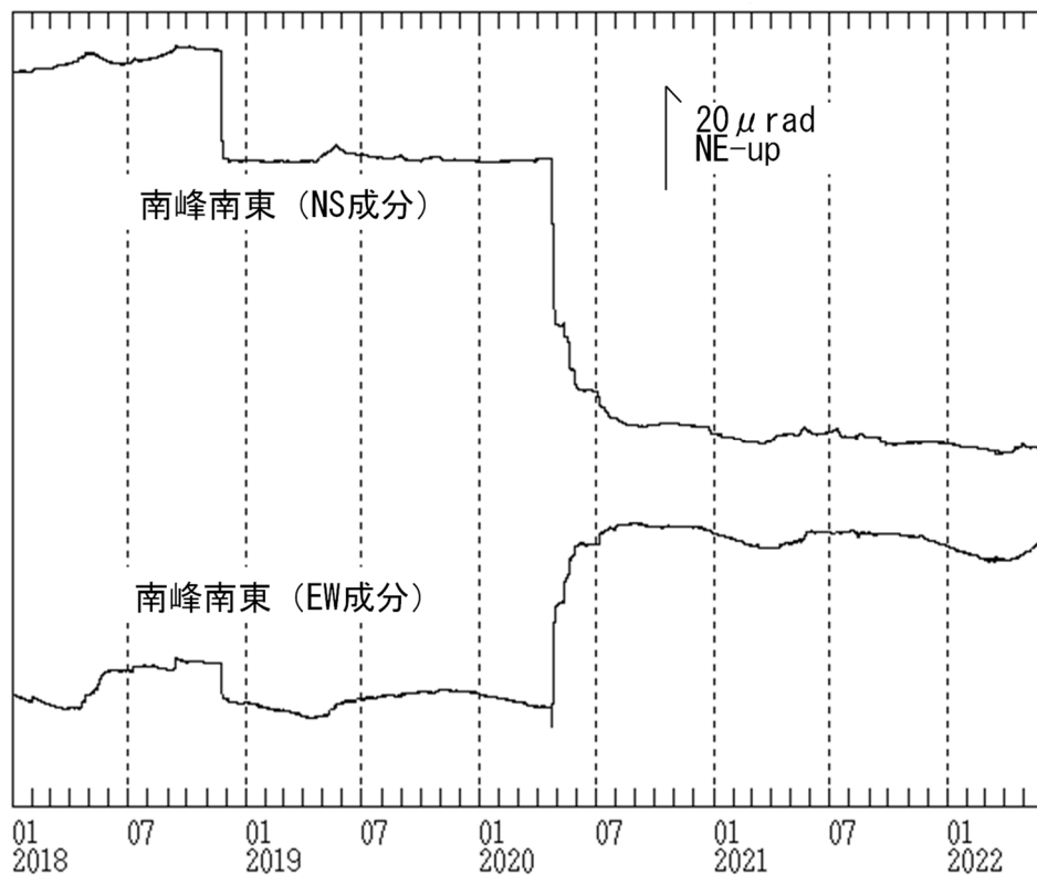
図 13 焼岳 南峰南東観測点における傾斜データ（2018 年 1 月 1 日～2022 年 5 月 31 日）
