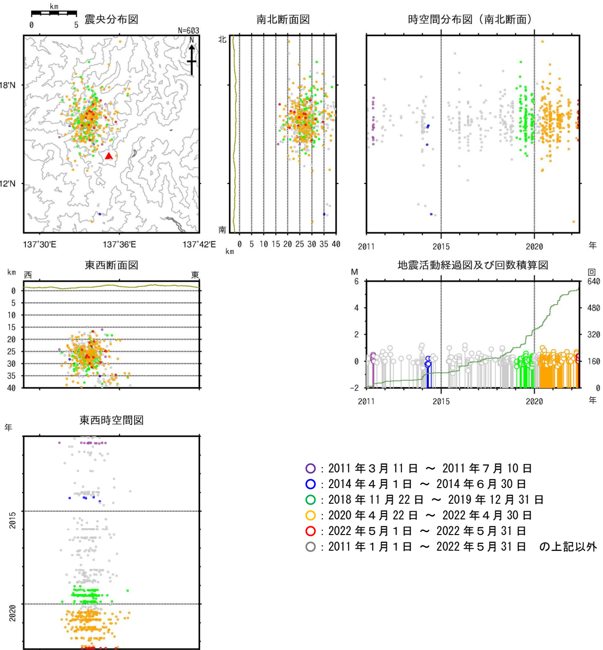
図15 焼岳 広域地震観測網による深部低周波地震の震源分布図（2011年1月1日～2022年5月31日） 広域地震観測網により震源決定したもので、深さは全て海面以下として決定しています。そのため、山頂付近の浅い地震の震源も海面下に決定されています。 M（マグニチュード）は地震の規模を表します。 図中の震源要素は一部暫定値が含まれており、後日変更することがあります。
