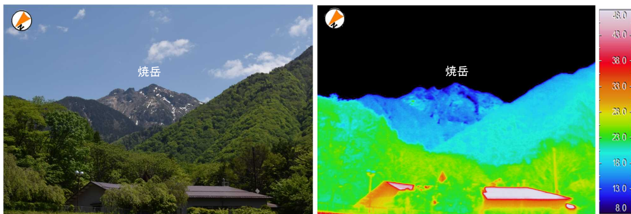
図8 焼岳 焼岳山頂周辺の状況（2022年5月24日13時32分撮影）
