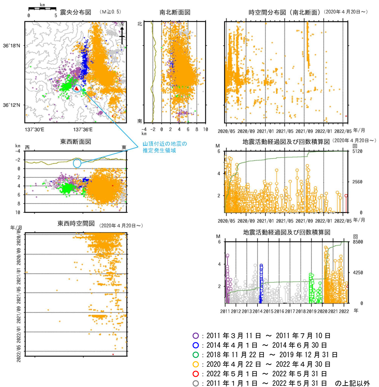
図14 焼岳 広域地震観測網による山体及び周辺の地震活動(2011年1月1日～2022年5月31日)
