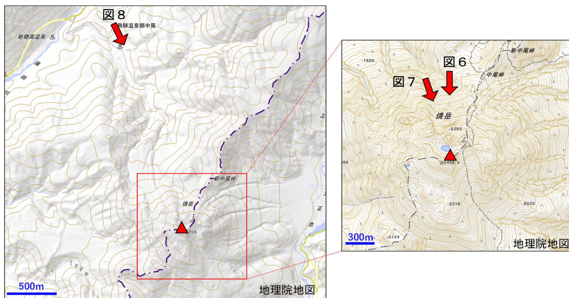
図9 焼岳 図6～8の撮影方向
