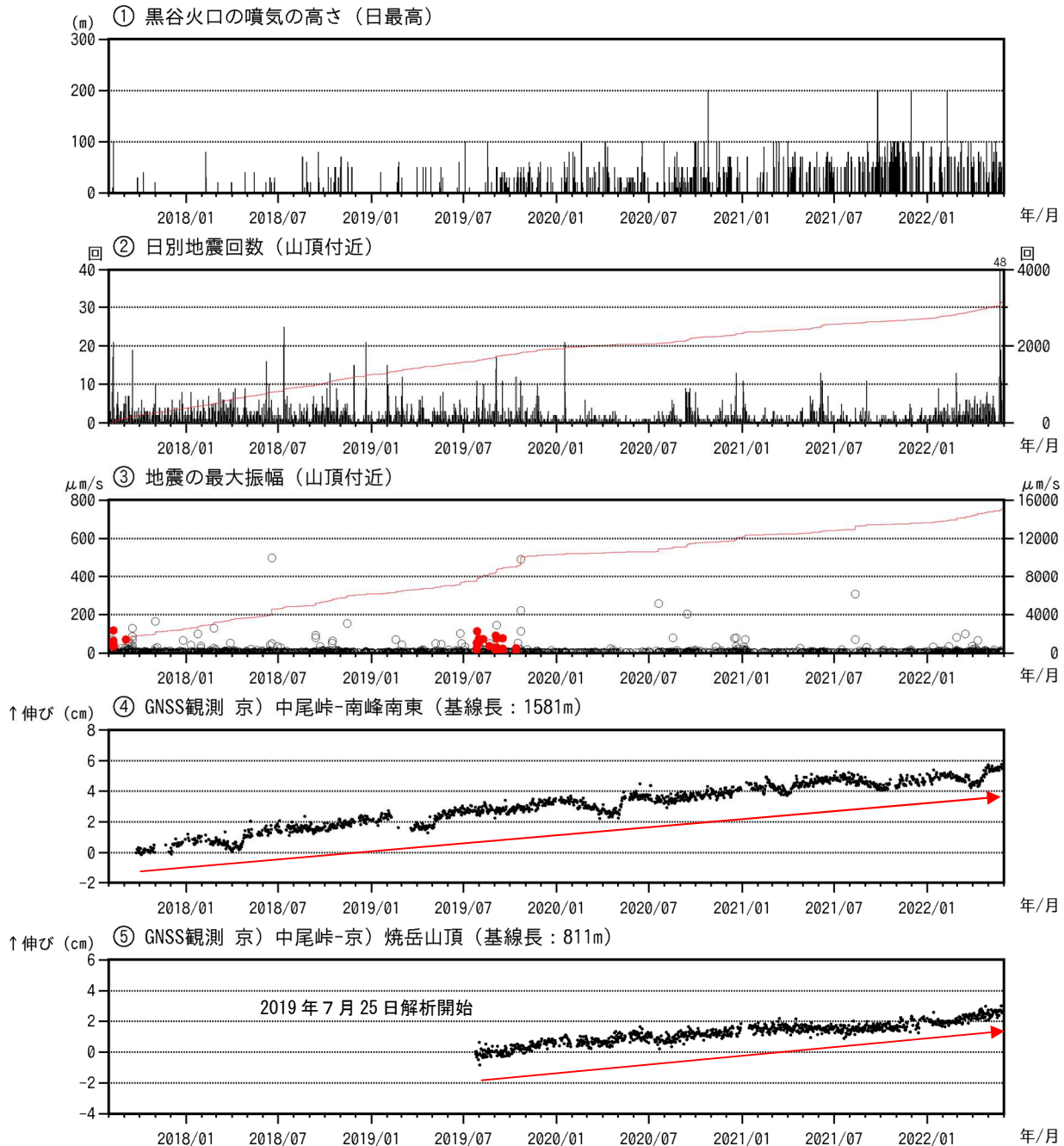
図3 焼岳 火山活動経過図（2017年8月1日～2022年5月31日）
