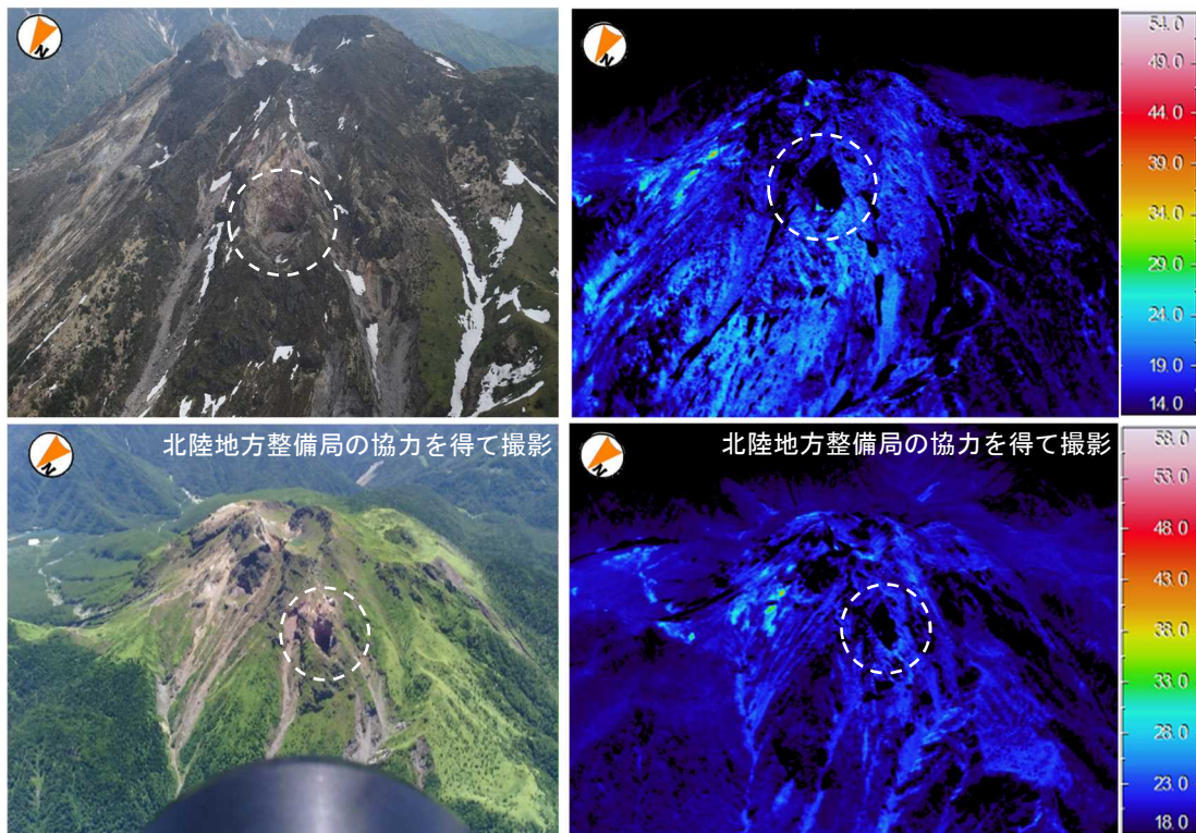
図7 焼岳 焼岳山頂周辺の状況
