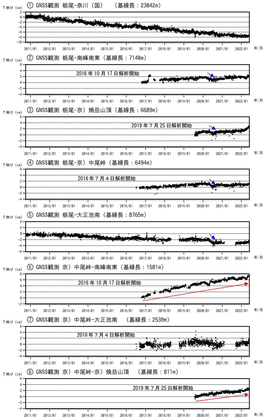
図11 焼岳 GNSS連続観測による基線長変化（2010年10月1日～2022年5月31日）
