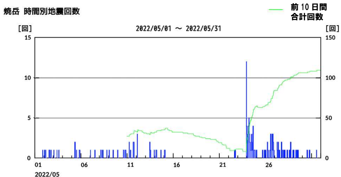
図2 焼岳 山頂付近の時間別地震回数（2022年5月1日～31日）
