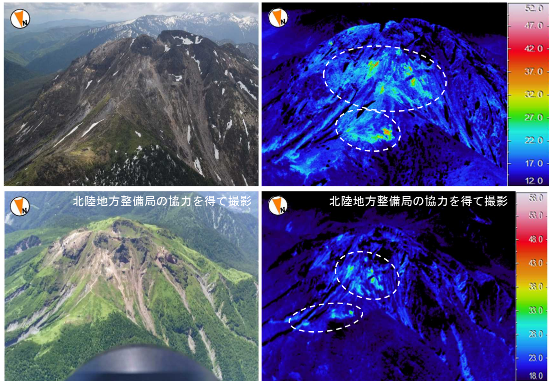
図6 焼岳 焼岳山頂周辺の状況
