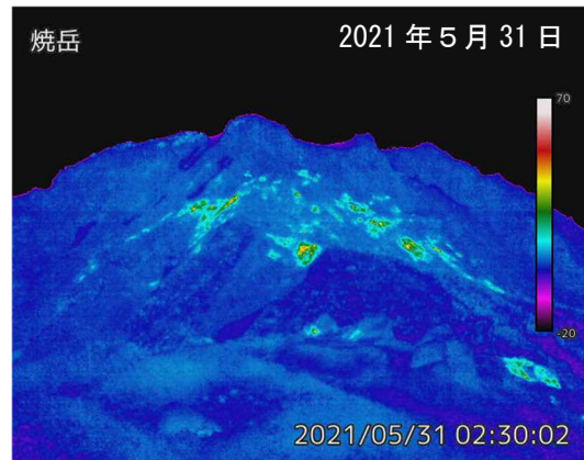
図5 焼岳 中尾峠赤外熱映像カメラによる焼岳の北側斜面の地表面温度分布と可視画像 撮影場所と撮影方向は図15を参照下さい。
