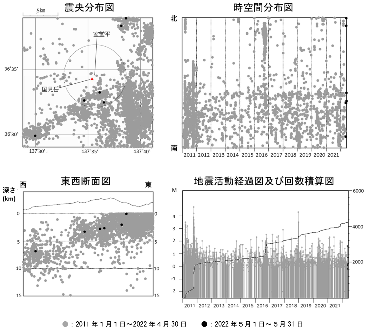
図2 弥陀ヶ原 広域地震観測網による山体・周辺の地震活動（2011 年 1 月 1 日～2022 年 5 月 31 日） 震央分布図中の円は弥陀ヶ原の計数対象地震（室堂平で S-P 時間 1 秒以内）のおよその範囲を示しています。 広域地震観測網により震源決定したもので、深さは全て海面以下として決定しています。 図中の震源要素は一部暫定値が含まれており、後日変更することがあります。 この図では、関係機関の地震波形を一元的に処理し、地震観測点の標高を考慮する等した手法で得られた震源を用いています（ただし、2020 年 8 月以前の地震については火山活動評価のための参考震源です）。
