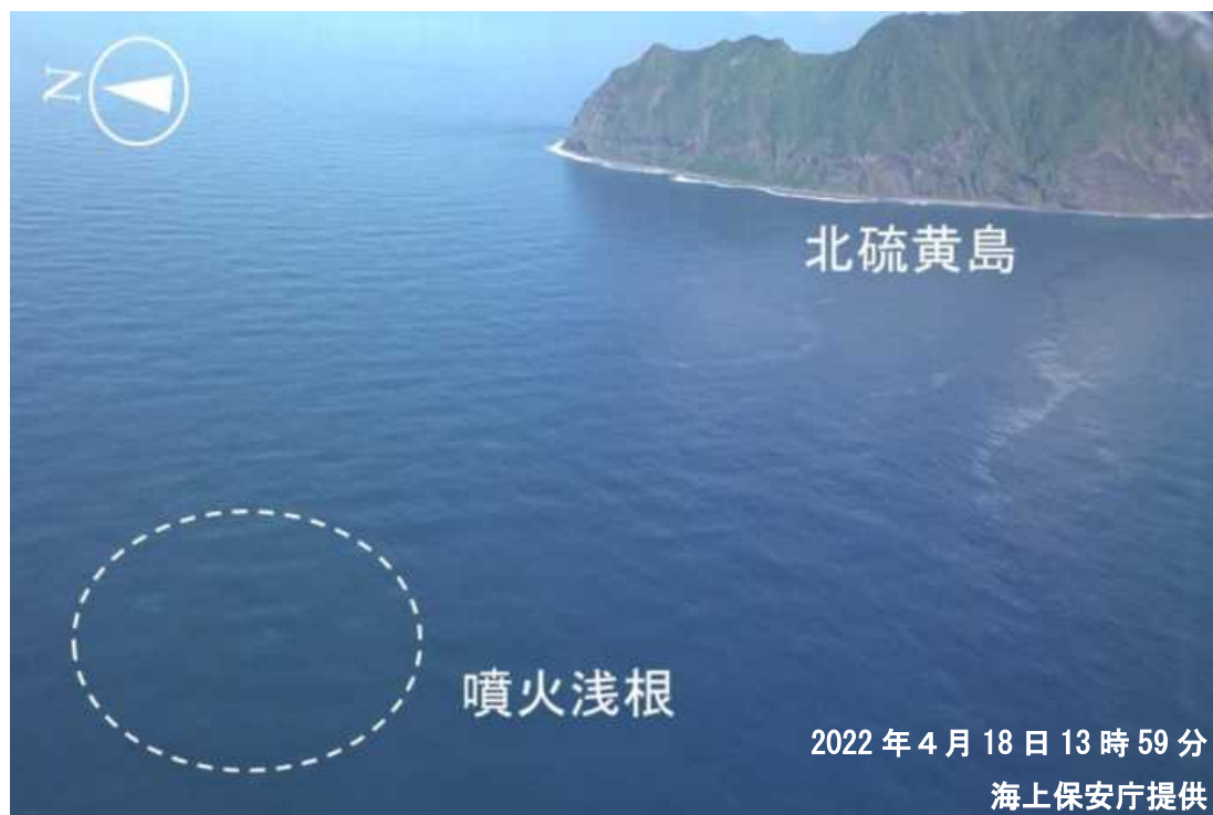
図2 噴火浅根 18日の状況
