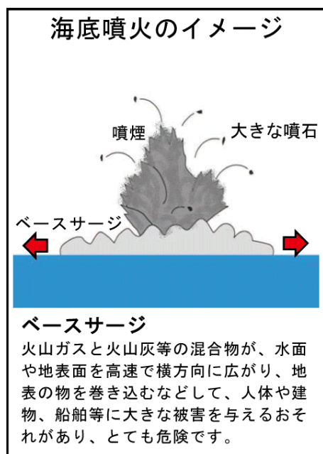
図5 海底噴火による影響のイメージ
