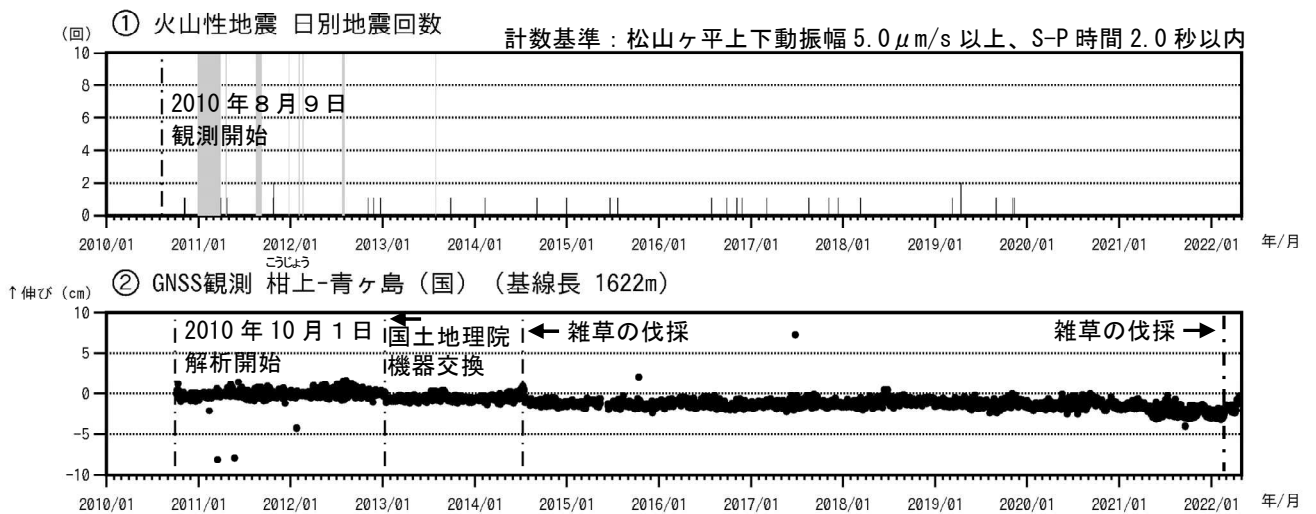
図3 青ヶ島 火山活動経過図（2010年8月9日～2022年4月30日）
