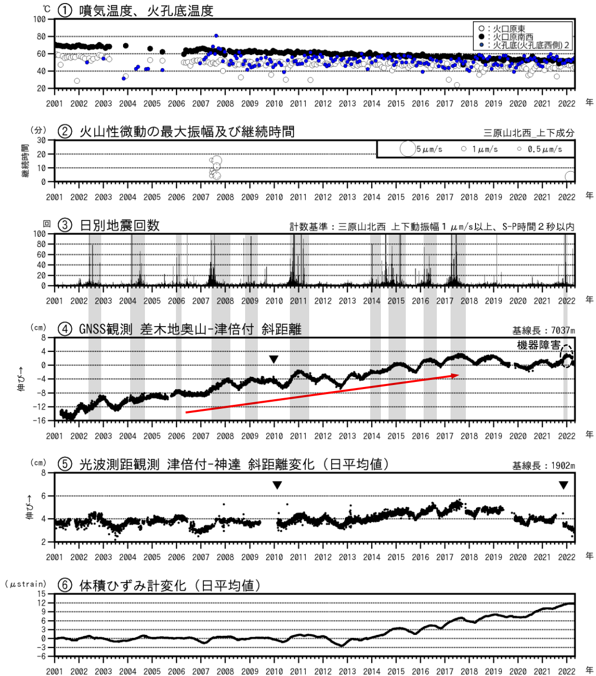
図2 伊豆大島 最近の火山活動経過図（2001年1月～2022年4月30日）
