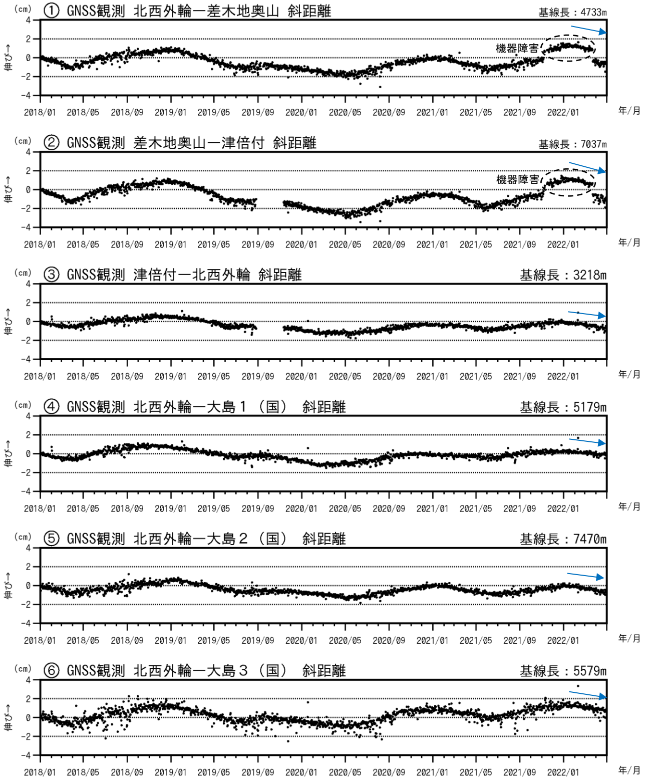
図3-2 伊豆大島 GNSS連続観測による基線長変化(2018年1月～2022年4月30日)
