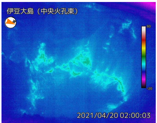
2021年4月20日 中央火孔東監視カメラによる
