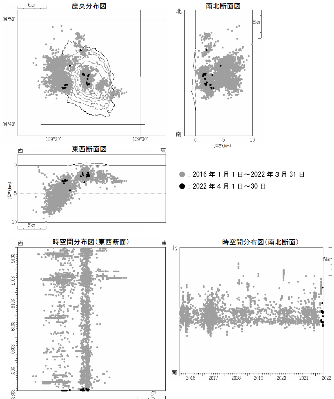
図4 伊豆大島 震源分布図（2016年1月1日～2022年4月30日）
