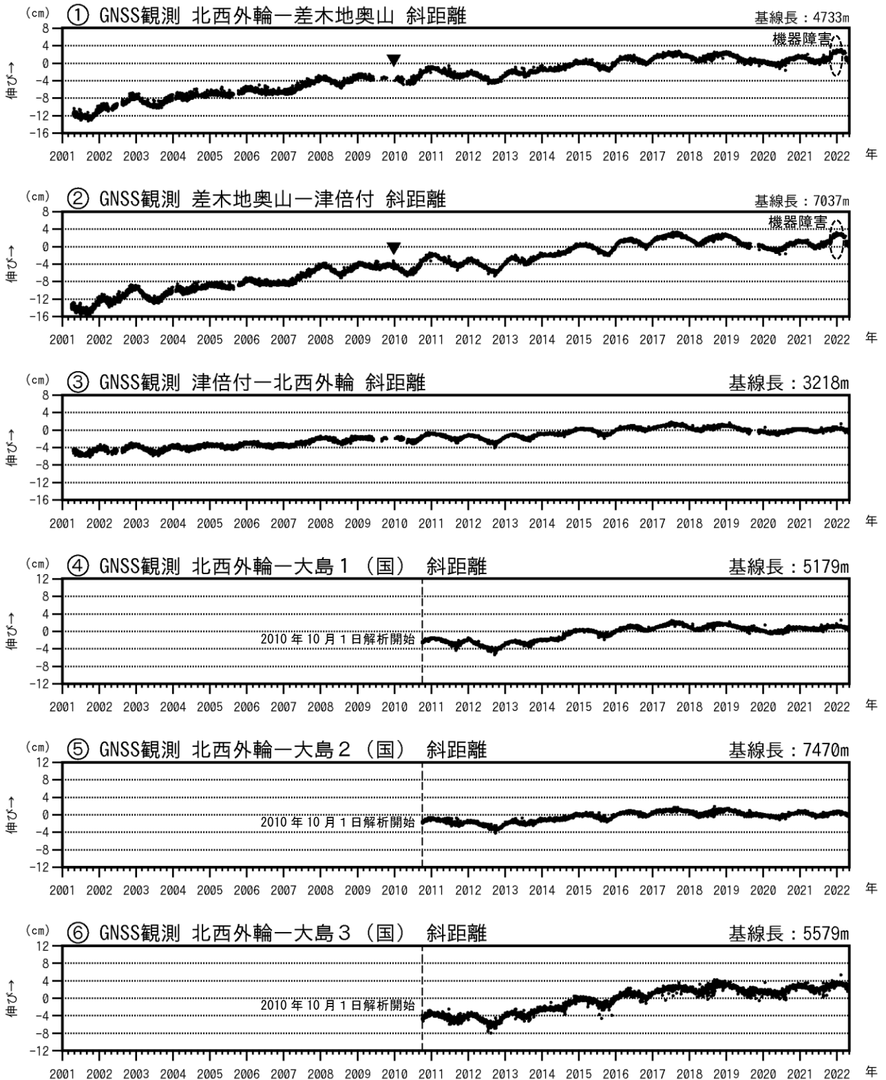
図3-1 伊豆大島 GNSS 連続観測による基線長変化(2001年1月～2022年4月30日)
