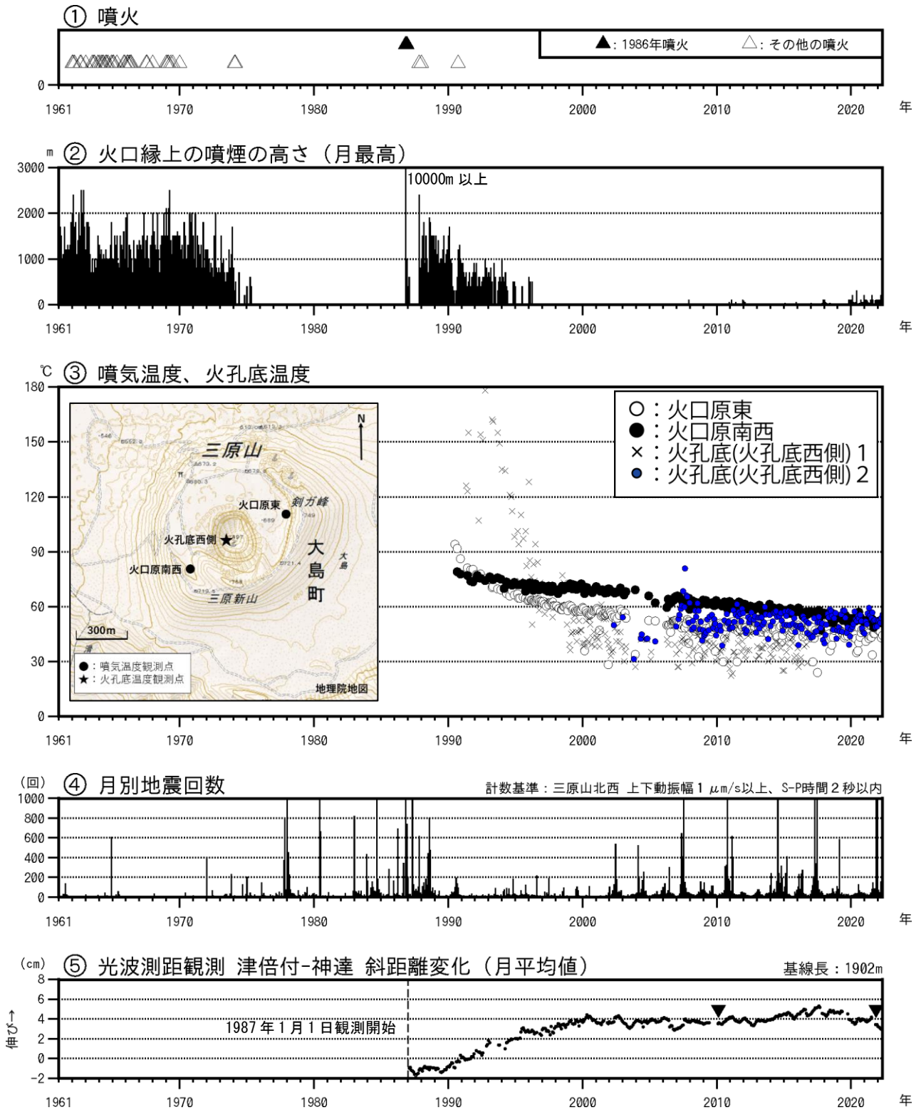
図1 伊豆大島 長期間の火山活動経過図（1961年1月～2022年4月30日）
