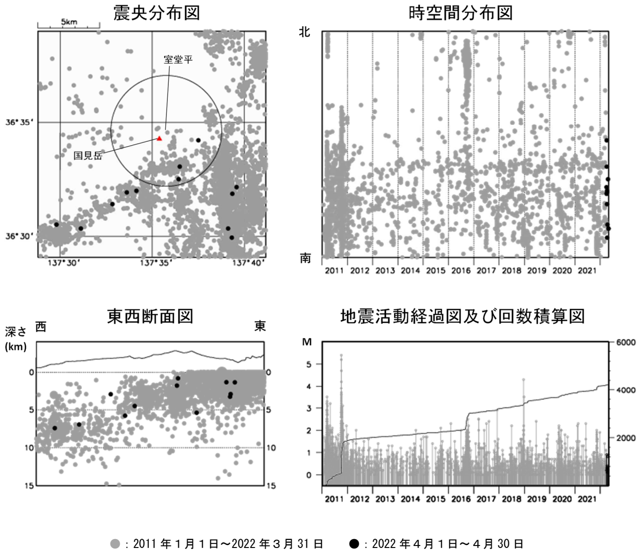
図2 弥陀ヶ原 広域地震観測網による山体・周辺の地震活動（2011 年 1 月 1 日～2022 年 4 月 30 日） 震央分布図中の円は弥陀ヶ原の計数対象地震（室堂平で S-P 時間 1 秒以内）のおよその範囲を示しています。 広域地震観測網により震源決定したもので、深さは全て海面以下として決定しています。 図中の震源要素は一部暫定値が含まれており、後日変更することがあります。 この図では、関係機関の地震波形を一元的に処理し、地震観測点の標高を考慮する等した手法で得られた震源を用いています（ただし、2020 年 8 月以前の地震については火山活動評価のための参考震源です）。
