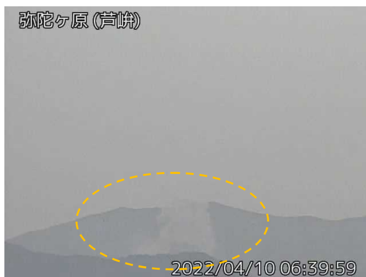
図1 弥陀ヶ原 地獄谷からの噴気の状況（橙丸）（4月10日、芦峠監視カメラによる）
