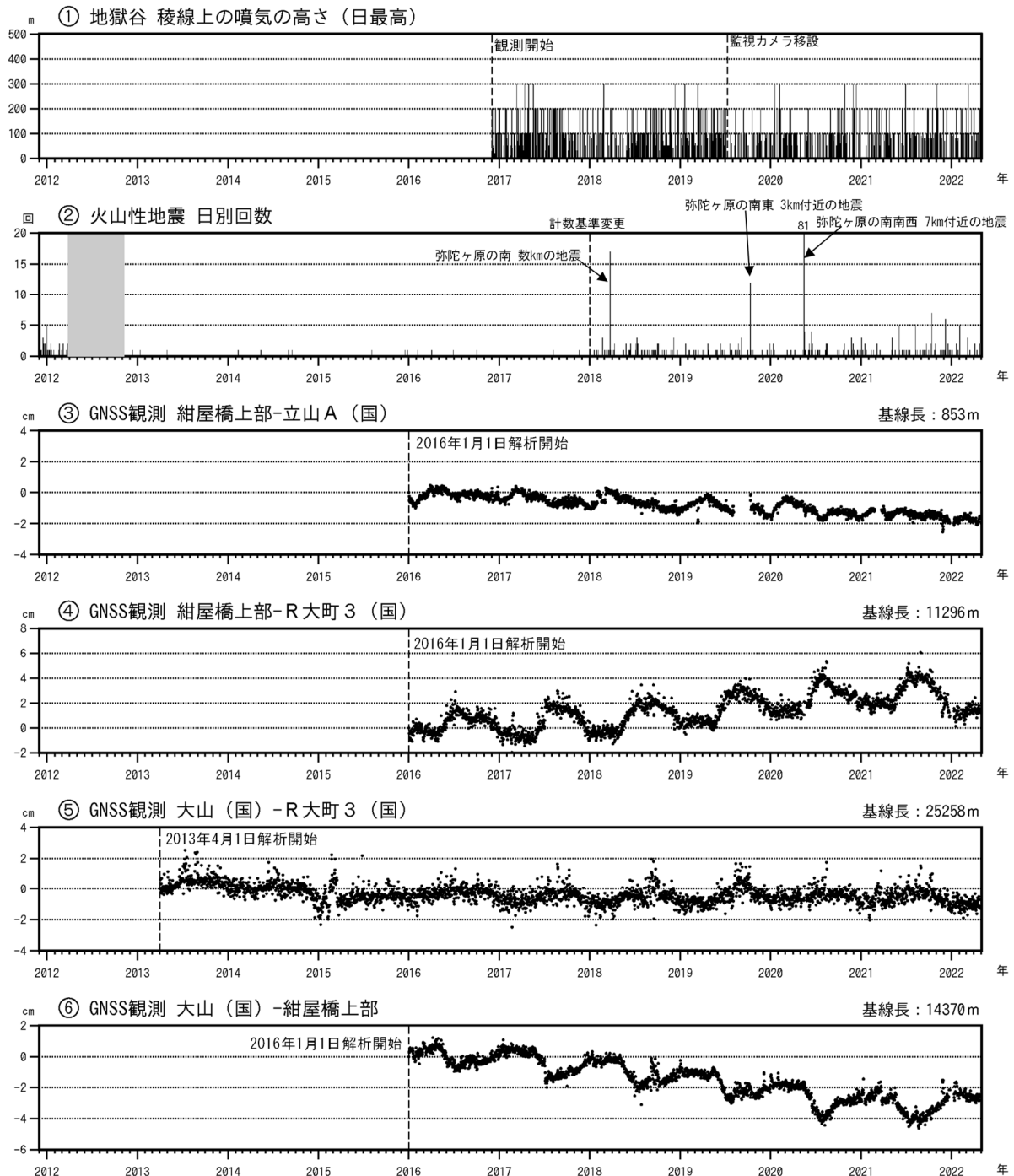
図3 弥陀ヶ原 火山活動経過図（2011年12月1日～2022年4月30日）
