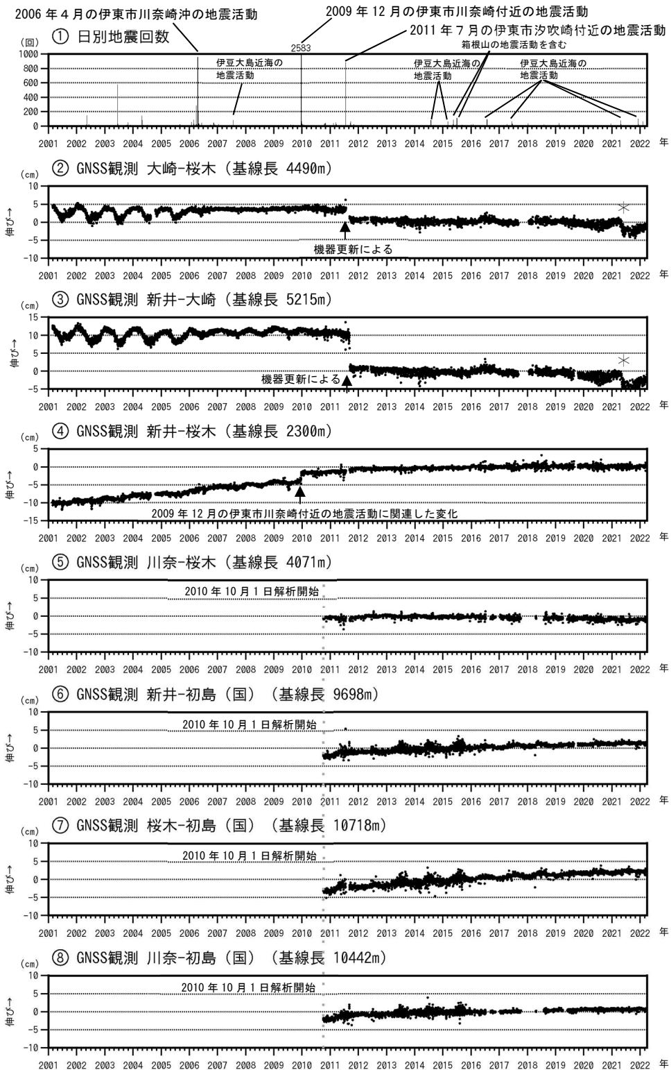
図3 伊豆東部火山群 火山活動経過図（2001年1月1日～2022年3月31日）
