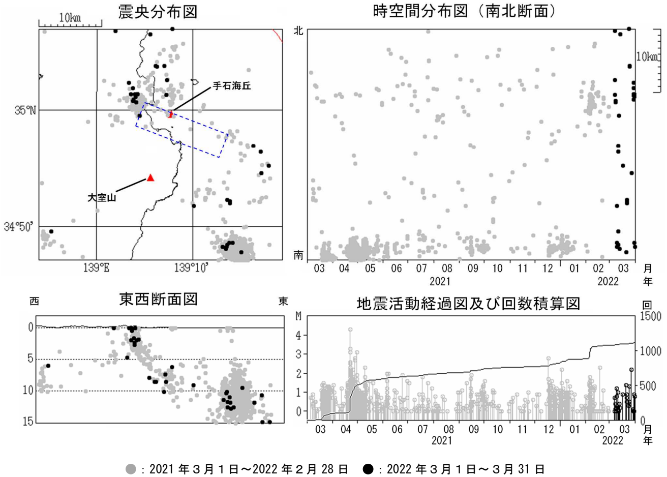
図2 伊豆東部火山群 広域地震観測網による震源分布図（2021年3月1日～2022年3月31日） □の領域は群発地震活動の発生する可能性がある範囲（火口が発生する可能性のある範囲）を示しています。 ( https://www.data.jma.go.jp/vois/data/tokyo/STOCK/level/PDF/level_316.pdf ) 広域地震観測網により震源決定したもので、深さは全て海面以下として決定しています。 M（マグニチュード）は地震の規模を表し、M0.0以上を表示しています。 図中の震源要素は一部暫定値が含まれており、後日変更することがあります。 この図では、関係機関の地震波形を一元的に処理し、地震観測点の標高を考慮する等した手法で得られた震源を用いています。
