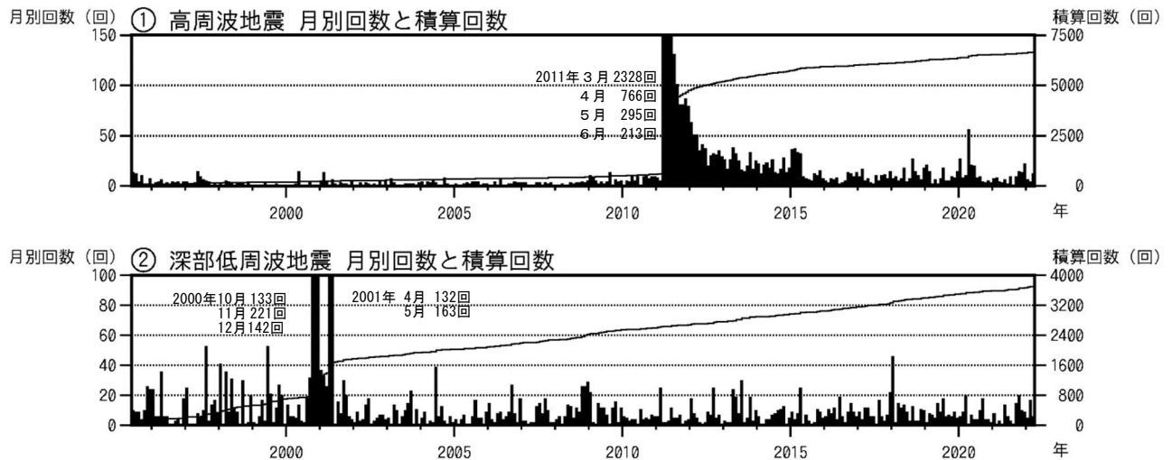
図2 富士山 月別地震回数（1995年6月1日～2022年3月31日）
