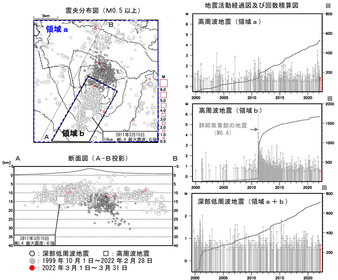
図3 富士山 広域地震観測網による山体及び周辺の地震活動（1999年10月1日～2022年3月31日）
