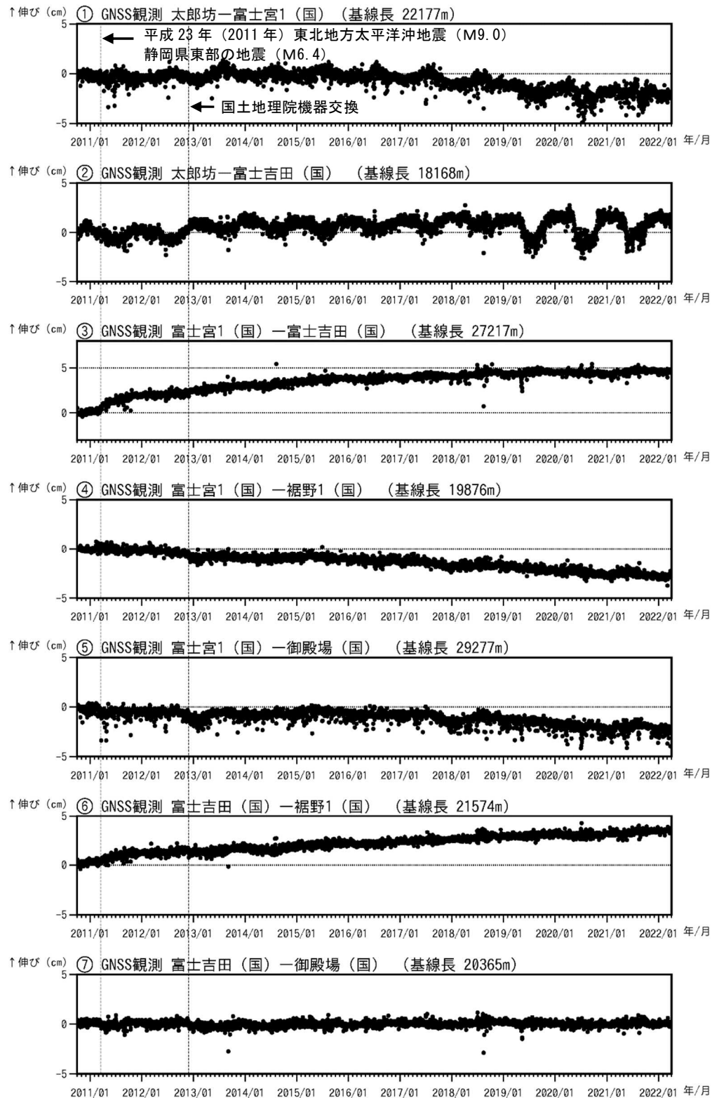
図4 富士山 GNSS 連続観測による基線長変化 (2010 年 10 月 1 日～2022 年 3 月 31 日) (国): 国土地理院 「平成 23 年 (2011 年) 東北地方太平洋沖地震」及び 2011 年 3 月 15 日に発生した静岡県東部の地震 (M 6.4) によるステップ状の変化を補正しています。 ①～⑦は図5の GNSS 基線①～⑦に対応しています。
