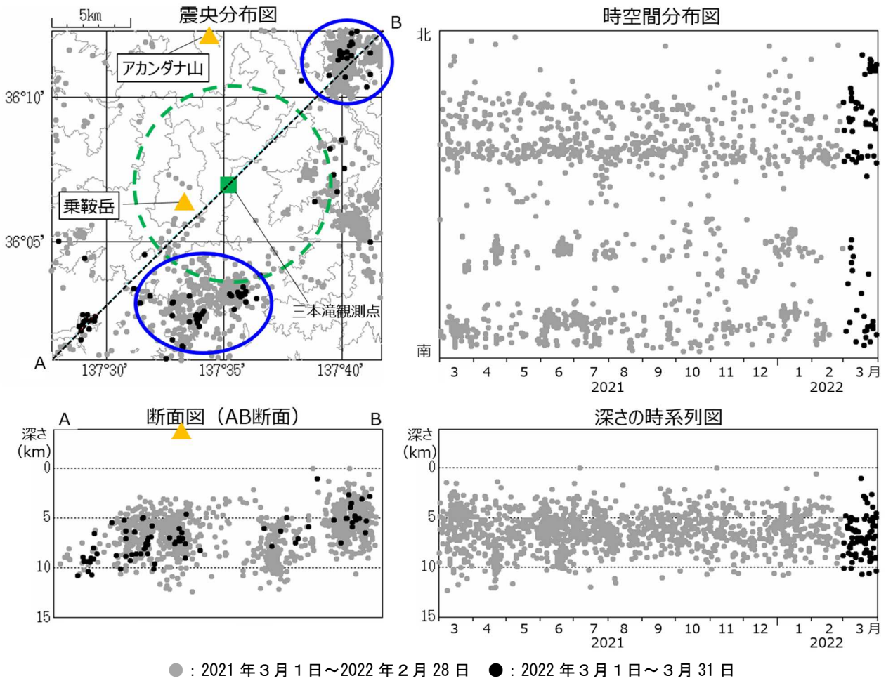
図3 乗鞍岳 広域地震観測網による山体・周辺の地震活動(2021年3月1日～2022年3月31日) 広域地震観測網により震源決定したもので、深さは全て海面以下として決定しています。図中の震源要素は一部暫定値が含まれており、後日変更することがあります。 この図では、関係機関の地震波形を一元的に処理し、地震観測点の標高を考慮する等した手法で得られた震源を用いています。 震央分布図中の緑破線円は、図2①で計数される地震のおおよその範囲を示します。
