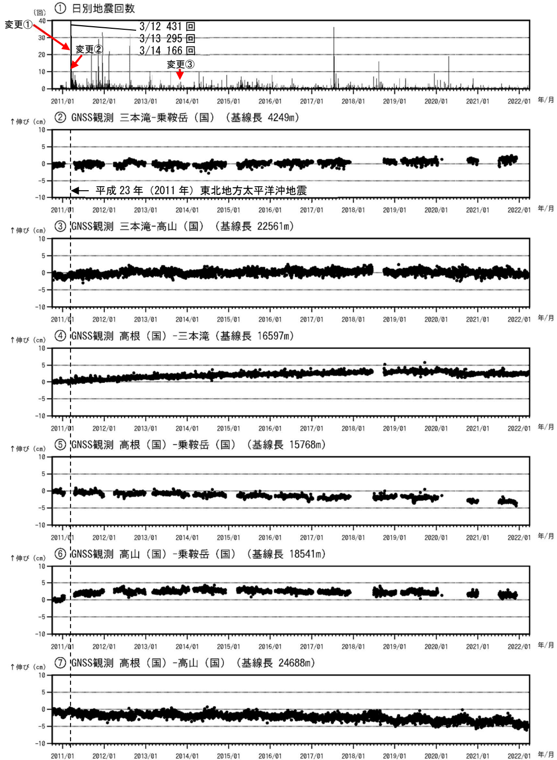
図2 乗鞍岳 火山活動経過図（2010年10月1日～2022年3月31日）
