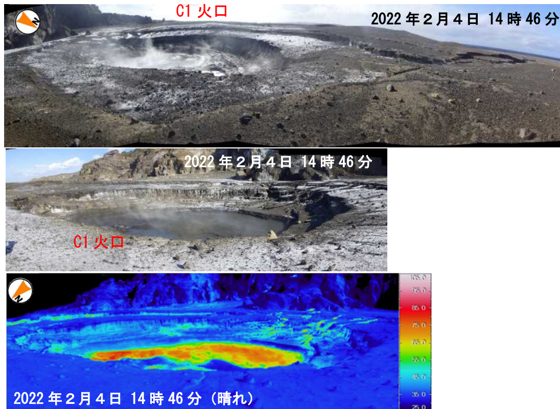
図 11 硫黄島 漂流木海岸C 1火口の様子
