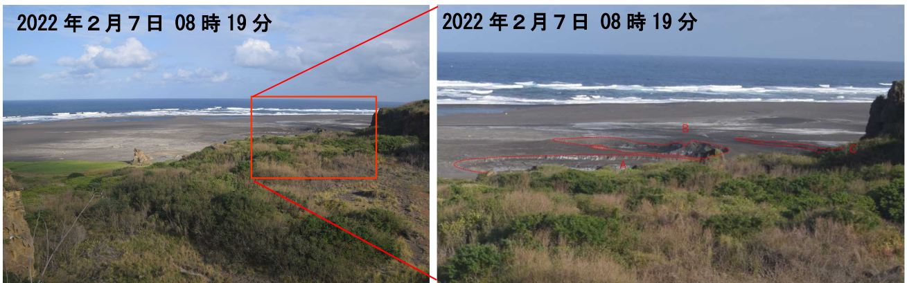
図8 硫黄島 漂流木海岸の状況
