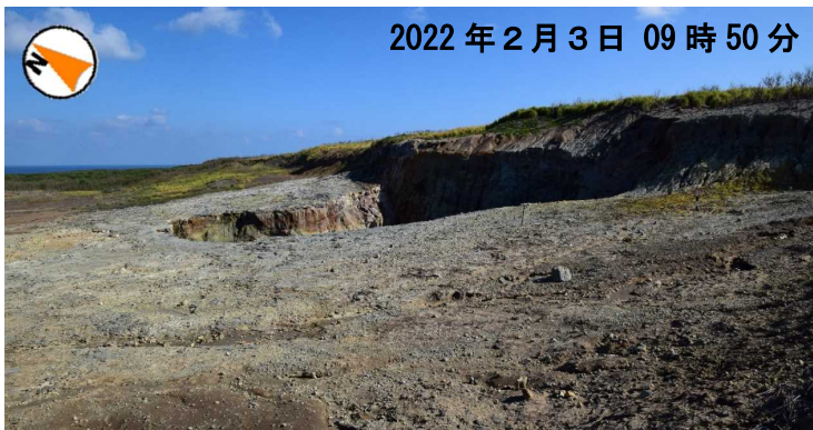
図12 硫黄島 阿蘇台陥没孔の様子
