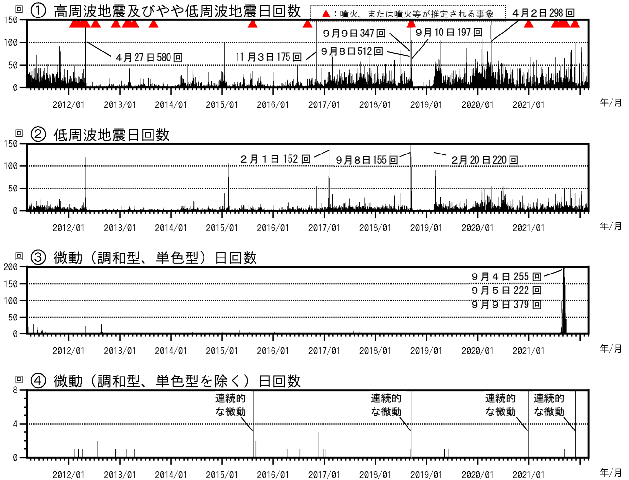
図4 硫黄島 長期火山活動経過図（2011年3月8日～2022年2月28日）
