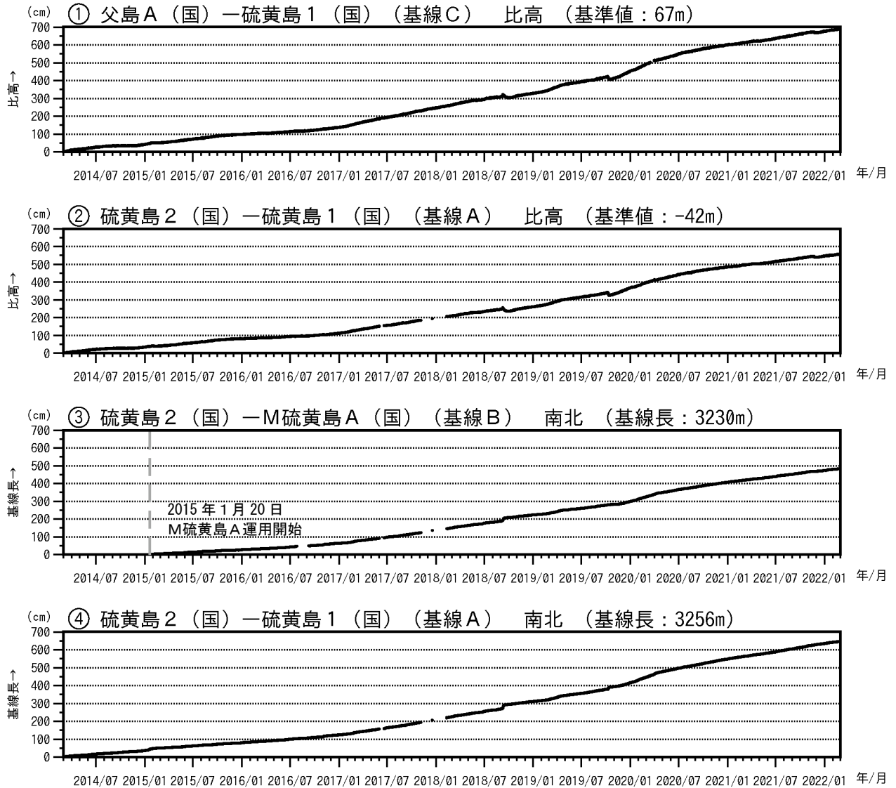
図5 硫黄島 GNSS 連続観測結果（2014年3月1日～2022年2月28日）
