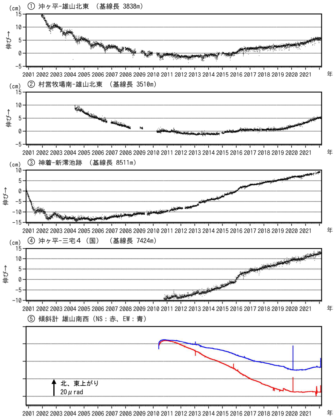
図8 三宅島 GNSS 連続観測及び傾斜計観測結果（2000年10月26日～2022年2月28日）
