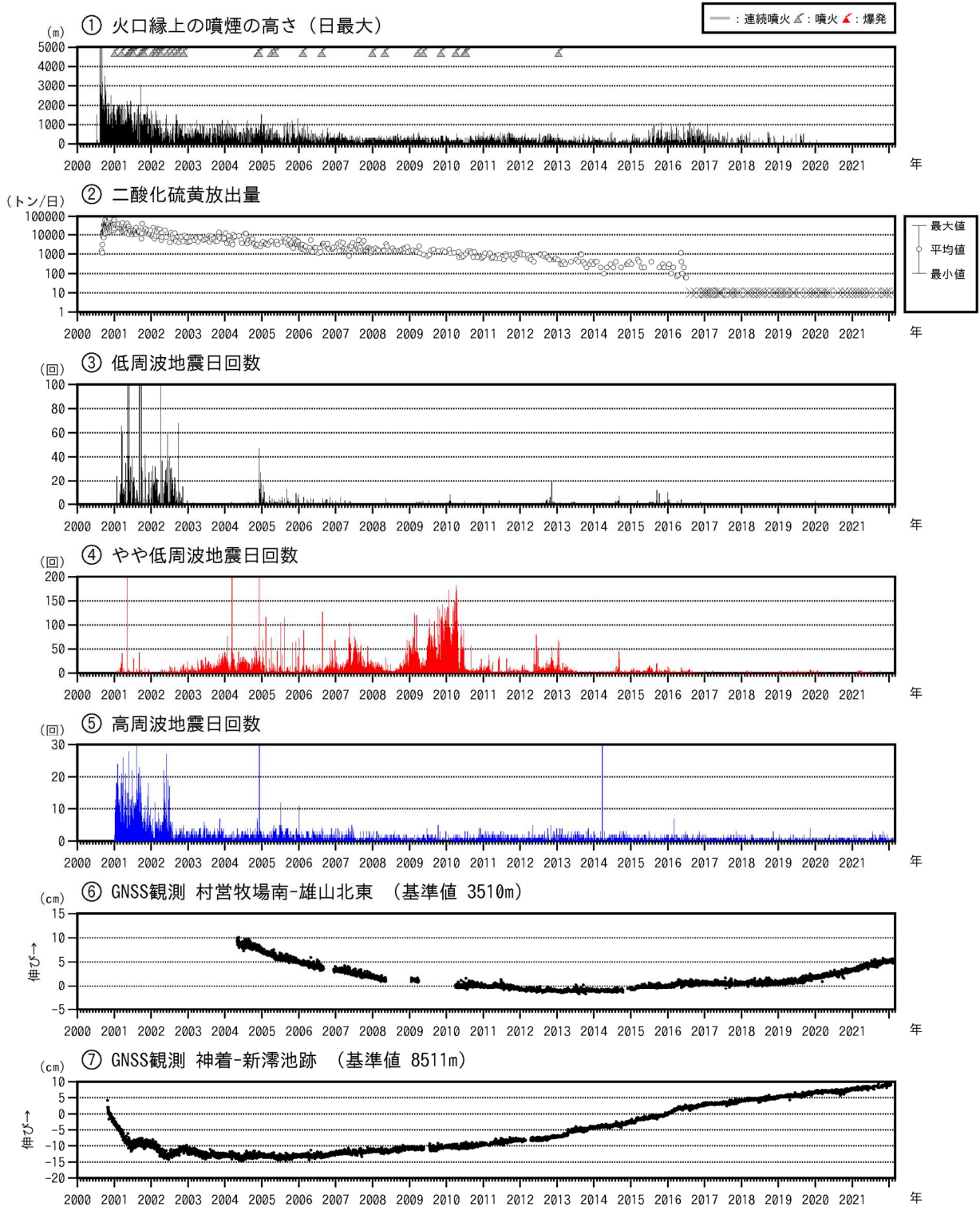
図6 三宅島 長期の火山活動経過図（2000年1月1日～2022年2月28日） ※図6の説明は次ページに掲載。
