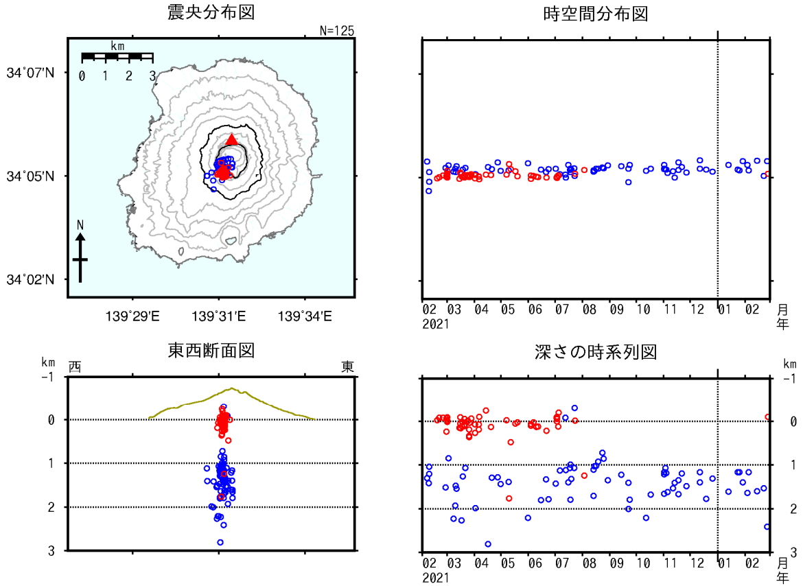
図9 三宅島 震源分布図（2021年2月1日～2022年2月28日）
