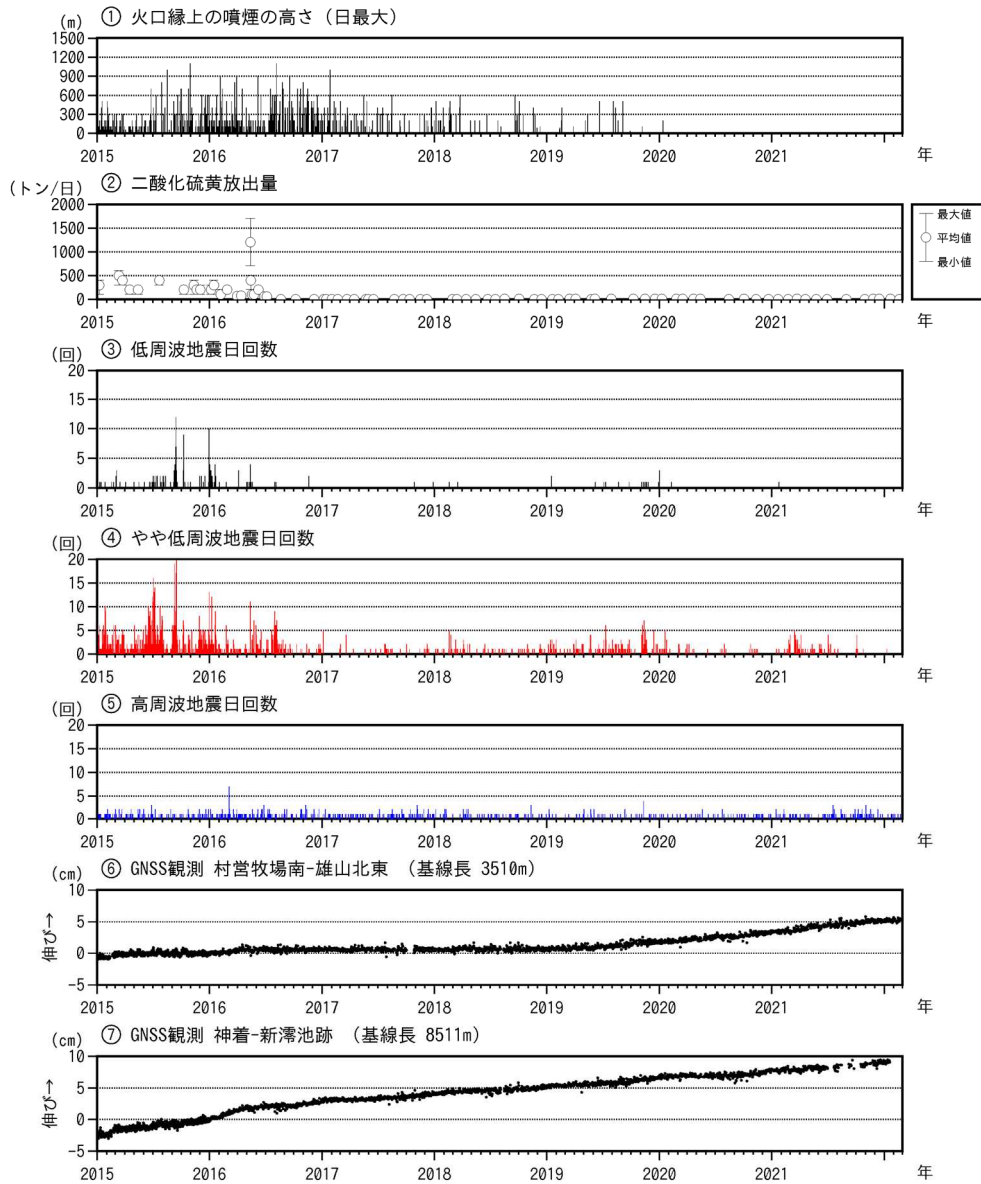
図7 三宅島 短期の火山活動経過図（2015年1月1日～2022年2月28日）
