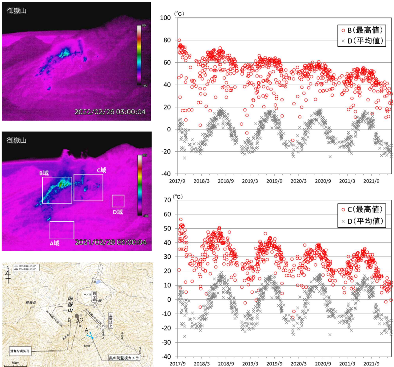
図9 御嶽山 奥の院赤外熱映像カメラによる剣ヶ峰南西側における最高温度の推移 (2017年9月13日～2022年2月28日)
