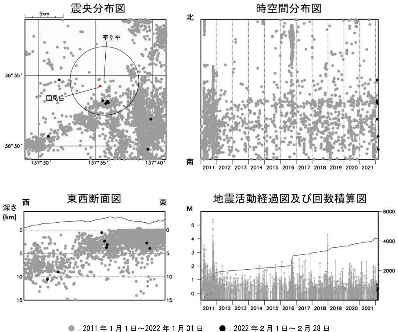
図2 弥陀ヶ原 広域地震観測網による山体・周辺の地震活動（2011 年 1 月 1 日～2022 年 2 月 28 日） 震央分布図中の円は弥陀ヶ原の計数対象地震（室堂平で S-P 時間 1 秒以内）のおよその範囲を示しています。 広域地震観測網により震源決定したもので、深さは全て海面以下として決定しています。 図中の震源要素は一部暫定値が含まれており、後日変更することがあります。 この図では、関係機関の地震波形を一元的に処理し、地震観測点の標高を考慮する等した新手法で得られた震源を用いています（ただし、2020 年 8 月以前の地震については火山活動評価のための参考震源です）。 2022 年 3 月 8 日現在、次の期間の地震について、暫定的に震源精査の基準を変更しているため、その前後の期間と比較して微小な地震での震源決定数の変化（増減）が見られます。 (1) 2020 年 9 月 1 日から 10 月 23 日まで、(2) 2021 年 1 月 9 日から 3 月 7 日まで、 (3) 2021 年 4 月 19 日から 12 月 5 日まで
