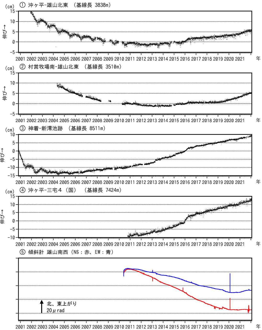
図8 三宅島 GNSS 連続観測及び傾斜計観測結果（2000年10月26日～2022年1月31日）
