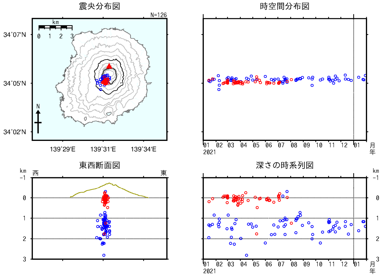
図9 三宅島 震源分布図（2021年1月1日～2022年1月31日）
