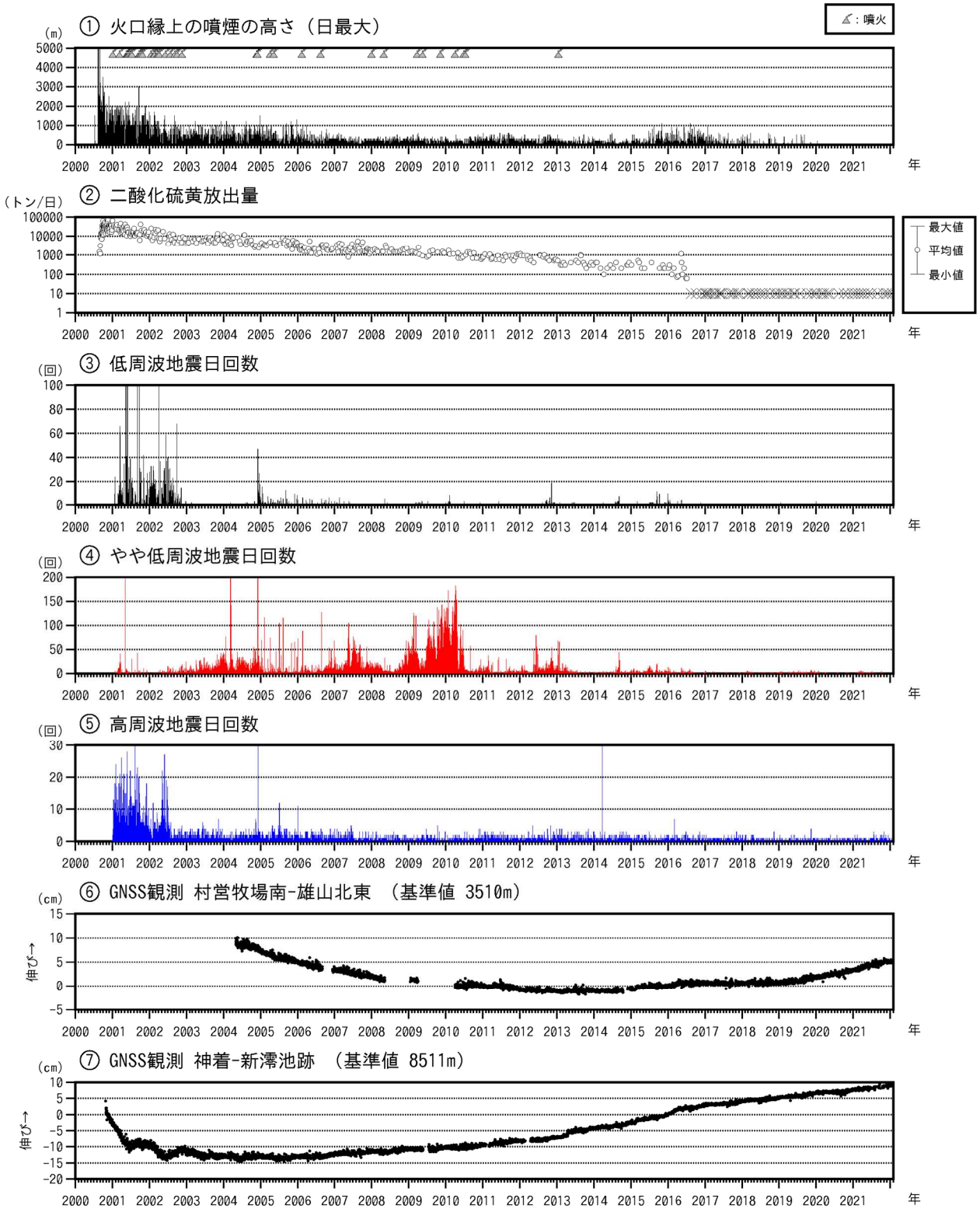
図6 三宅島 火山活動長期経過図（2000年1月1日～2022年1月31日） ※図6の説明は次ページに掲載。
