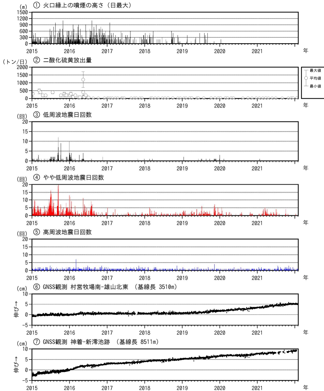
図7 三宅島 火山活動短期経過図（2015年1月1日～2022年1月31日）
