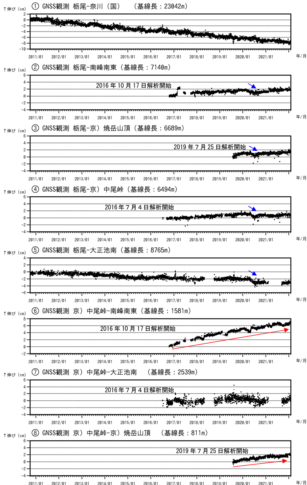
図5 焼岳 GNSS連続観測による基線長変化（2010年10月1日～2022年1月31日）
