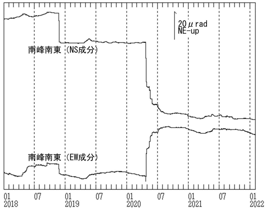
図7 焼岳 南峰南東観測点における傾斜データ（2018年1月1日～2022年1月31日）
