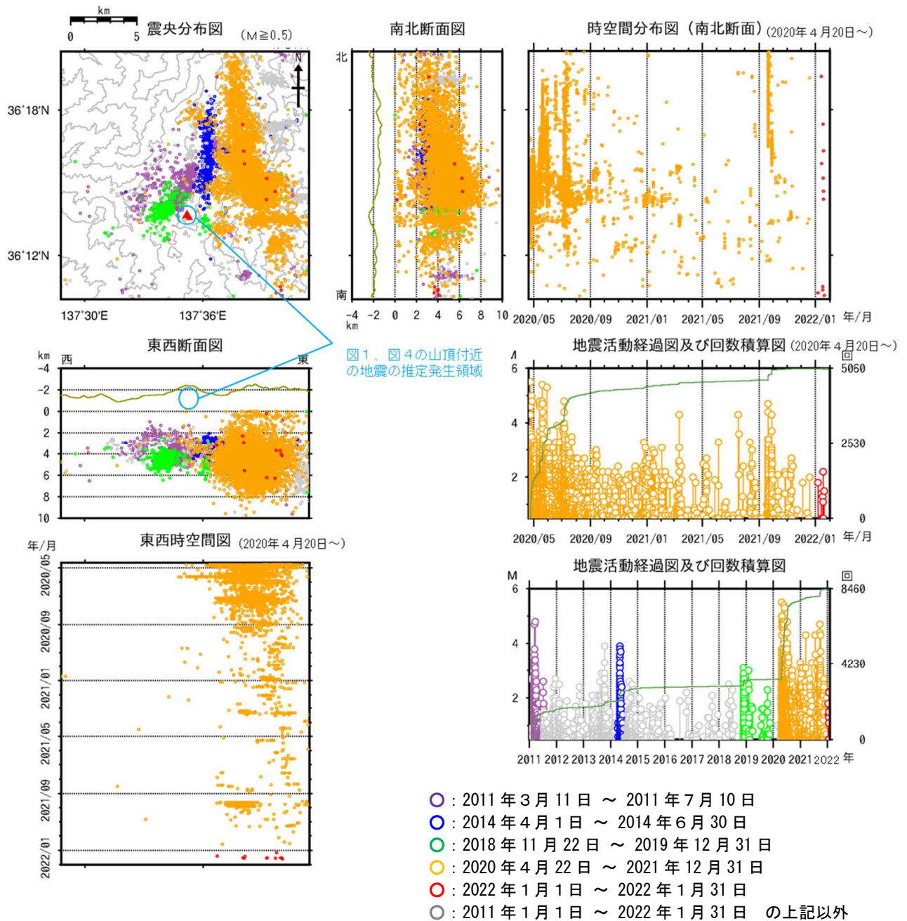
図8 焼岳 広域地震観測網による山体及び周辺の地震活動(2011年1月1日～2022年1月31日)
