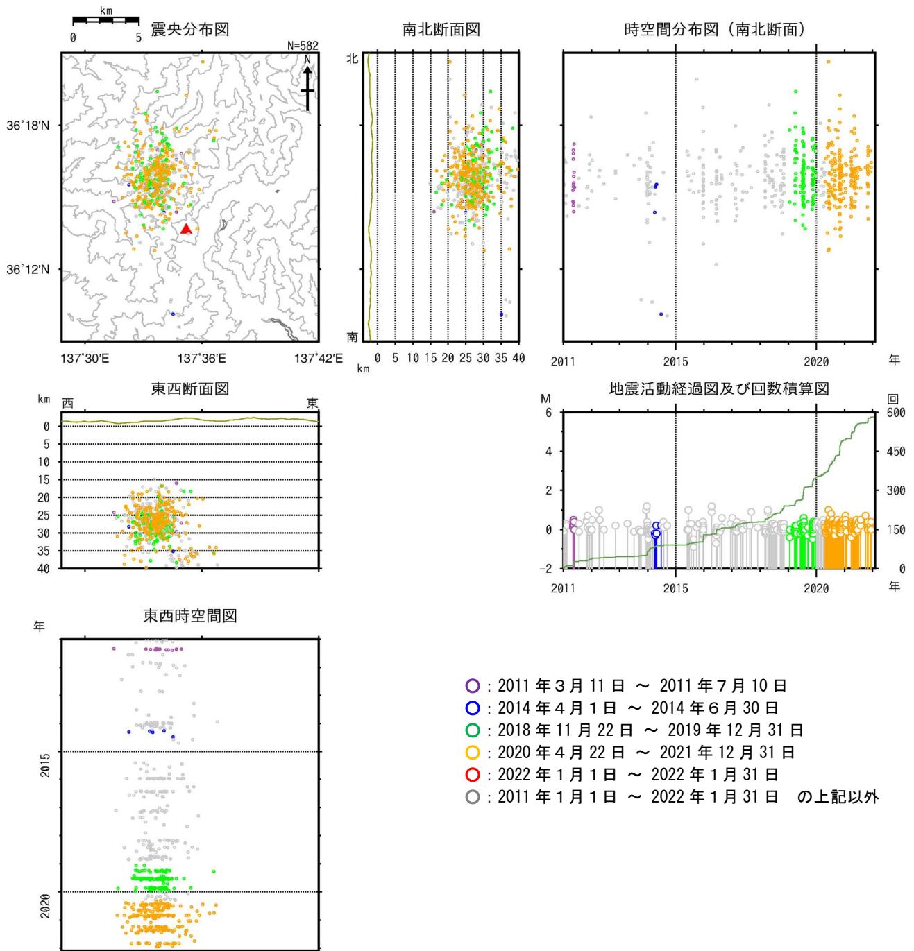
図9 焼岳 広域地震観測網による深部低周波地震の震源分布図（2011年1月1日～2022年1月31日） 広域地震観測網により震源決定したもので、深さは全て海面以下として決定しています。そのため、山頂付近の浅い地震の震源も海面下に決定されています。
