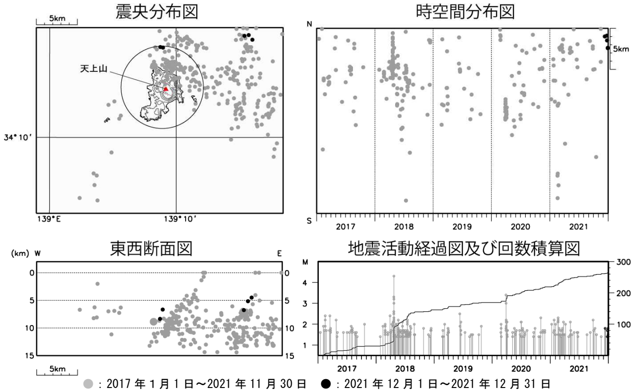
図3 神津島 広域地震観測網による山体・周辺の地震活動（2017年1月1日～2021年12月31日）
