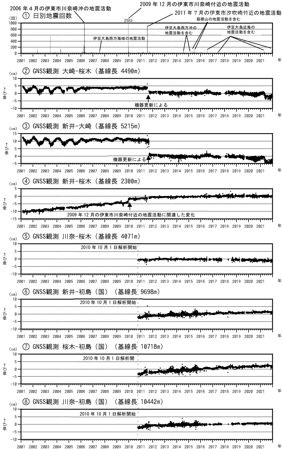
図3 伊豆東部火山群 火山活動経過図（2001年1月1日～2021年12月31日）
