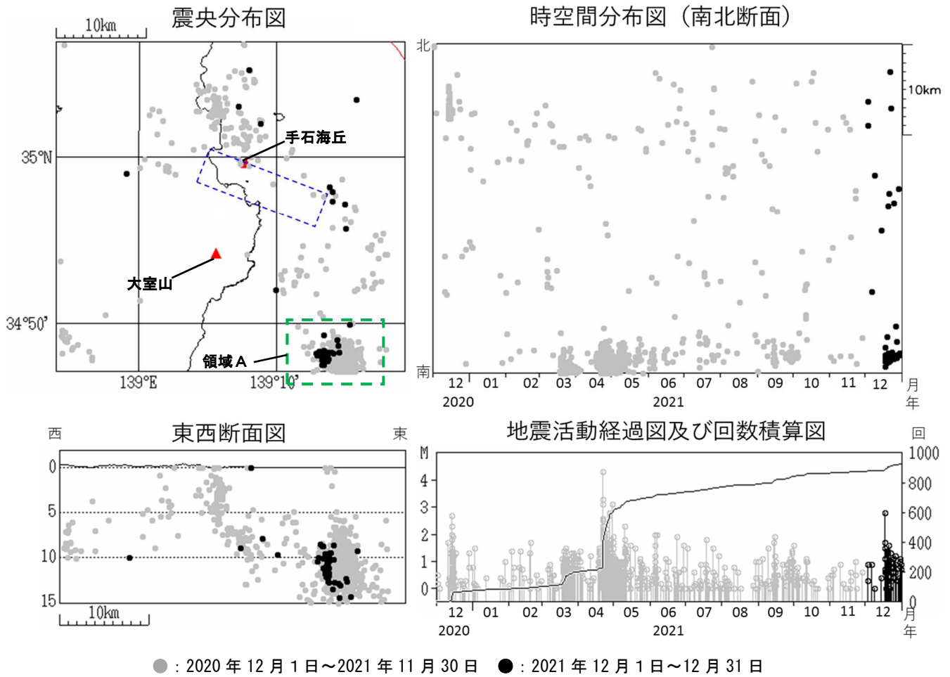
図2 伊豆東部火山群 広域地震観測網による震源分布図（2020年12月1日～2021年12月31日） □の領域は群発地震活動の発生する可能性がある範囲（火口が発生する可能性のある範囲）を示しています。 https://www.data.jma.go.jp/vois/data/tokyo/STOCK/level/PDF/level_316.pdf 広域地震観測網により震源決定したもので、深さは全て海面以下として決定しています。 M（マグニチュード）は地震の規模を表し、M0.0以上を表示しています。 図中の震源要素は一部暫定値が含まれており、後日変更することがあります。 この図では、関係機関の地震波形を一元的に処理し、地震観測点の標高を考慮する等した新手法で得られた震源を用いています。 2022年1月12日現在、次の期間の地震について、暫定的に震源精査の基準を変更しているため、その前後の期間と比較して微小な地震での震源決定数の変化（増減）が見られます。 ① 2021年1月9日から3月7日まで、② 2021年4月19日から12月5日まで
