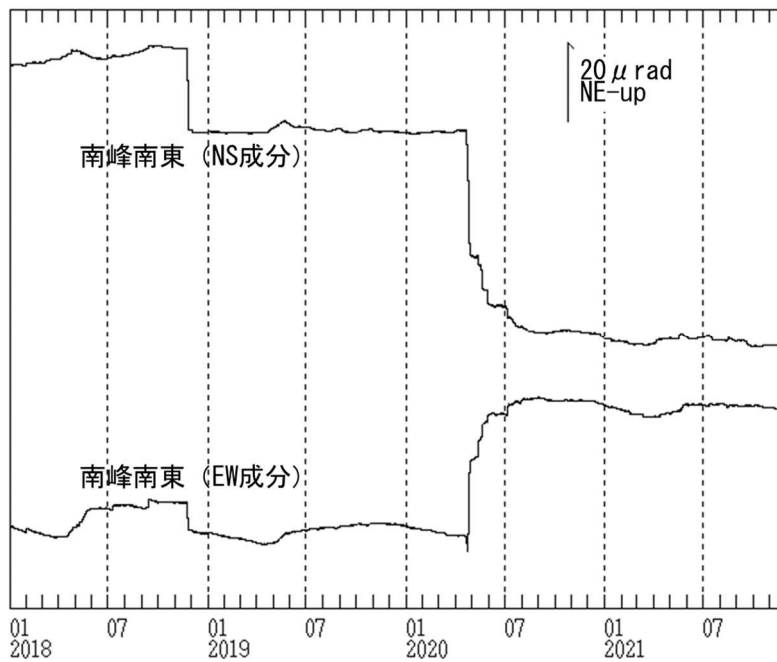
図7 焼岳 南峰南東観測点における傾斜データ（2018年1月1日～2021年11月30日）
