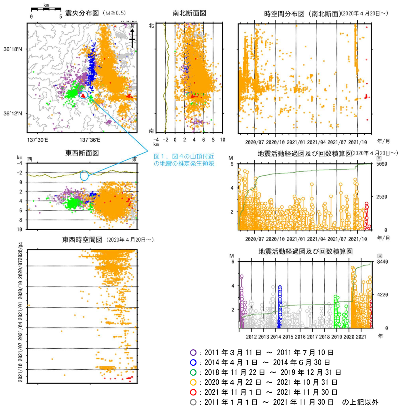
図8 焼岳 広域地震観測網による山体及び周辺の地震活動(2011年1月1日～2021年11月30日)
