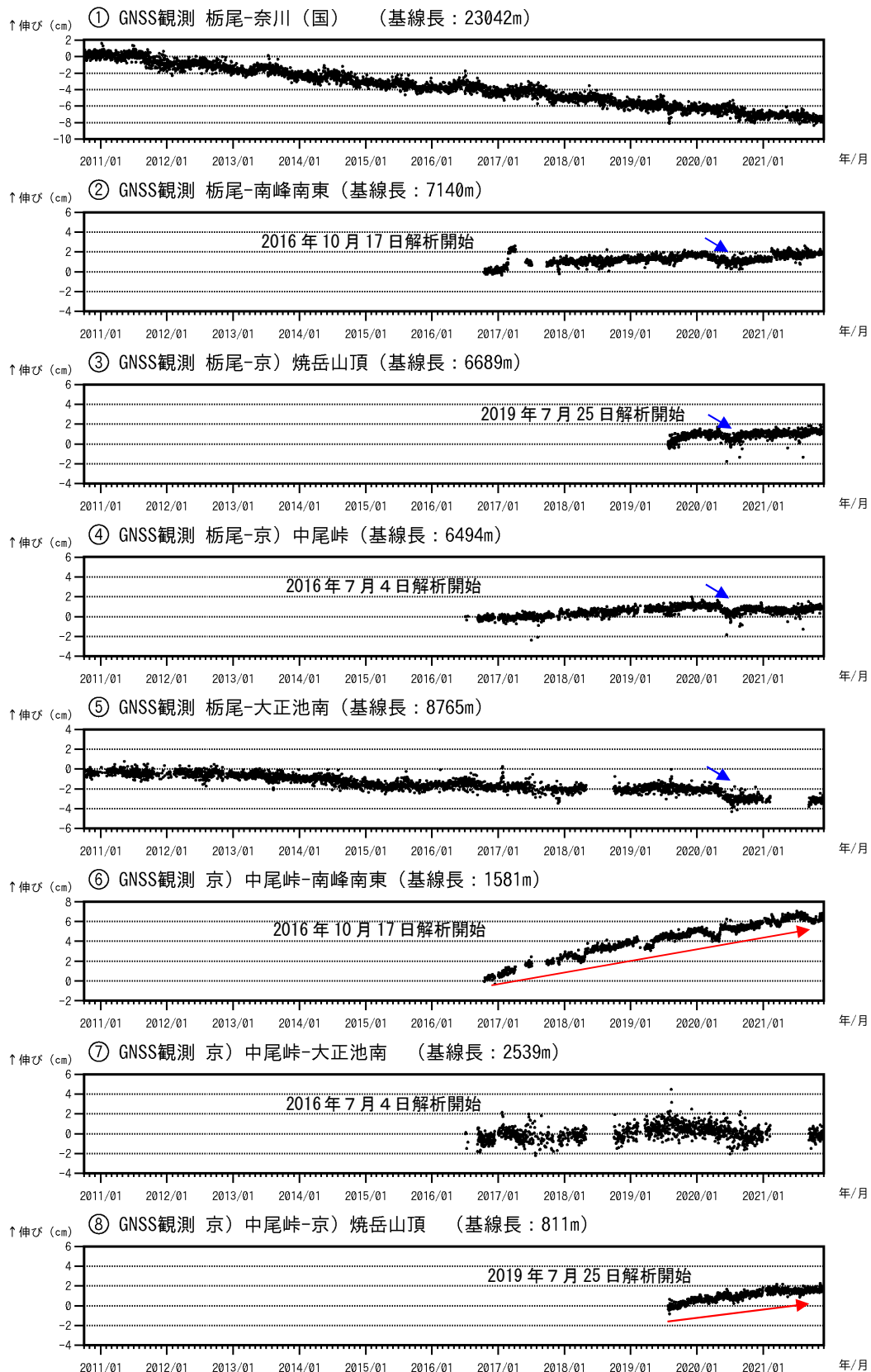
図5 焼岳 GNSS連続観測による基線長変化（2010年10月1日～2021年11月30日）
