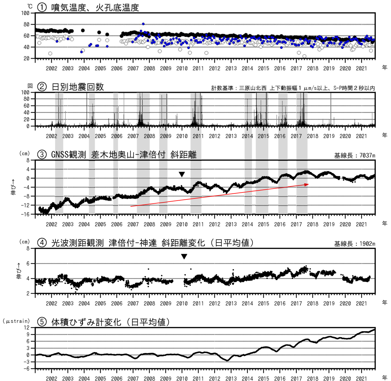
図2 伊豆大島 最近の火山活動経過図（2001年1月～2021年10月31日）
