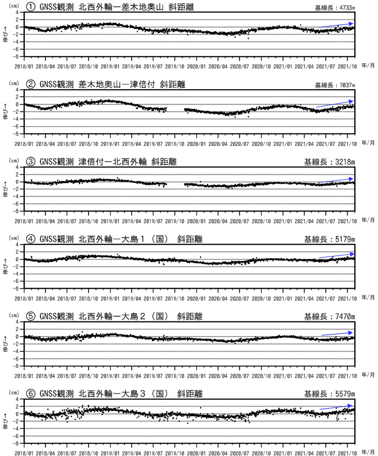
図3-2 伊豆大島 GNSS連続観測による基線長変化(2018年1月~2021年10月31日)
