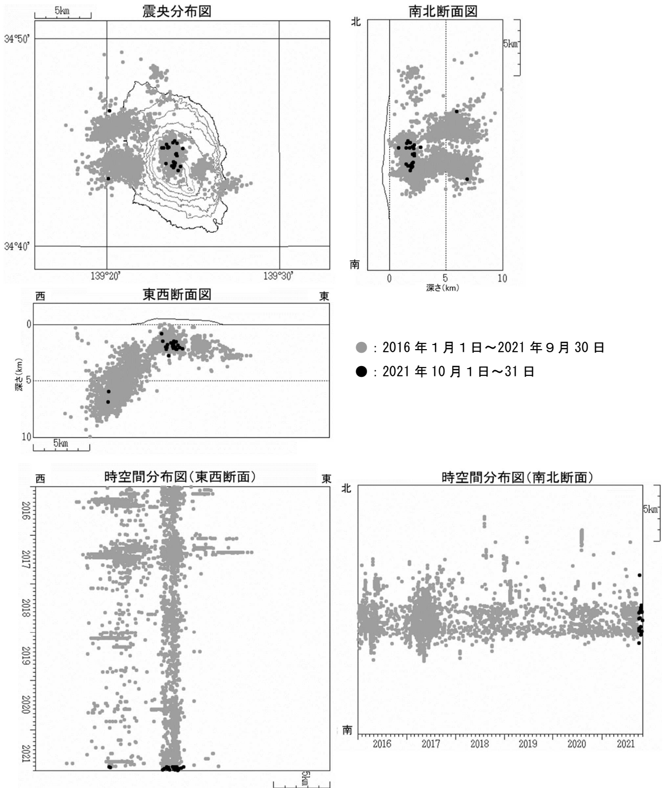
図4 伊豆大島 震源分布図（2016年1月1日～2021年10月31日）
