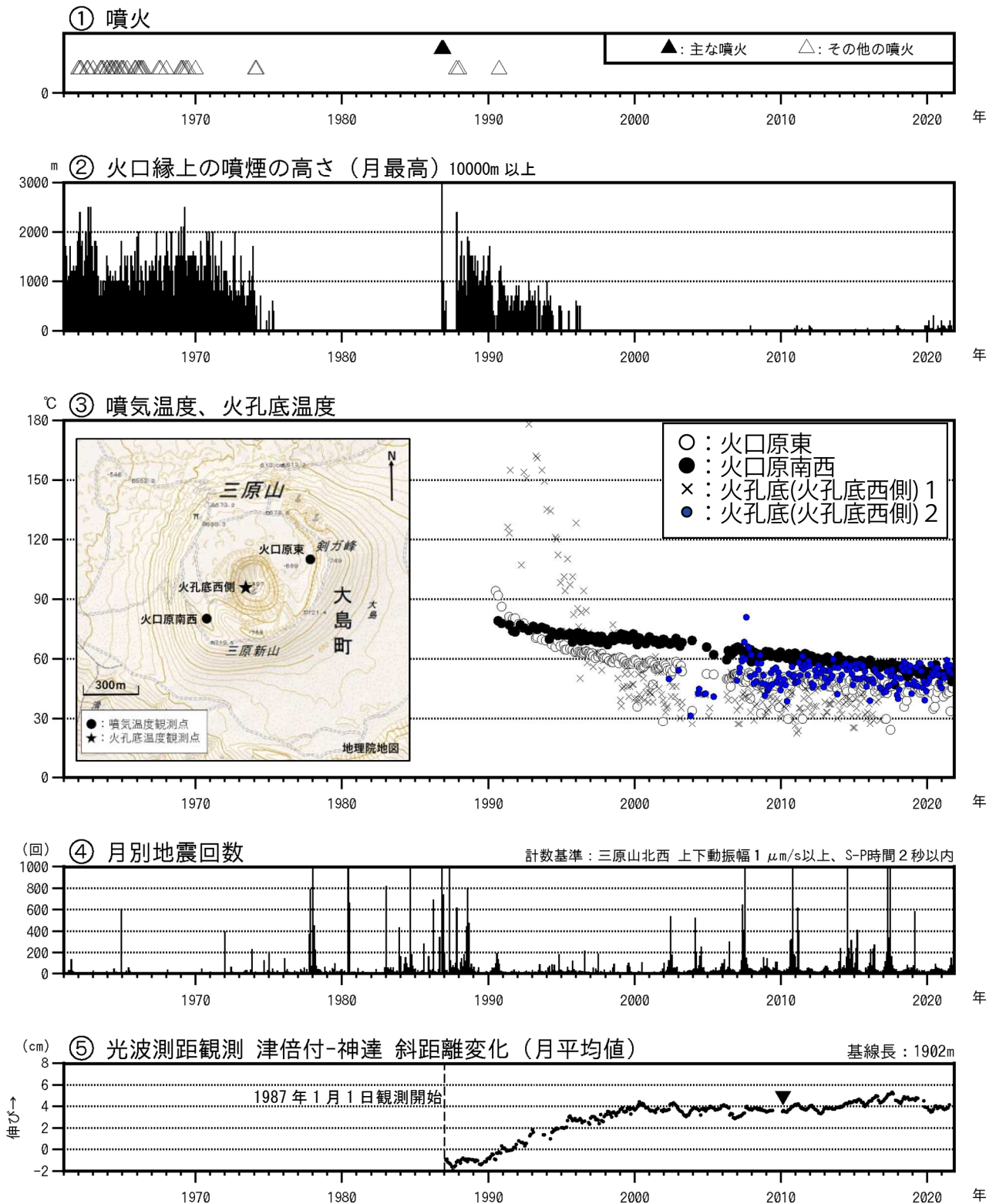
図1 伊豆大島 長期間の火山活動経過図（1961年1月～2021年10月31日）
