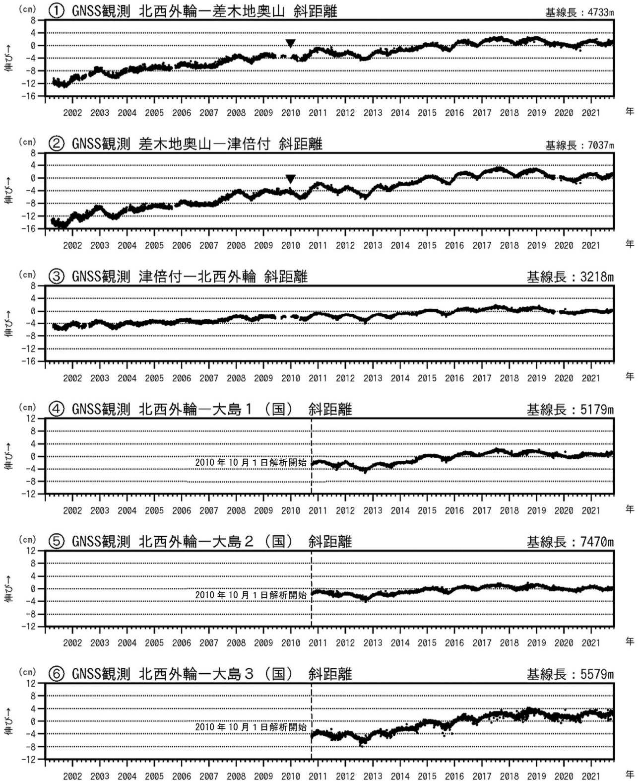
図3-1 伊豆大島 GNSS連続観測による基線長変化(2001年1月～2021年10月31日)
