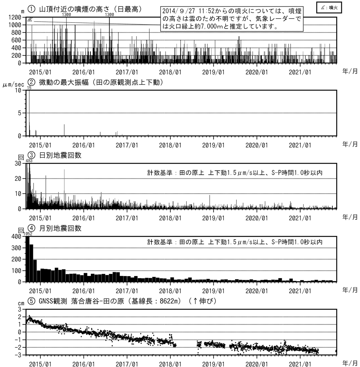
図4 御嶽山 最近の火山活動経過図（2014年9月1日～2021年10月31日）
