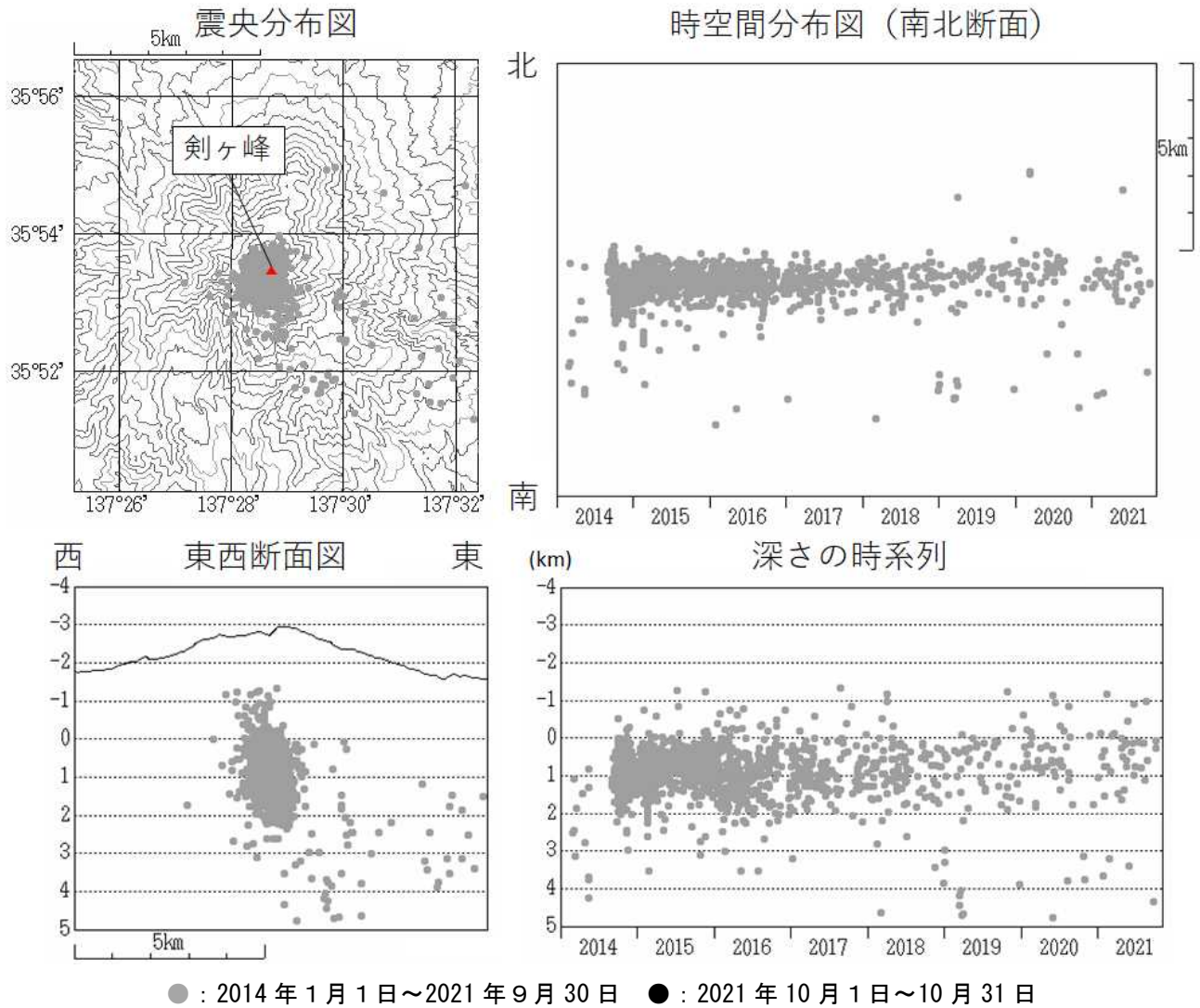
図3 御嶽山 震源分布図（2014 年 1 月 1 日～2021 年 10 月 31 日）
