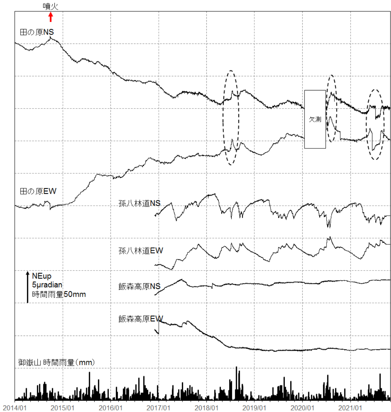
図7 御嶽山 傾斜変動（2014年1月1日～2021年10月31日）
