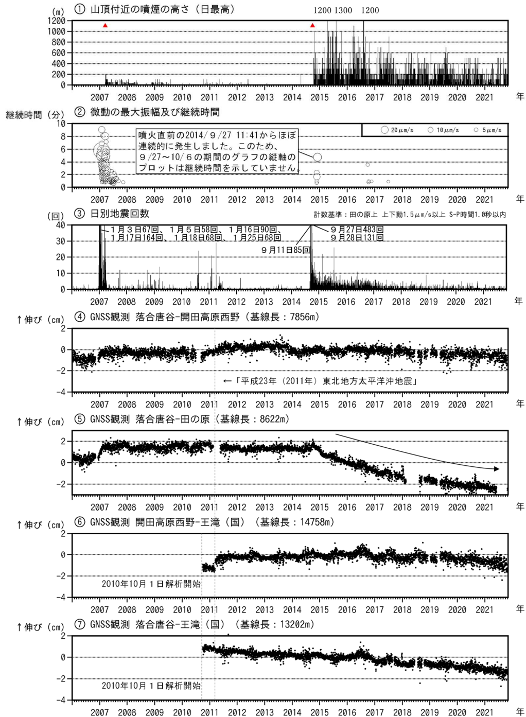
図5 御嶽山 長期間の火山活動経過図（2006年1月1日～2021年10月31日）
