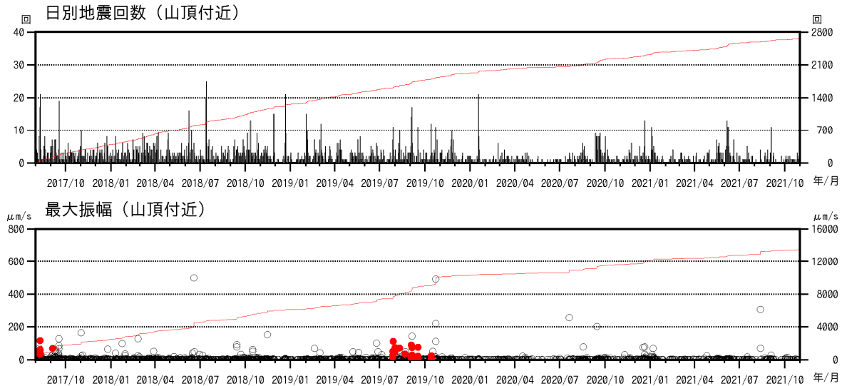
図1 焼岳 山頂付近の地震回数、及び南峰南東観測点上下動最大振幅
