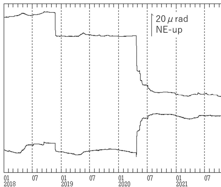
図7 焼岳 南峰南東観測点における傾斜データ（2018年1月1日～2021年10月31日）
