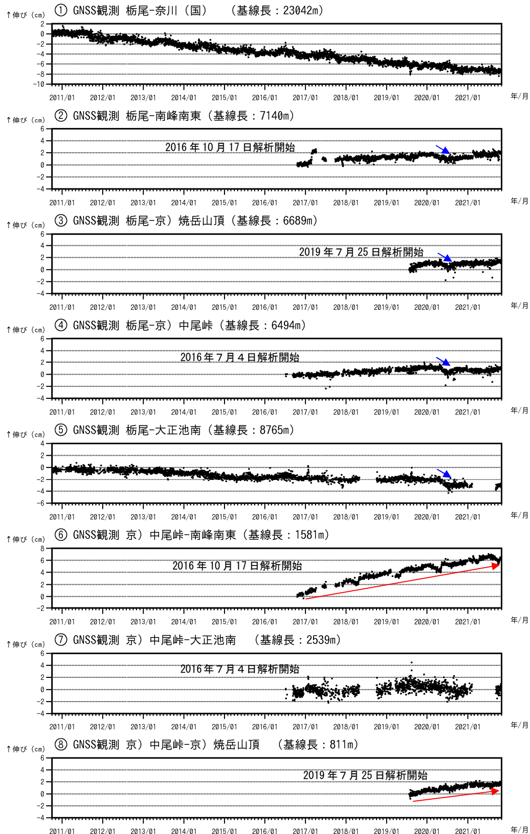
図5 焼岳 GNSS連続観測による基線長変化（2010年10月1日～2021年10月31日）
