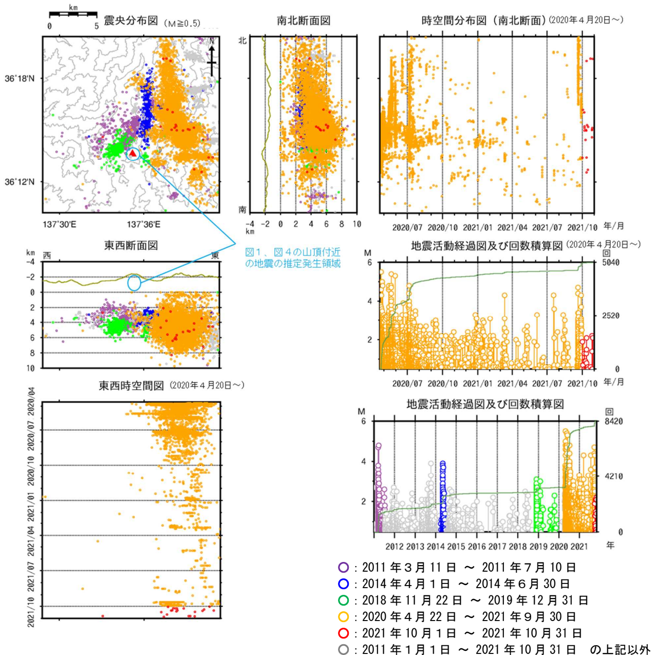
図8 焼岳 広域地震観測網による山体及び周辺の地震活動(2011年1月1日～2021年10月31日)
