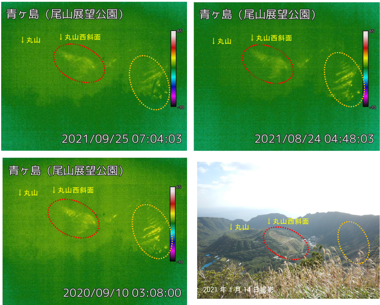
図2 青ヶ島 カルデラ内の地表面温度の状況（左上, 右上, 左下：尾山展望公園監視カメラによる、右下：2021年1月14日に撮影した同場所からの写真）
