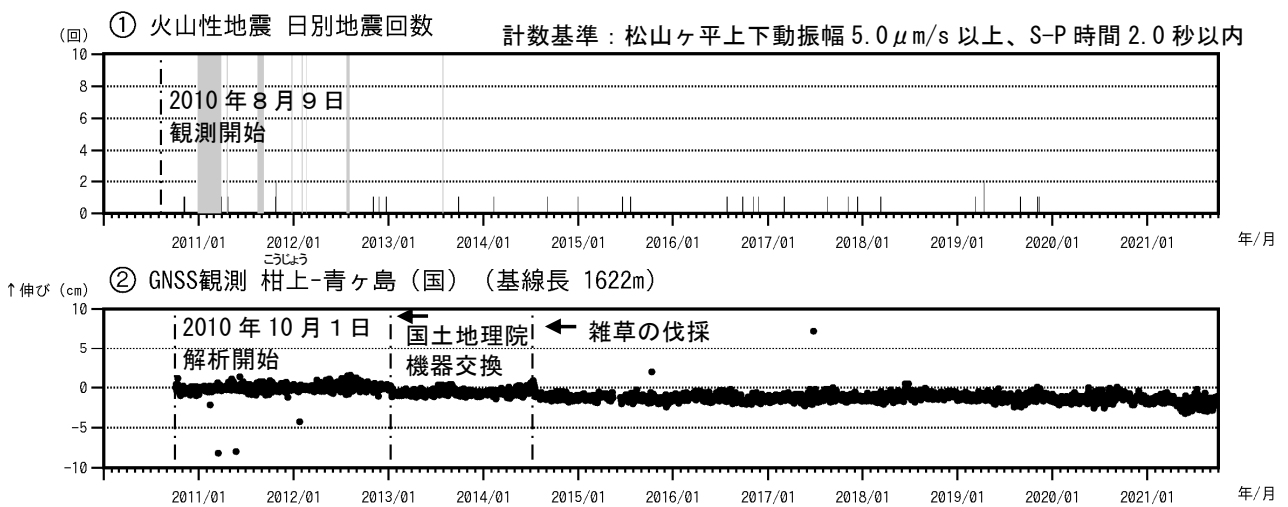
図3 青ヶ島 火山活動経過図（2010年8月9日～2021年9月30日）
