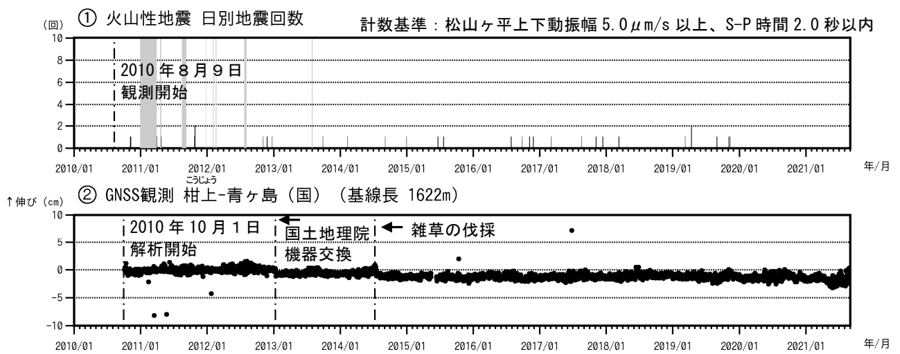
図3 青ヶ島 火山活動経過図（2010年8月9日～2021年8月31日）
