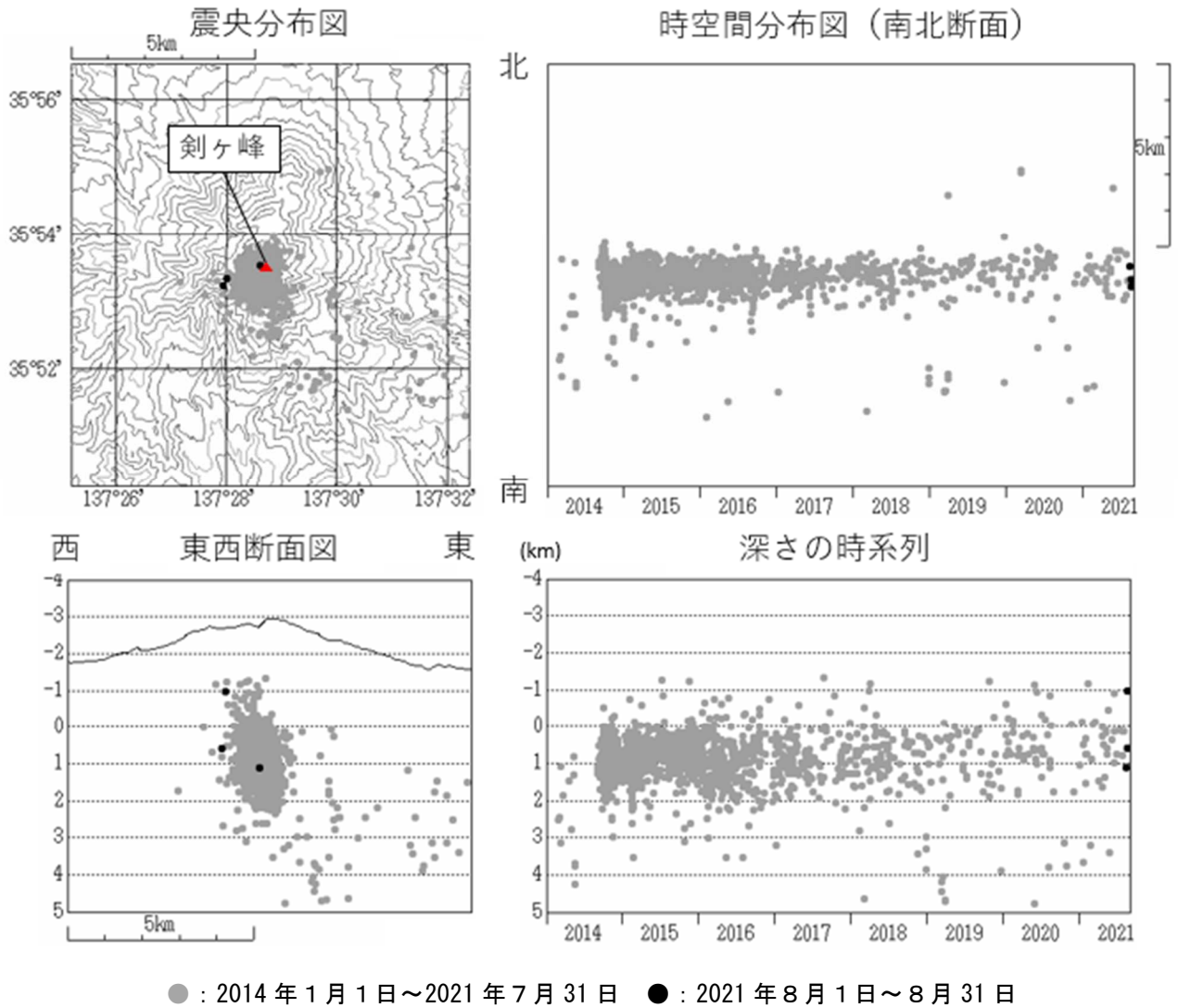
図3 御嶽山 震源分布図（2014 年 1 月 1 日～2021 年 8 月 31 日）
