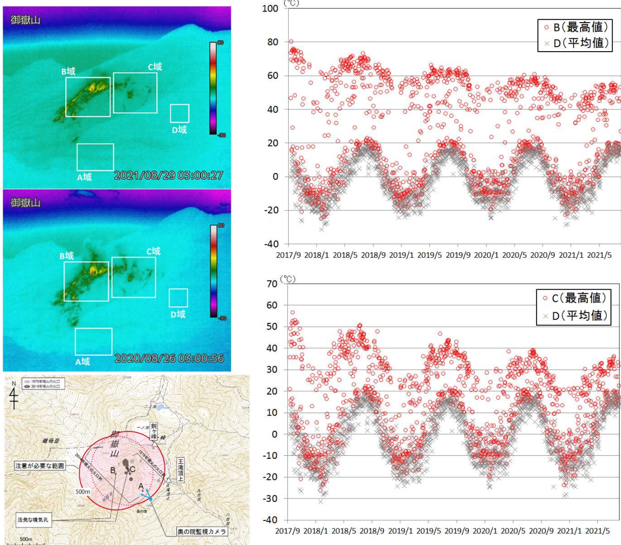
図2 御嶽山 奥の院赤外熱映像カメラによる剣ヶ峰南西側における最高温度の推移
