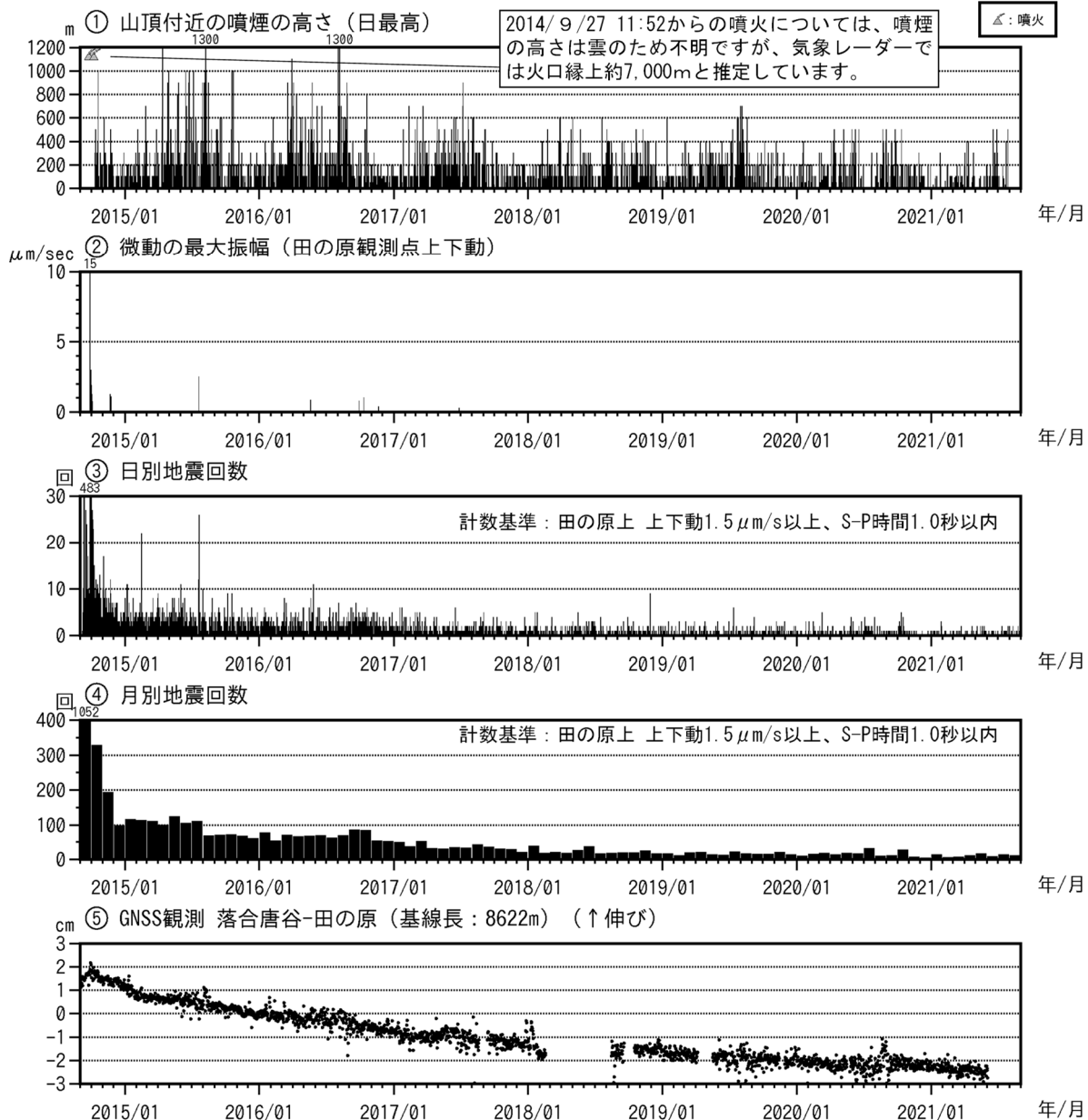
図4 御嶽山 最近の火山活動経過図（2014年9月1日～2021年8月31日）
