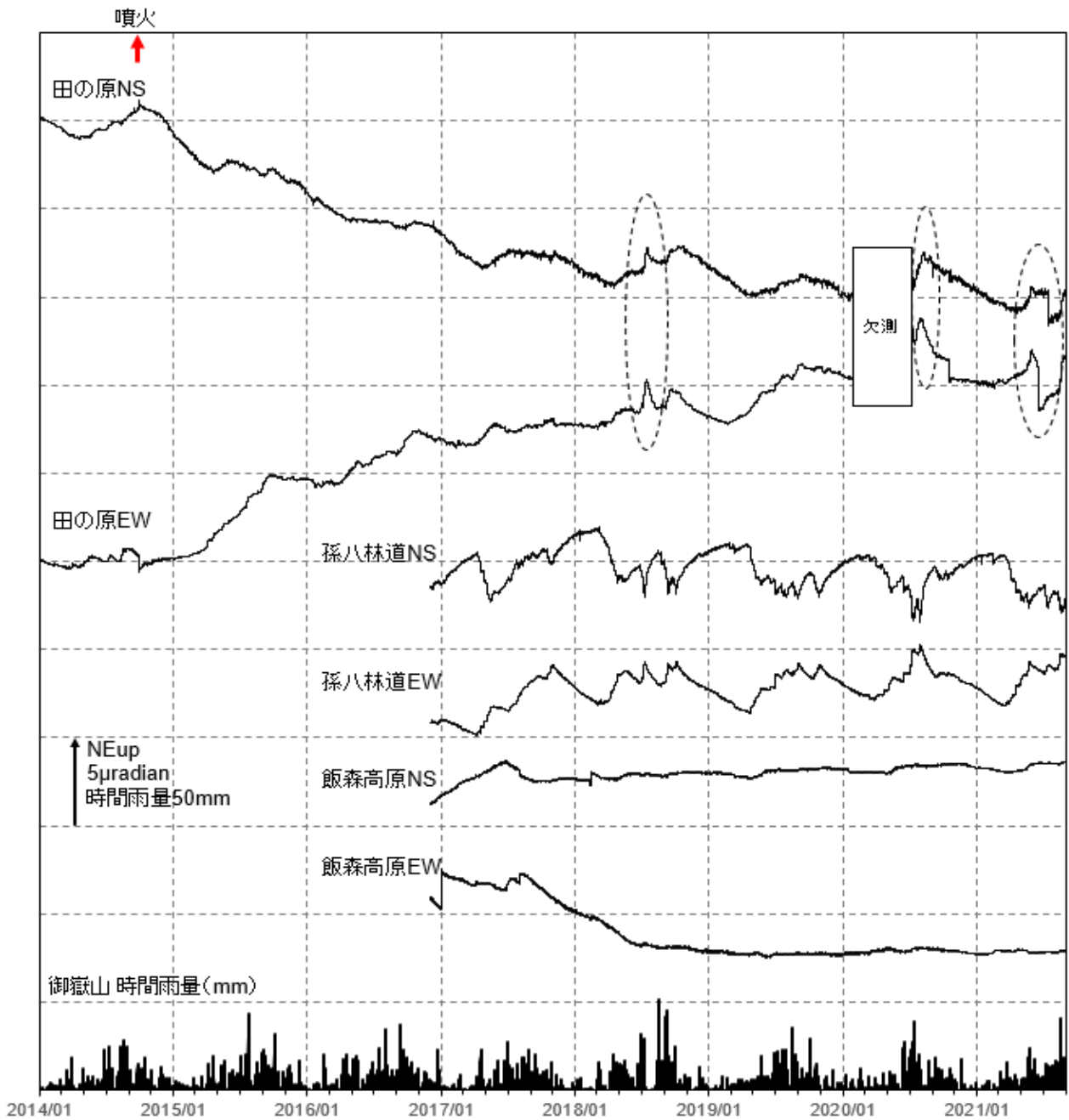
図7 御嶽山 傾斜変動（2014年1月1日～2021年8月31日）
