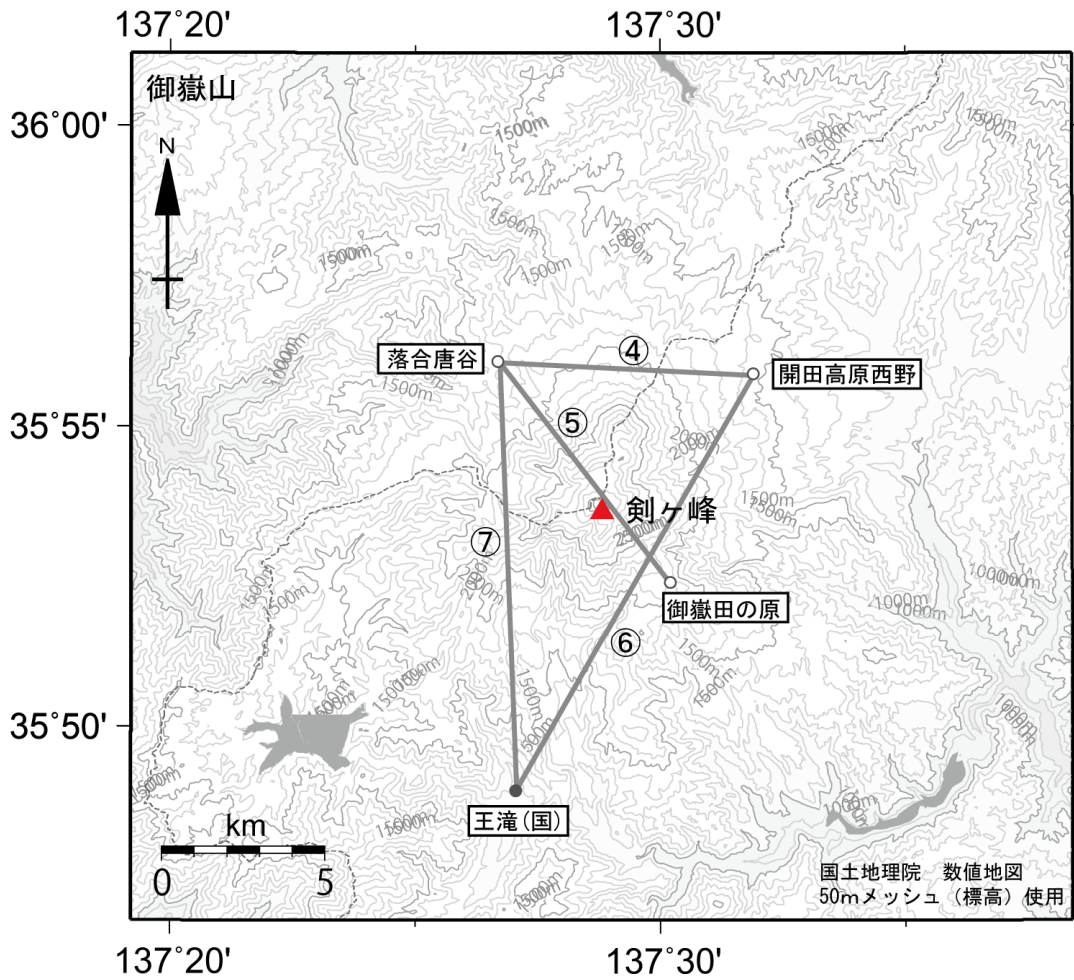
図6 御嶽山 GNSS 連続観測点と基線番号
