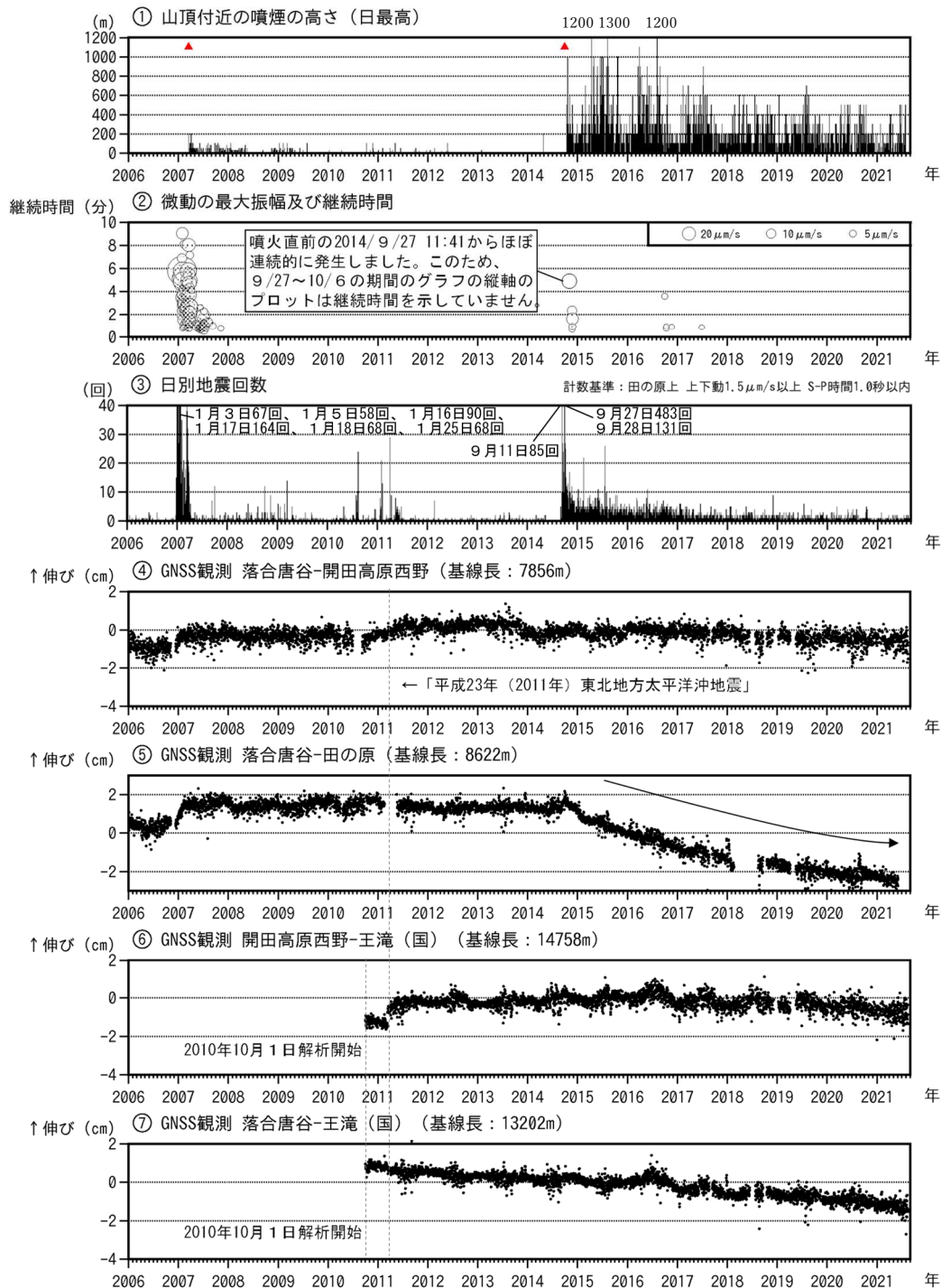
図5 御嶽山 長期間の火山活動経過図（2006年1月1日～2021年8月31日）
