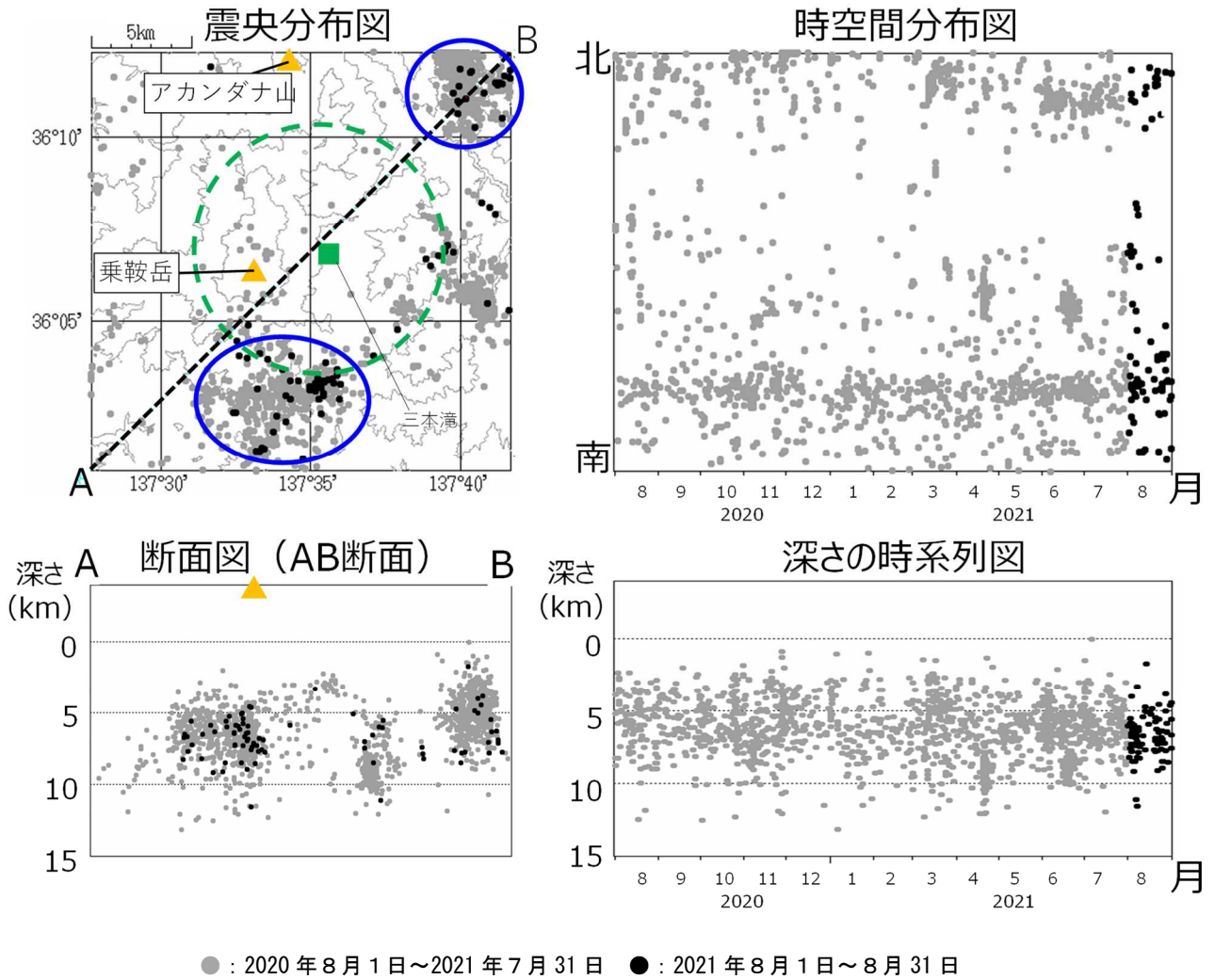
図3 乗鞍岳 広域地震観測網による山体・周辺の地震活動(2020年8月1日～2021年8月31日) 広域地震観測網により震源決定したもので、深さは全て海面以下として決定しています。図中の震源要素は一部暫定値が含まれており、後日変更することがあります。 この図では、関係機関の地震波形を一元的に処理し、地震観測点の標高を考慮する等した新手法で得られた震源を用いています（ただし、2020年8月以前の地震については火山活動評価のための参考震源です）。 2021年9月8日現在、次の期間の地震について、暫定的に震源精査の基準を変更しているため、その前後の期間と比較して微小な地震での震源決定数の変化（増減）が見られます。 (1)2020年4月18日から10月23日まで、(2)2021年1月9日から3月7日まで、(3)2021年4月19日以降 震央分布図中の緑点線円は、図2①で計数される地震のおおよその範囲を示します。
