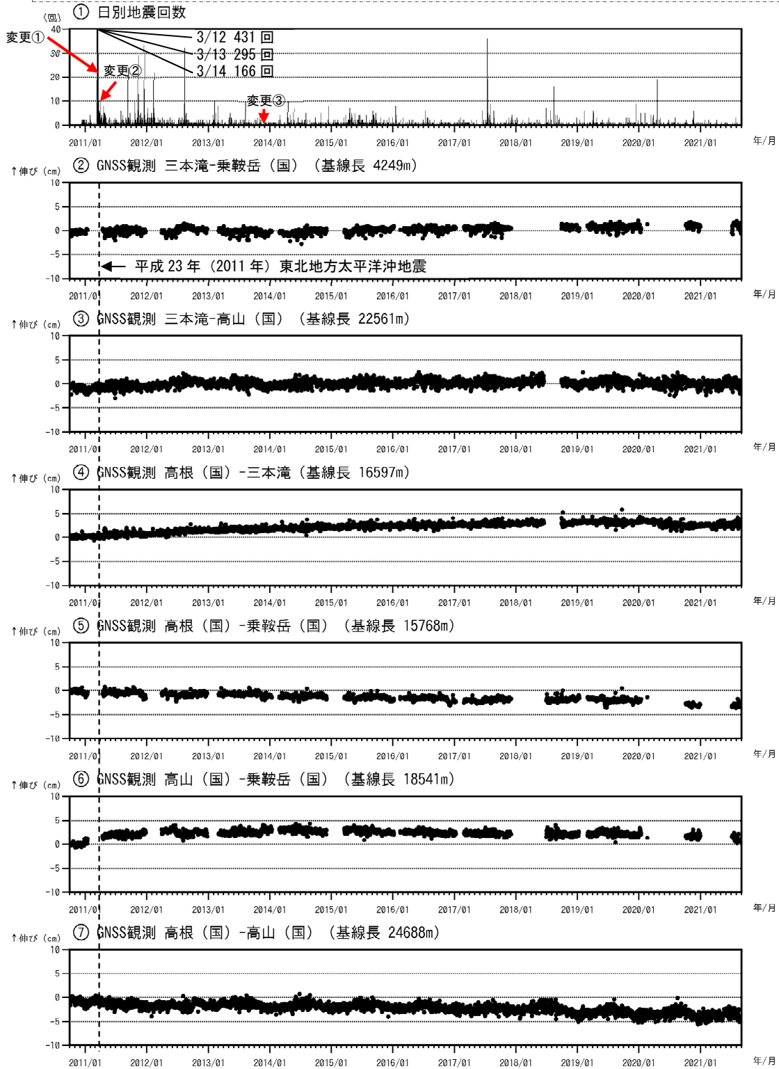
図2 乗鞍岳 火山活動経過図（2010年10月1日～2021年8月31日）
