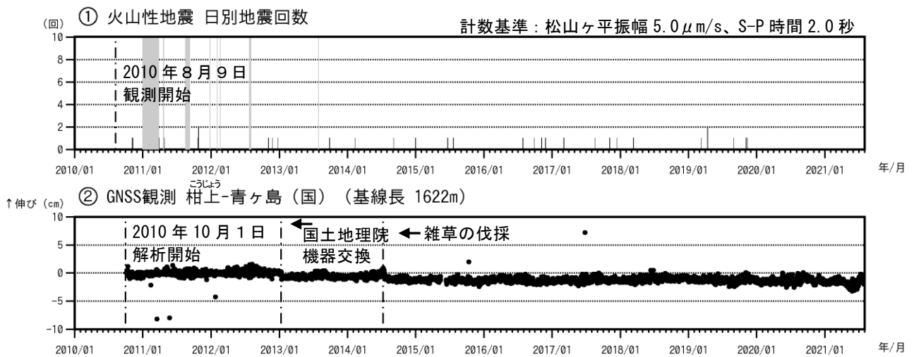
図3 青ヶ島 火山活動経過図（2010年8月9日～2021年7月31日） ① グラフの灰色部分は機器障害による欠測を示す。 ② (国)：国土地理院、図4のGNSS基線②に対応。グラフの空白部分は欠測を示す。
