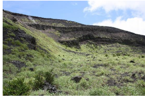
剣ガ峰付近（7月20日撮影）
