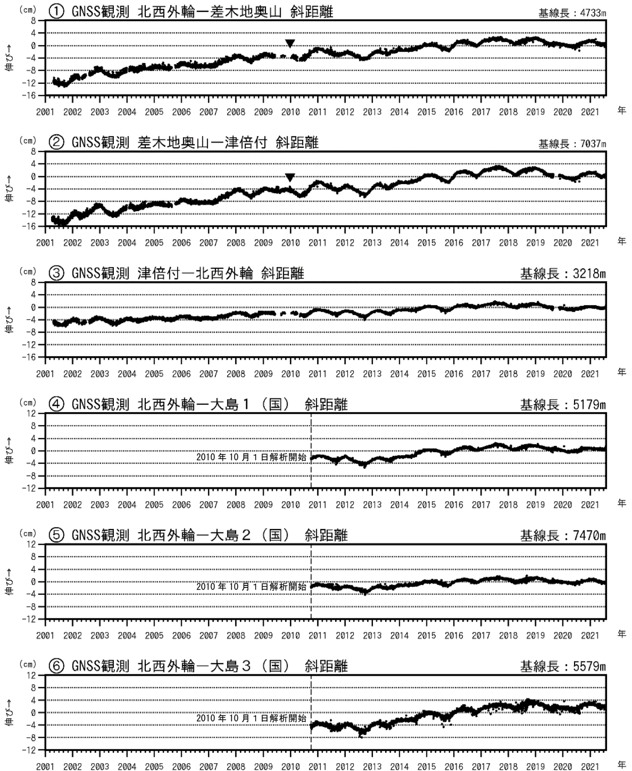
図3-1 伊豆大島 GNSS 連続観測による基線長変化(2001年1月～2021年7月31日)
