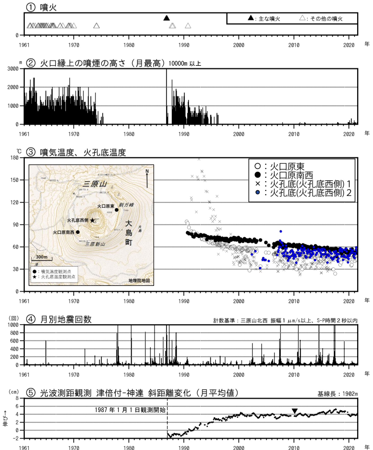
図1 伊豆大島 長期間の火山活動経過図（1961年1月～2021年7月31日）
