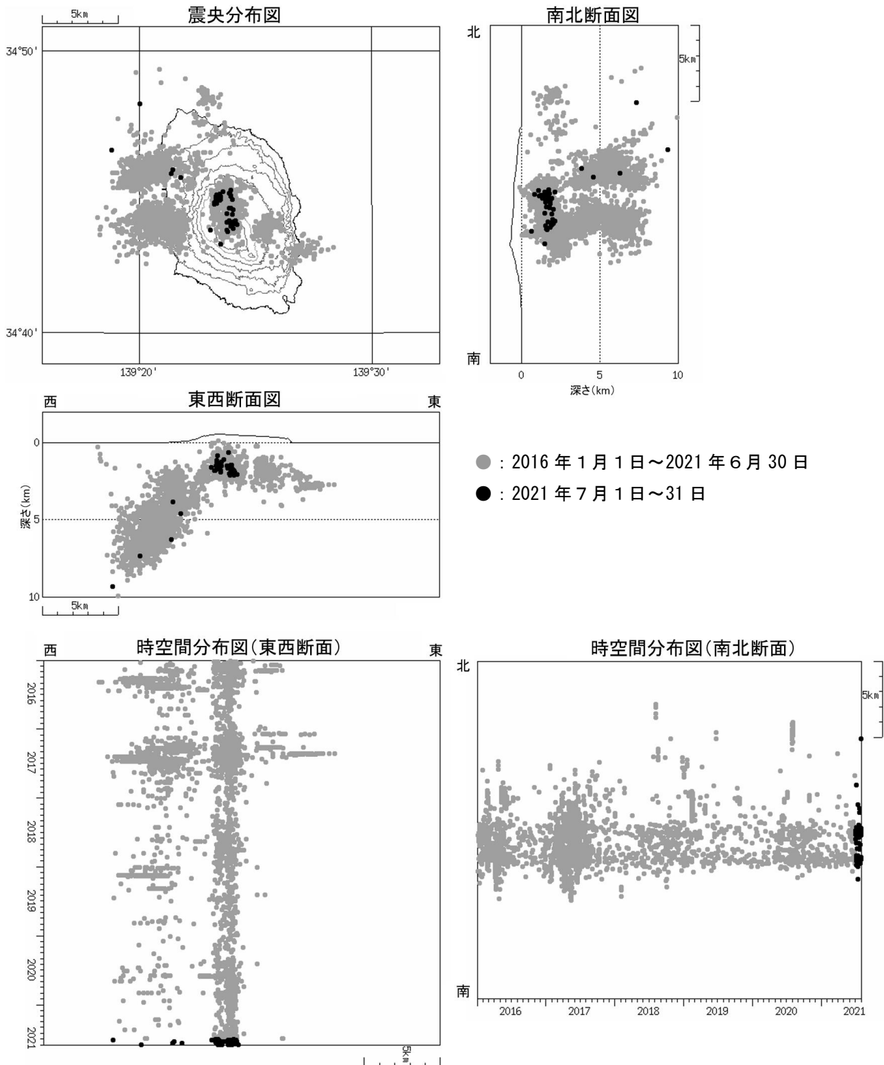
図4 伊豆大島 震源分布図（2016 年 1 月 1 日～2021 年 7 月 31 日）
