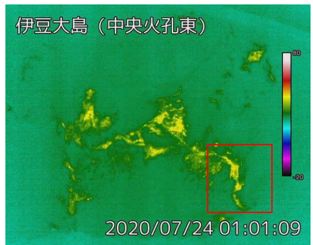
2020年7月24日 中央火孔東監視カメラによる
