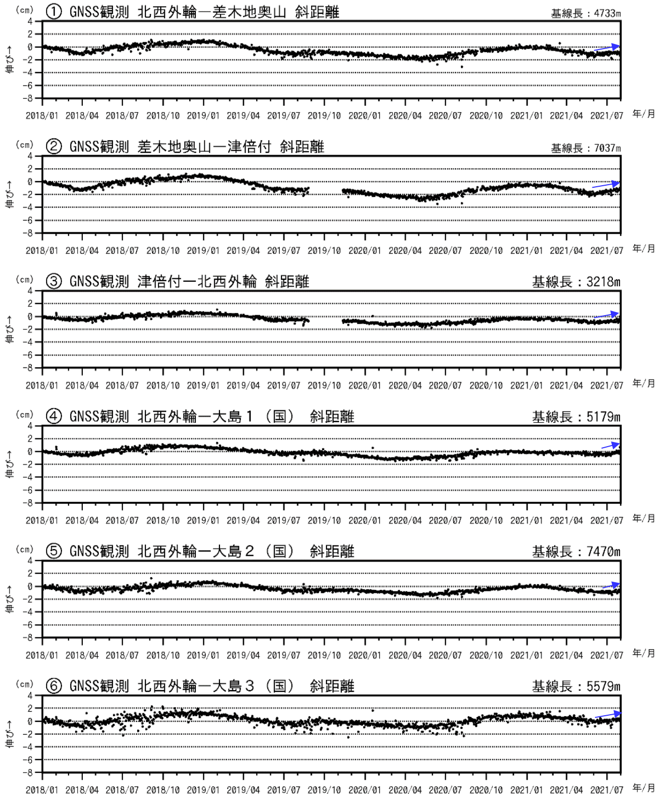
図3-2 伊豆大島 GNSS 連続観測による基線長変化(2018年1月～2021年7月31日)
