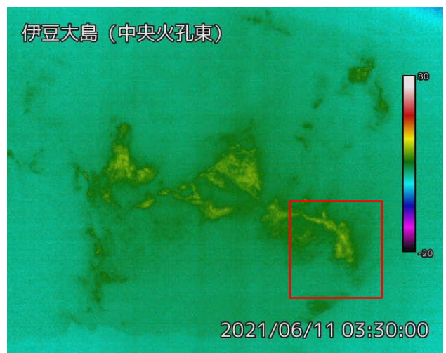
6月11日 中央火孔東監視カメラによる
