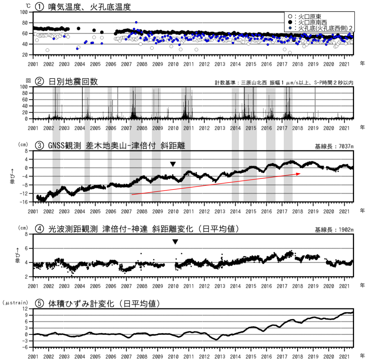
図2 伊豆大島 最近の火山活動経過図（2001年1月～2021年7月31日）
