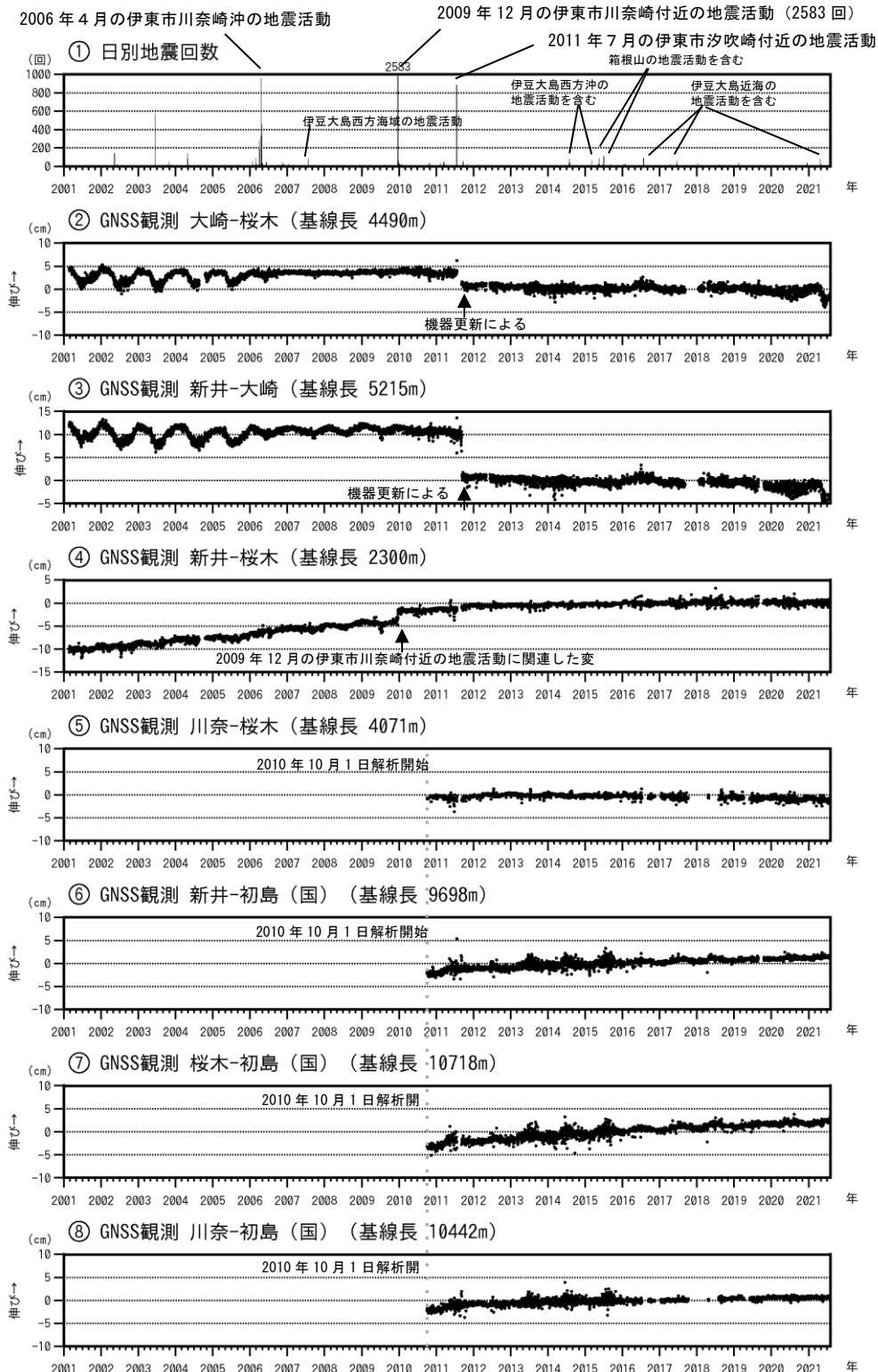
図3 伊豆東部火山群 火山活動経過図（2001年1月1日～2021年7月31日）
