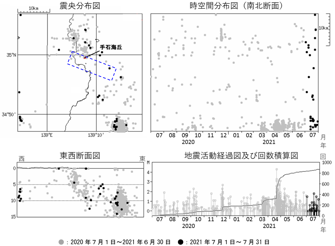
図2 伊豆東部火山群 広域地震観測網による震源分布図（2020年7月1日～2021年7月31日） □の領域は群発地震活動の発生する可能性がある範囲（火口が発生する可能性のある範囲）を示しています。 https://www.data.jma.go.jp/svd/vois/data/tokyo/STOCK/level/PDF/level_316.pdf 広域地震観測網により震源決定したもので、深さは全て海面以下として決定しています。 M（マグニチュード）は地震の規模を表し、M0.0以上を表示しています。 図中の震源要素は一部暫定値が含まれており、後日変更することがあります。 この図では、関係機関の地震波形を一元的に処理し、地震観測点の標高を考慮する等した新手法で得られた震源を用いています（ただし、2020年8月以前の地震については火山活動評価のための参考震源です）。 2021年8月10日現在、次の期間の地震について、暫定的に震源精査の基準を変更しているため、その前後の期間と比較して微小な地震での震源決定数の変化（増減）が見られます。 (1)2020年4月18日から10月23日まで、(2)2021年1月9日から3月7日まで、(3)2021年4月19日以降
